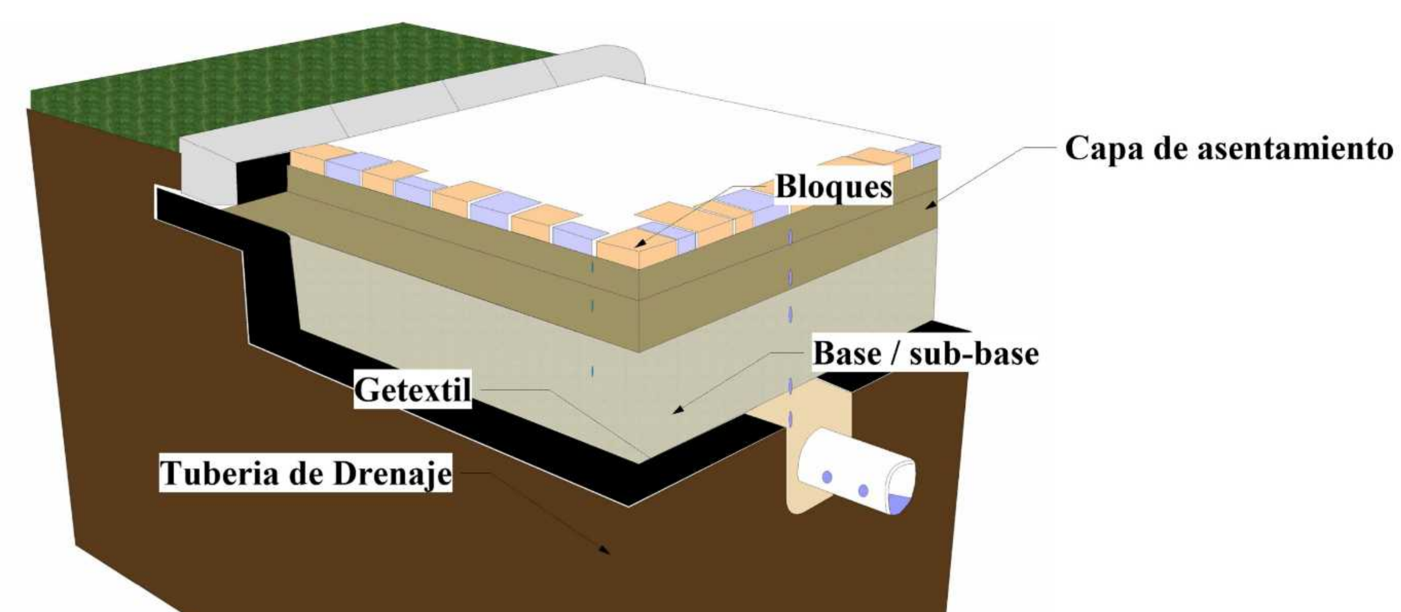
DETALLE DE DRENAJE SOSTENIBLE (SUDS)
