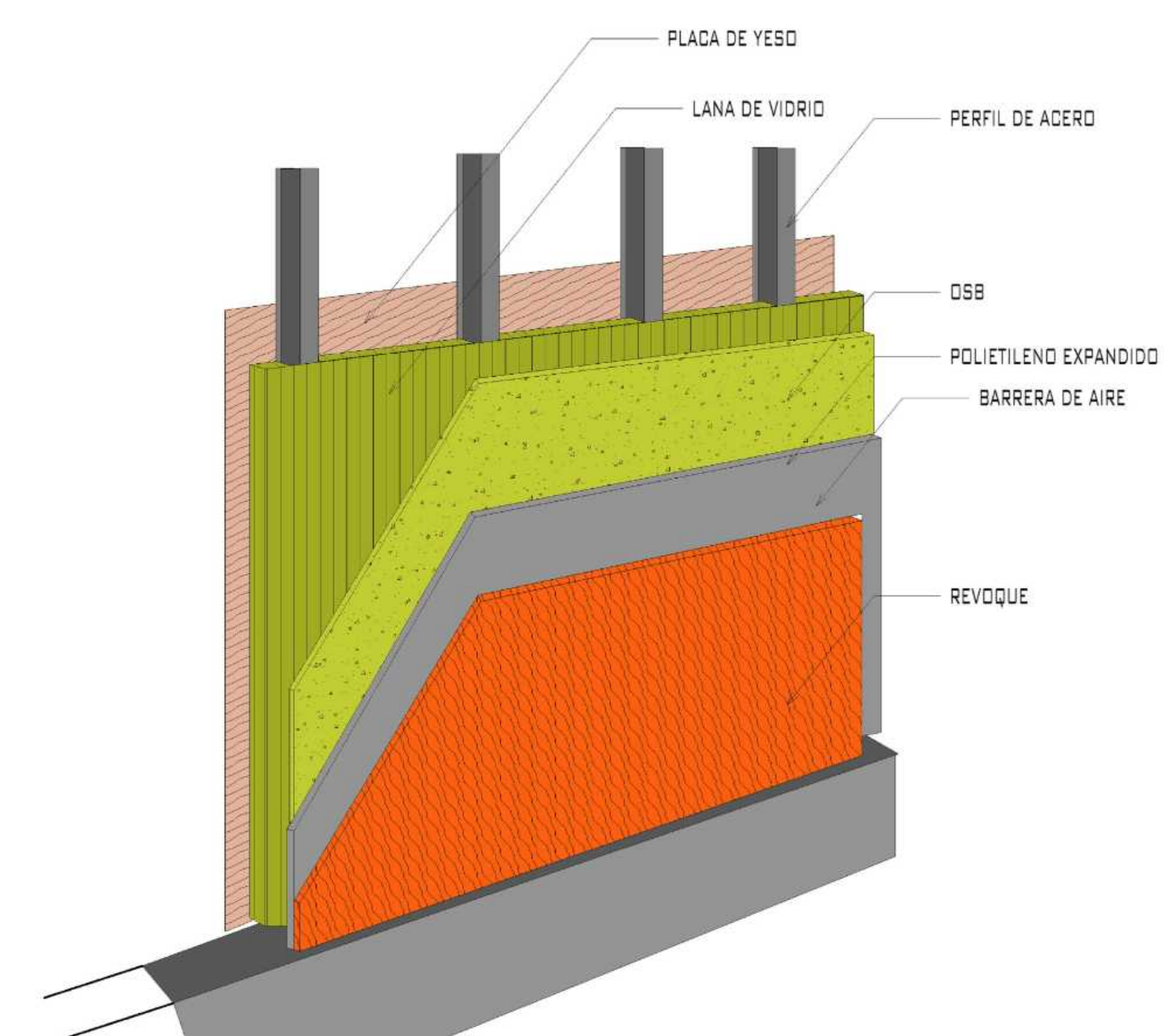
DETALLE DE MURO EN SECO
