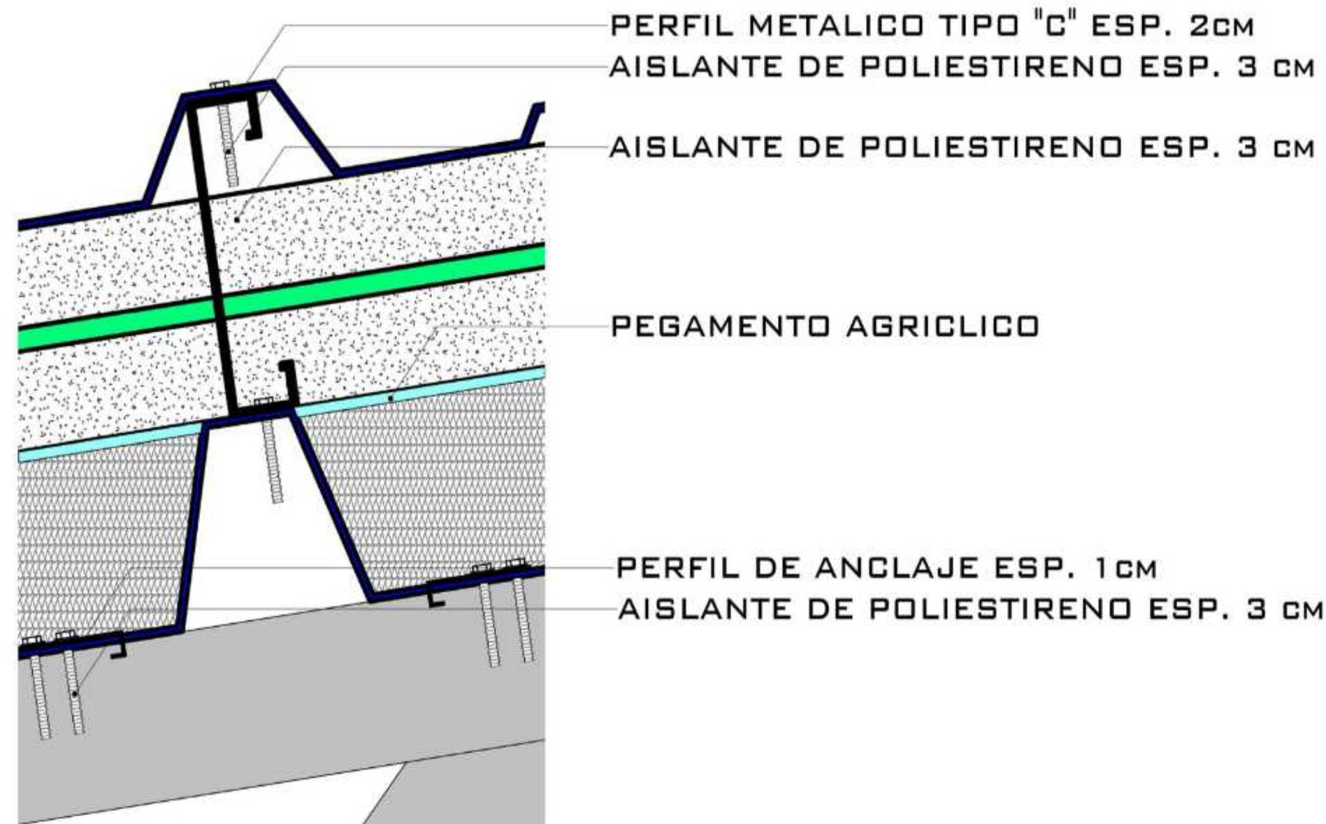
DETALLE DE UNIONES ESC:1:2
