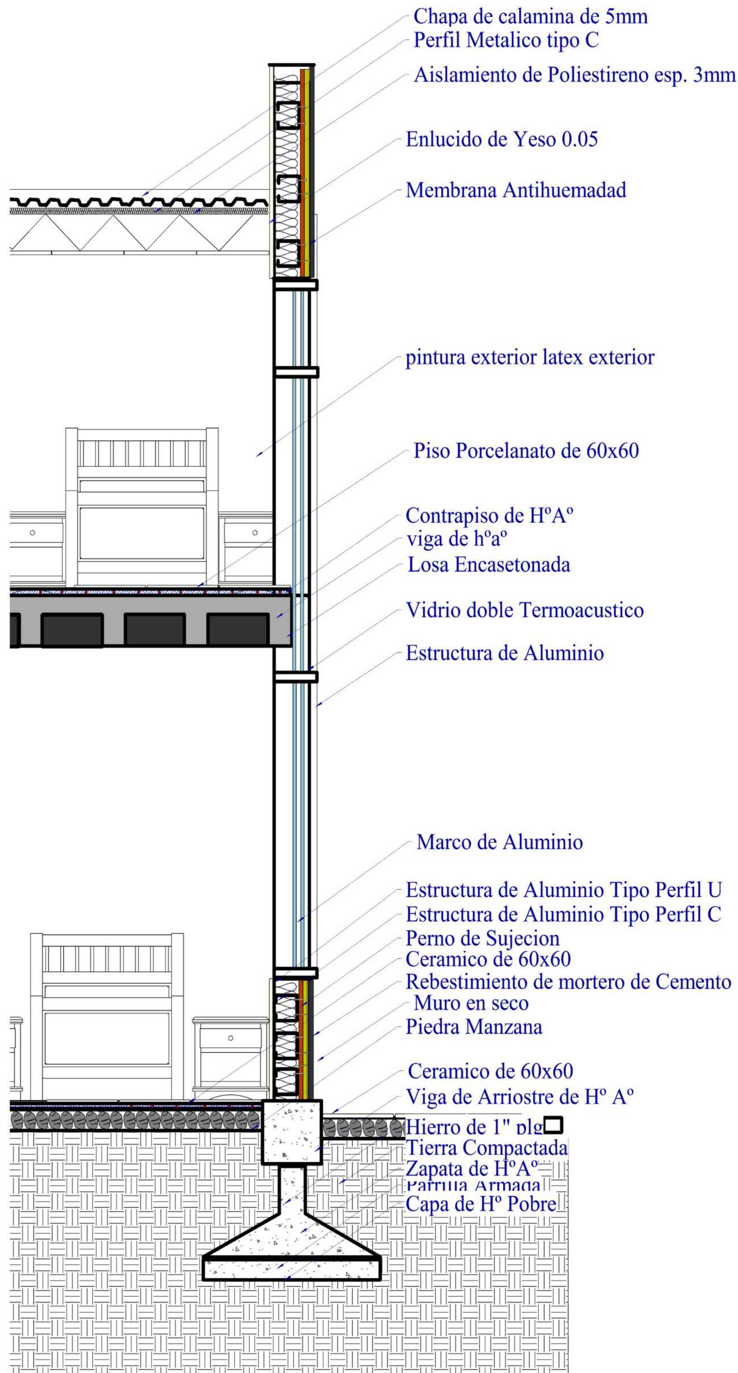
CORTE DE BORDE ( ÁREA HABITACIONAL) ESC: 1:20
