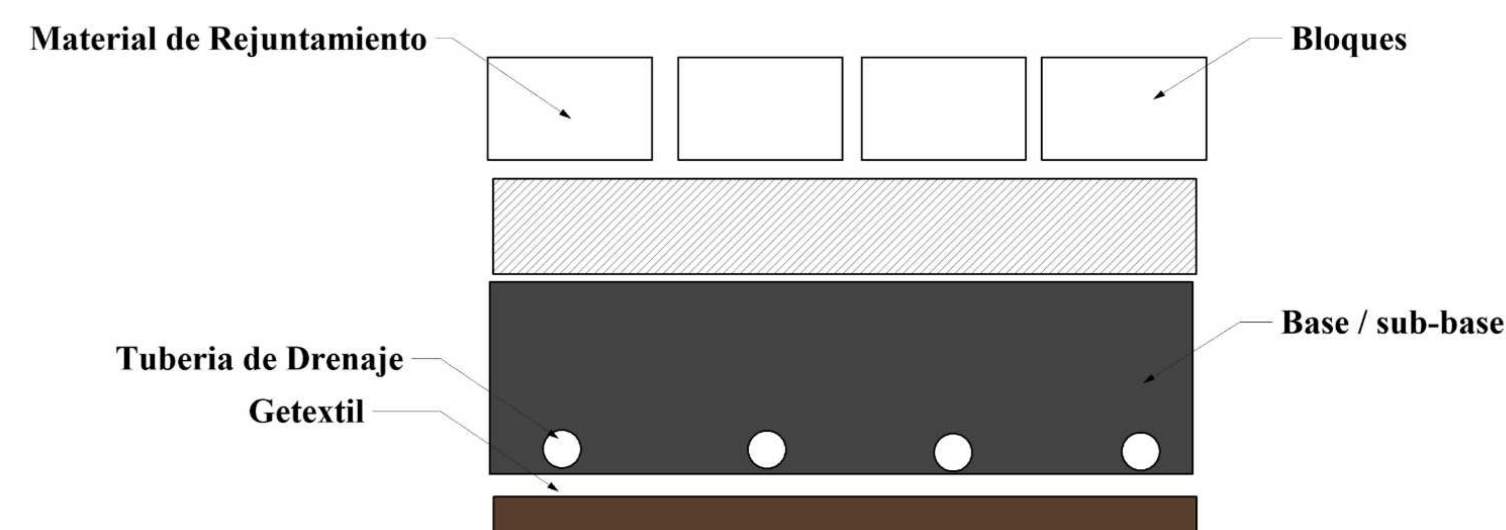
DETALLE DE DRENAJE SOSTENIBLE (SUDS) / SECTOR ESTACIONAMIENTO
