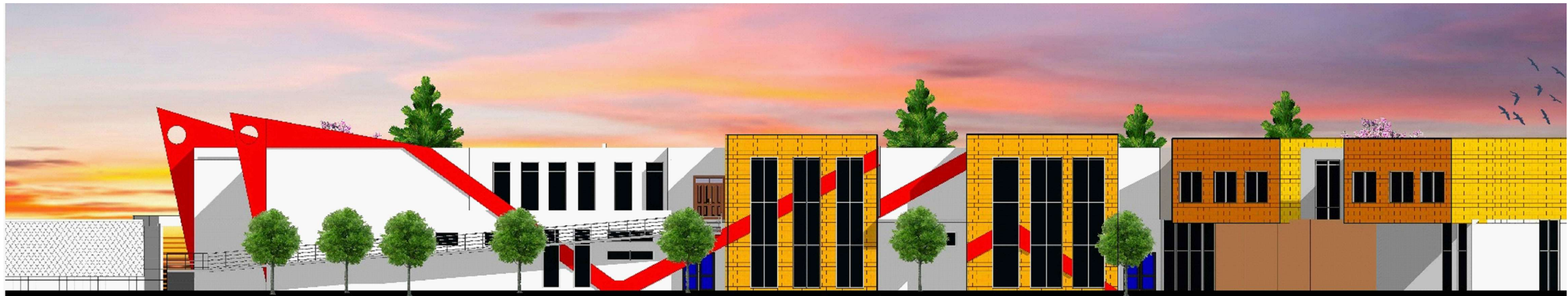
FACHADA LATERAL NOROESTE ESC 1/200 INSTITUTO DE INVESTIGACIÓN Y CAPACITACIÓN PECUARIA
