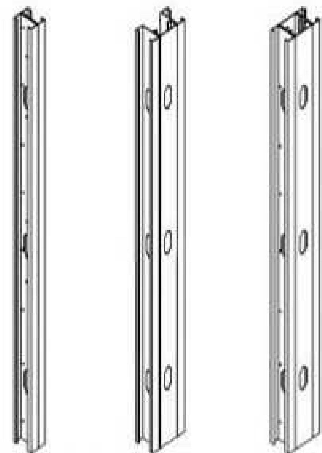
PERFILES DE ACERO PARA MURO EN SECO
