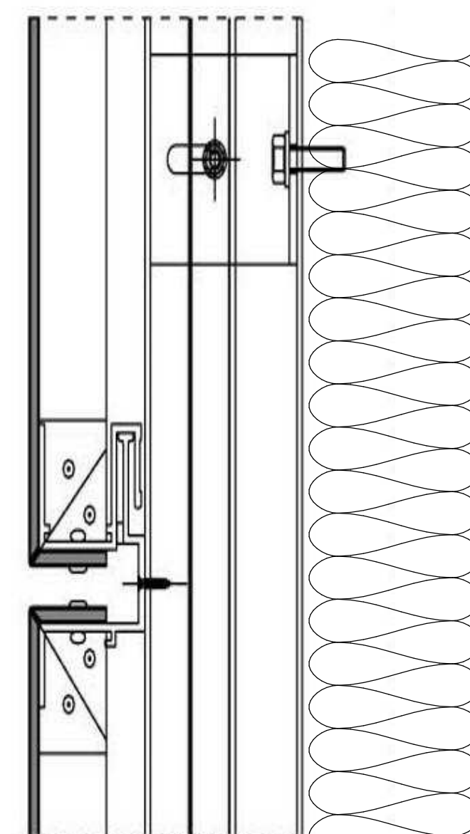
SECCION VERTICAL
