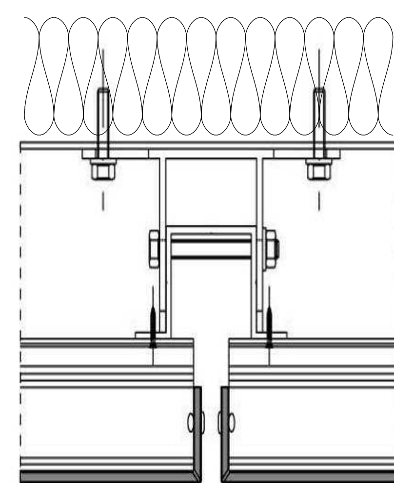
SECCION HORIZONTAL
