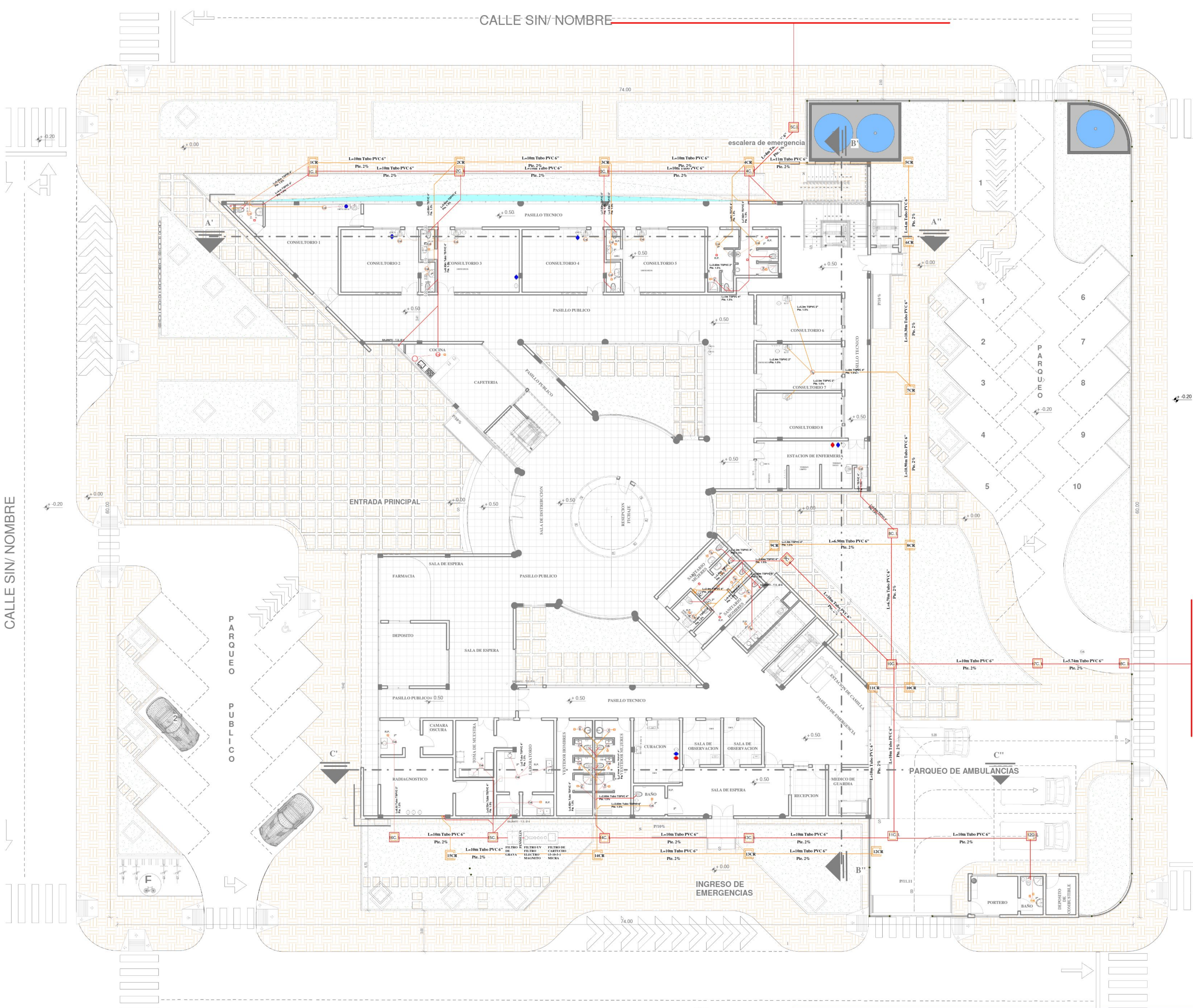
PLANTA BAJA INSTALACIÓN SANITARIO ESC. 1:100
