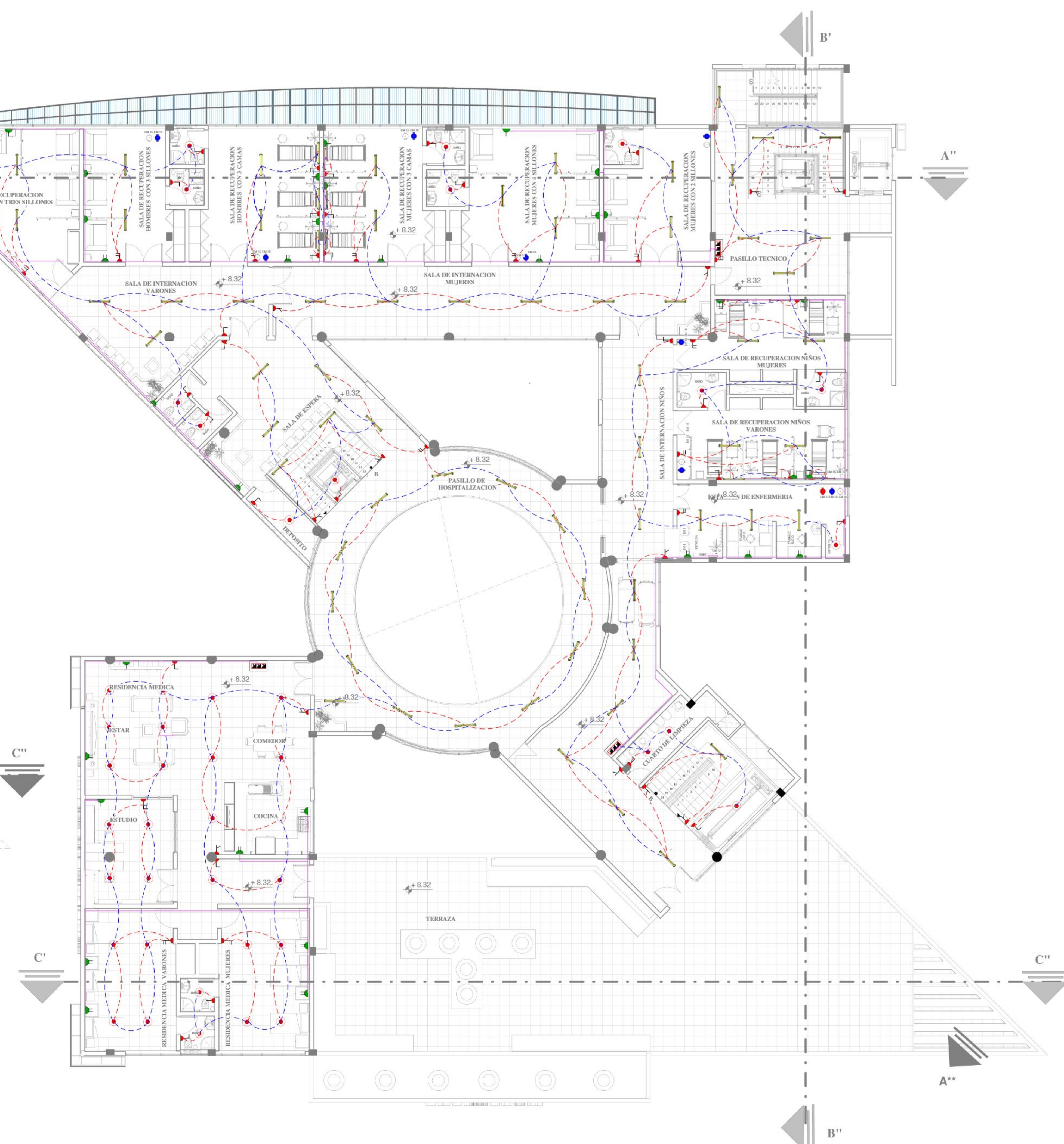
SEGUNDO PISO INSTALACIÓN ELÉCTRICA ESC. 1:100
