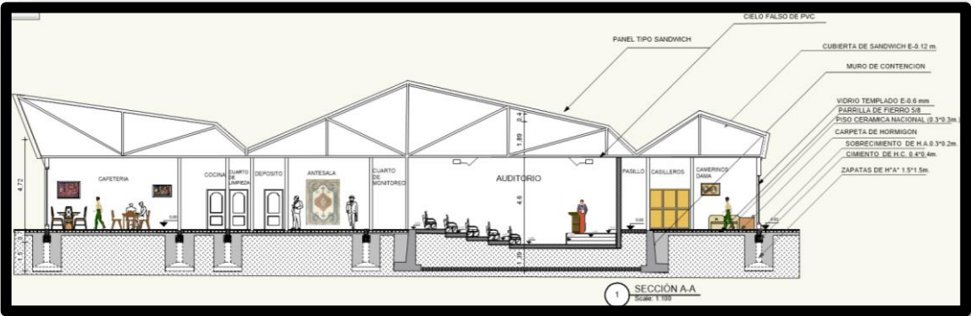
SECCION A-A''
