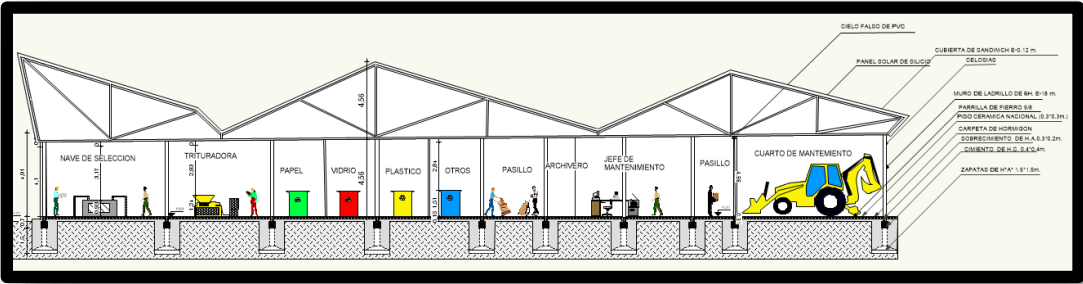
SECCION B-B''
