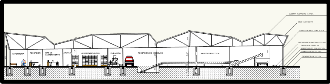
SECCION D-D''
