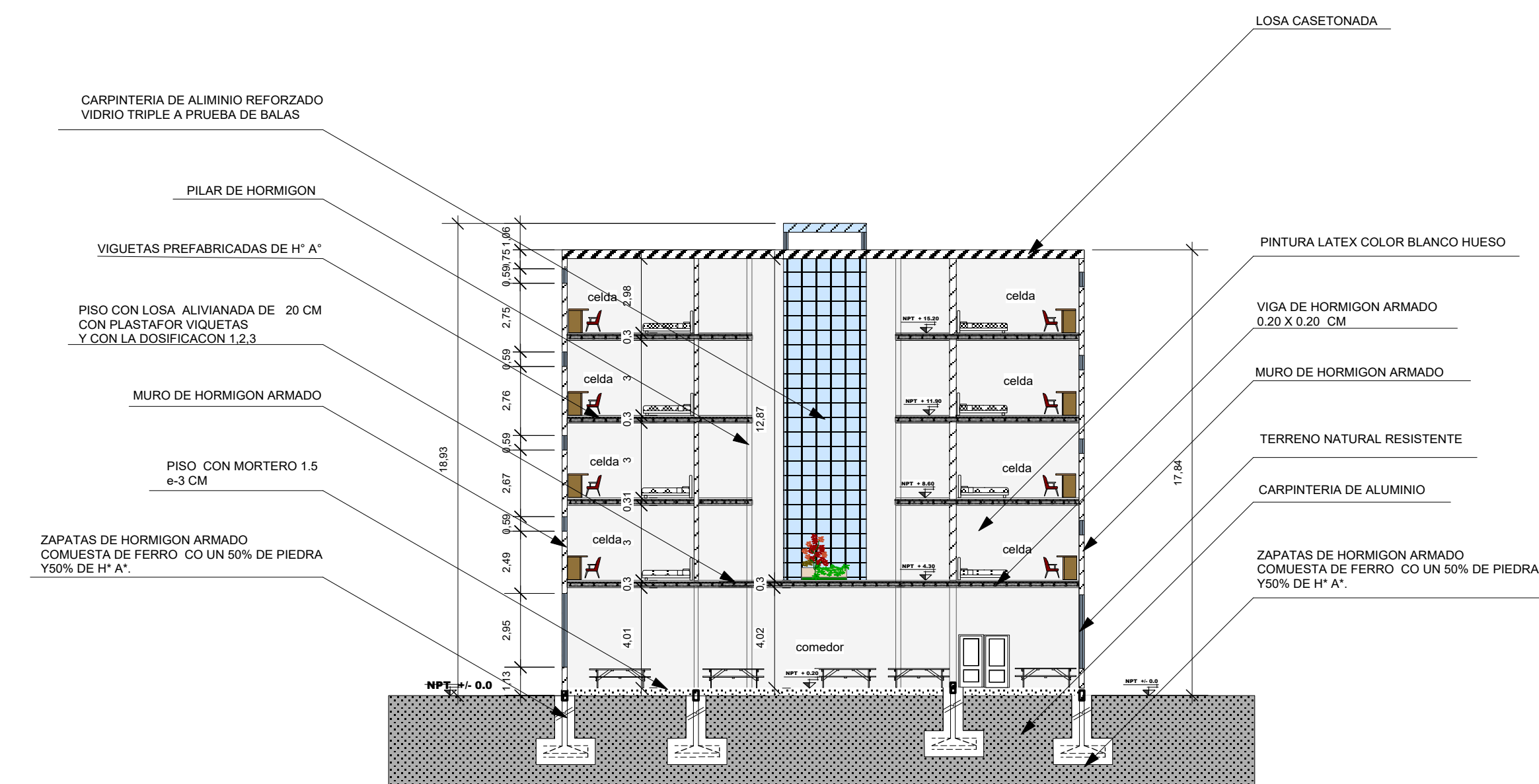
CORTE C-C' ESCALA: 1:100
