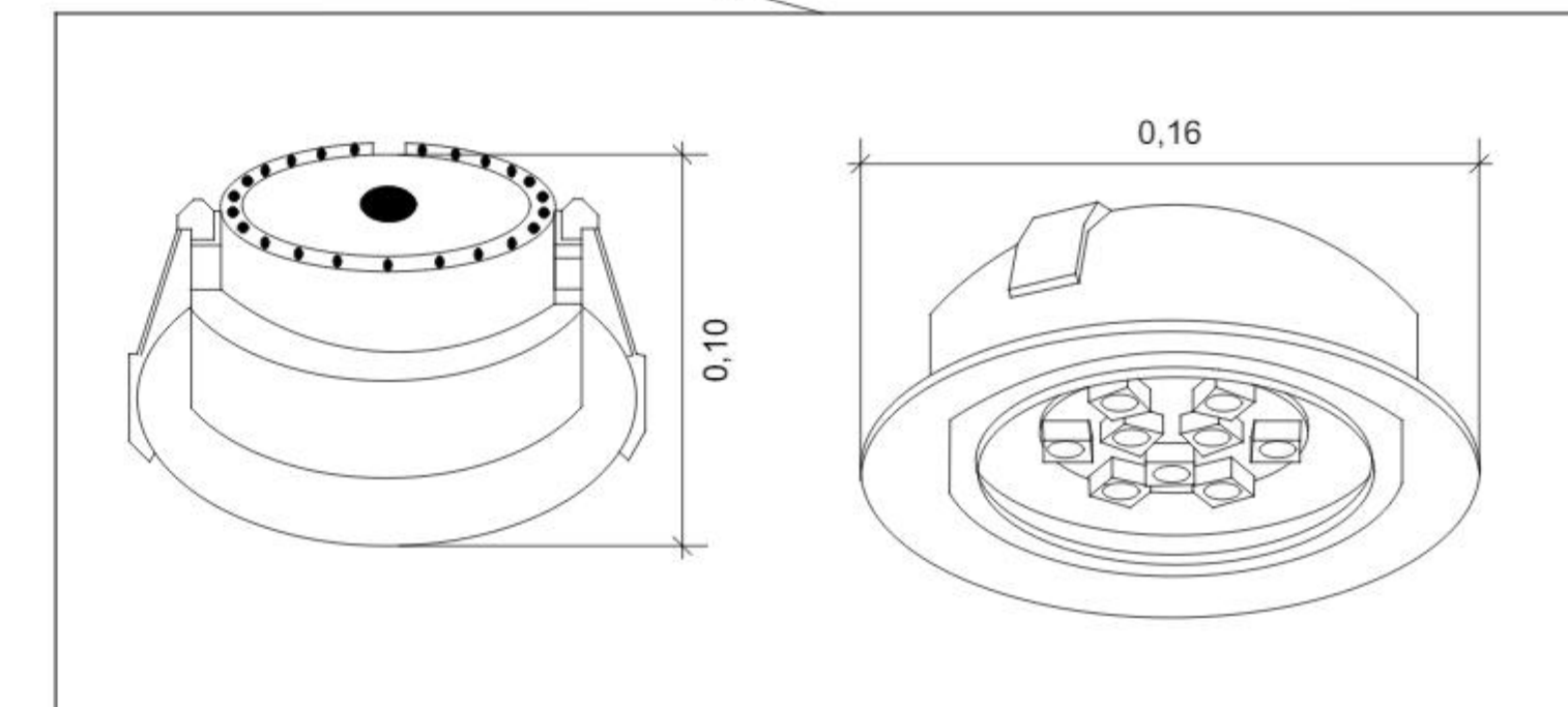
LUMINARIA FOTOVOLTAICA ESC: 1;2
