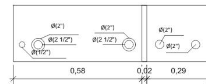
DETALLE CAJA DE INTERRUPTORES ESC: 1;10
