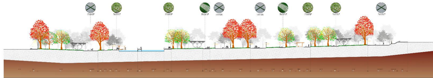
CORTE G-G'
