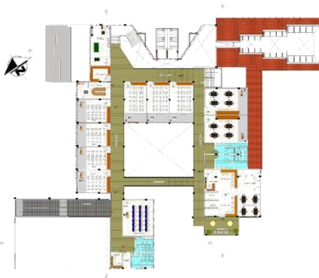
PLANTA ALTA AMOBLADA ESC:1:100
