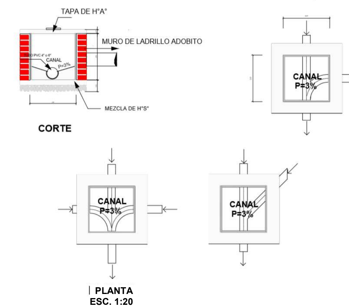
DETALLE CONSTRUCTIVO - CAMARA DE INSPECCION (TIPOS)
