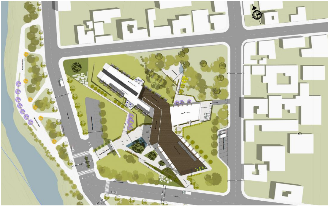
PLANIMETRIA.
