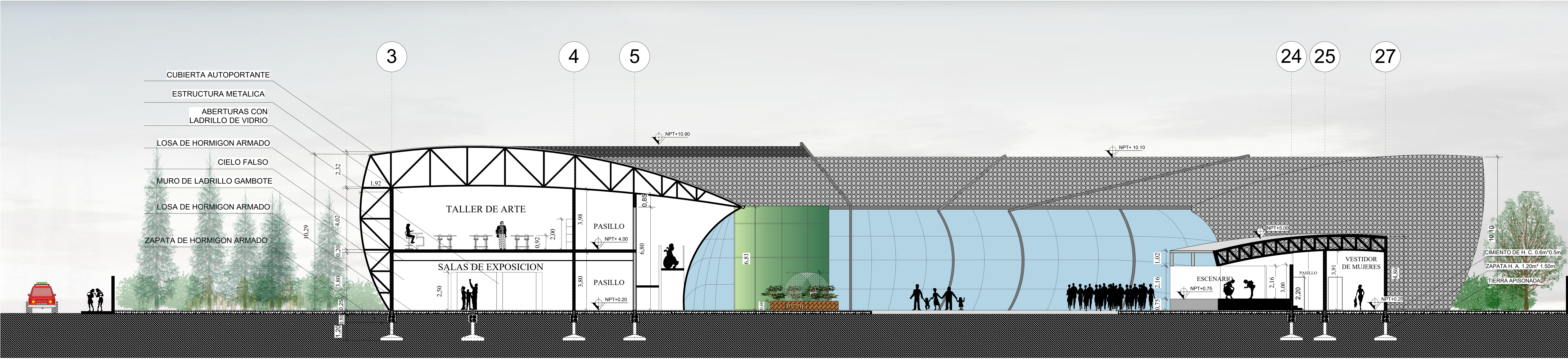
CORTE A' - A''
