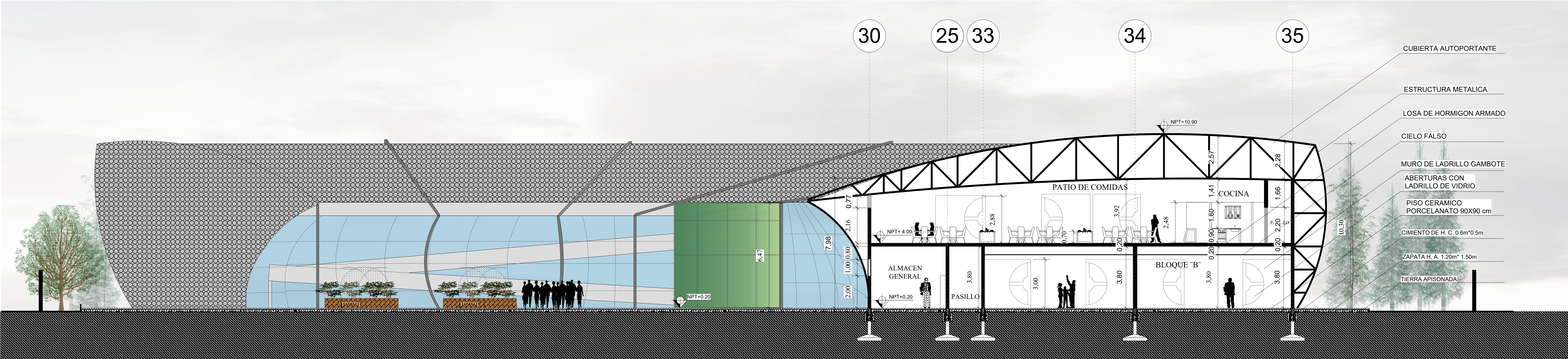
CORTE B'- B''
