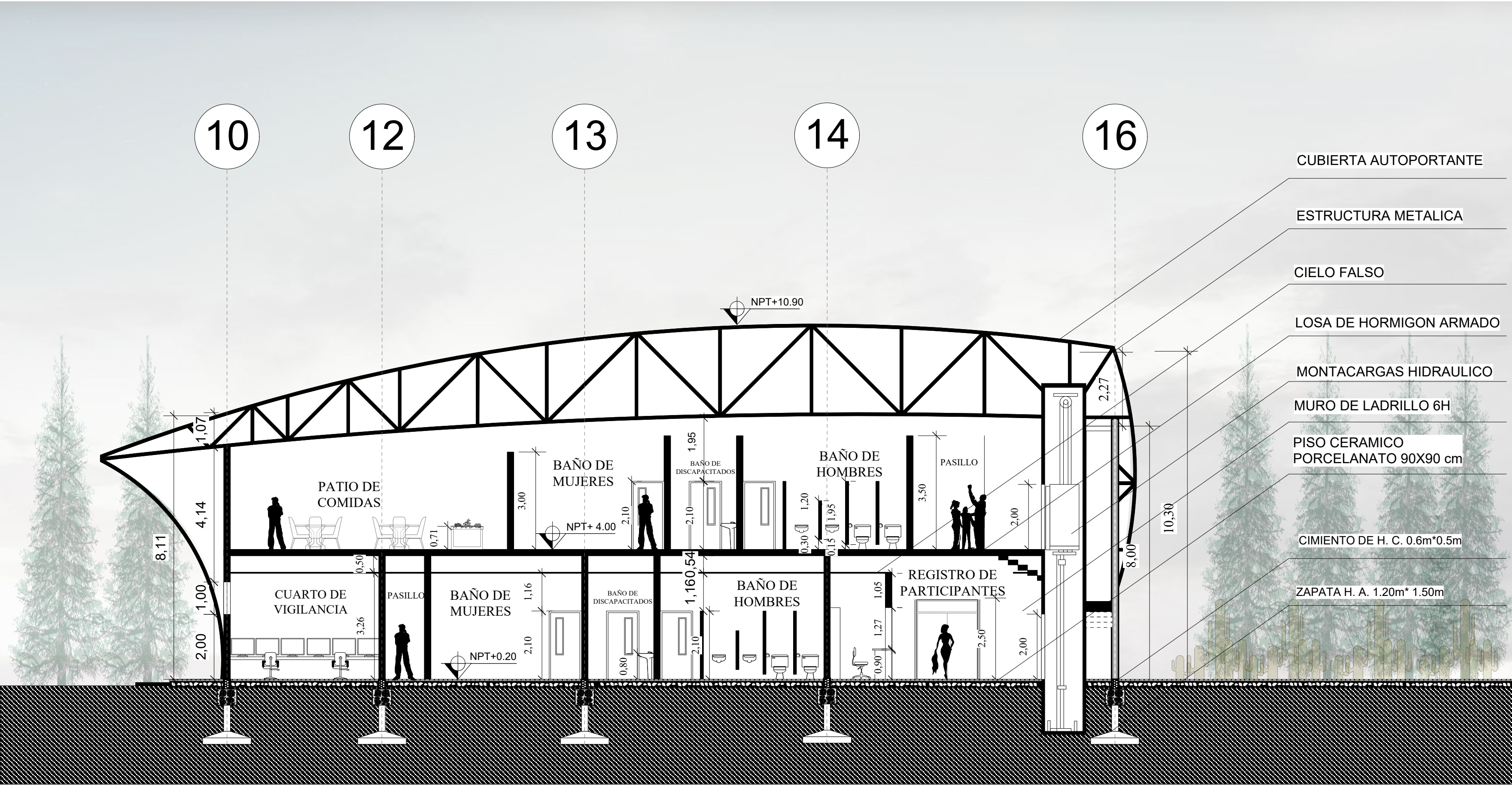
CORTE D'- D''
