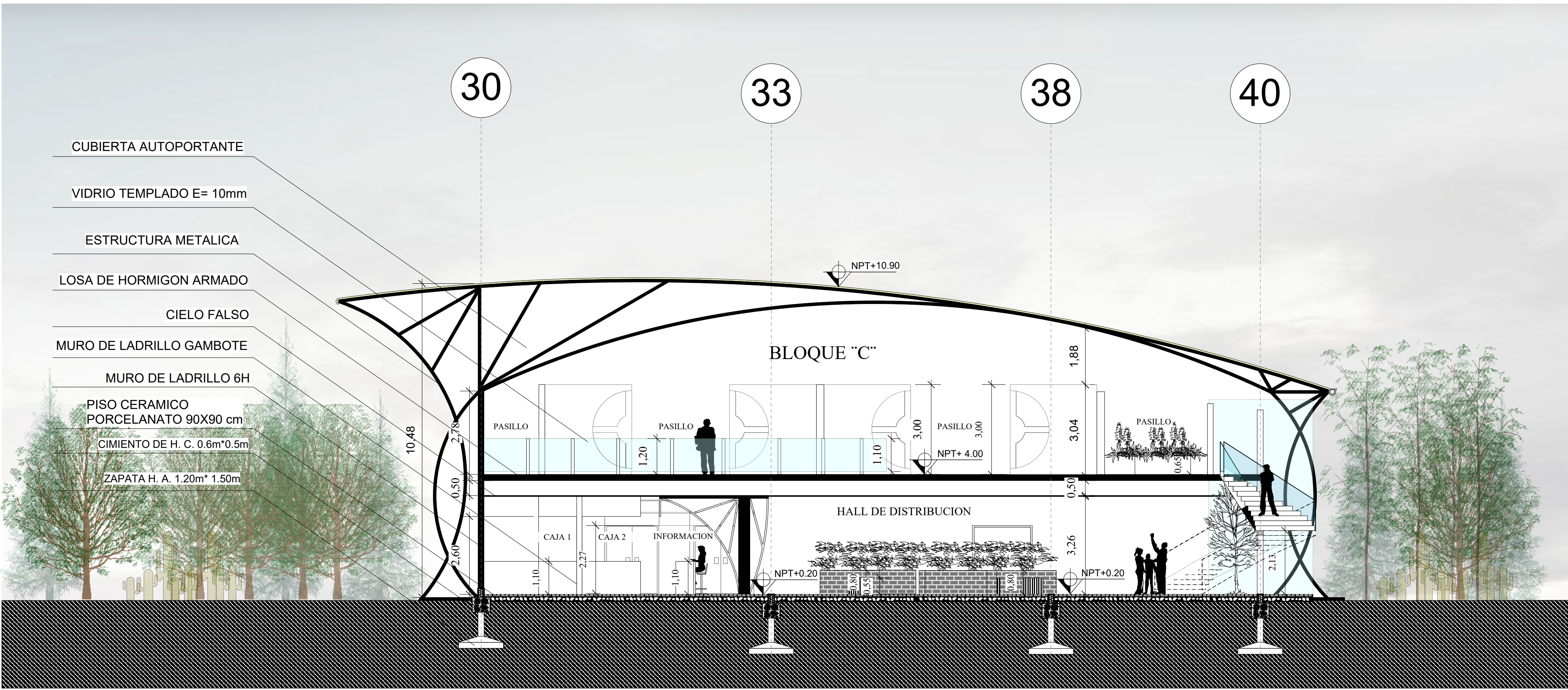
CORTE C' - C''
