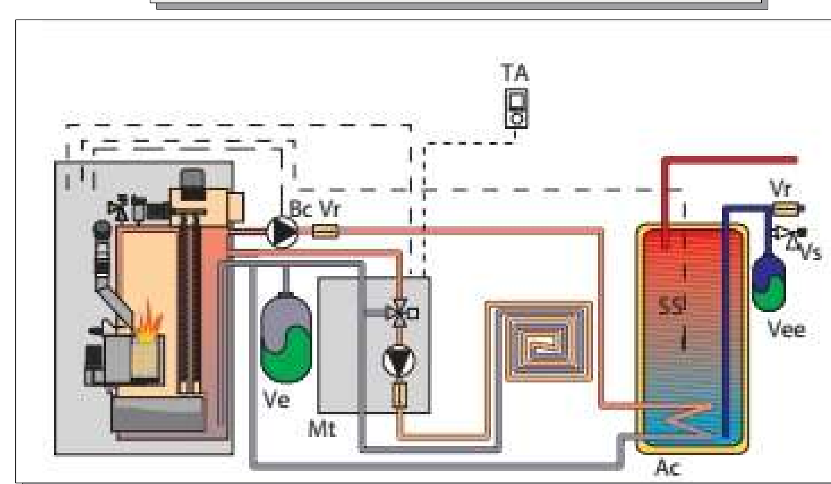
DIAGRAMA DE CALDERO
