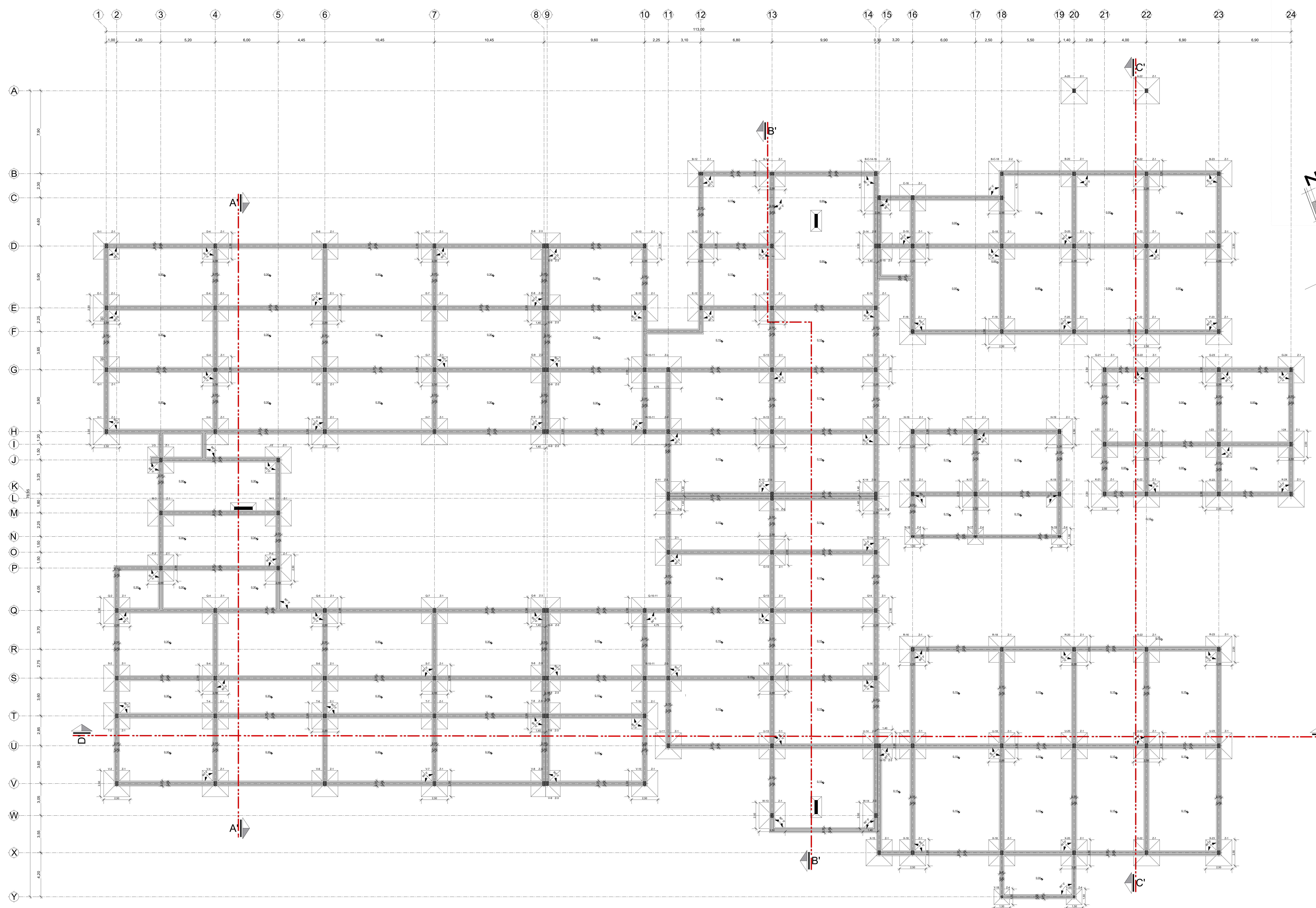
Esc: 1:120 Plano de Cimientos
