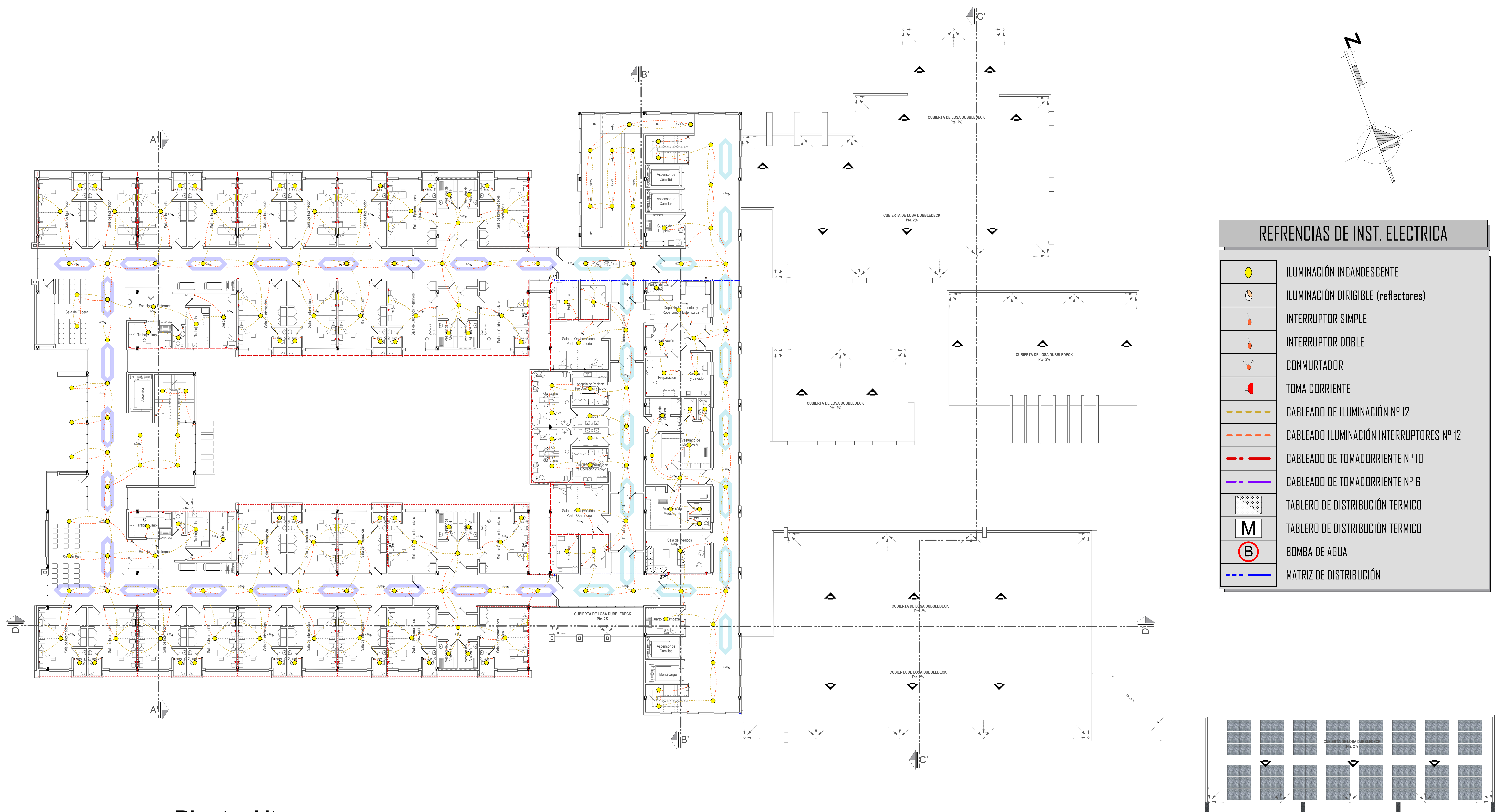
Esc: 1:120 Planta Alta Instalación Eléctrica
