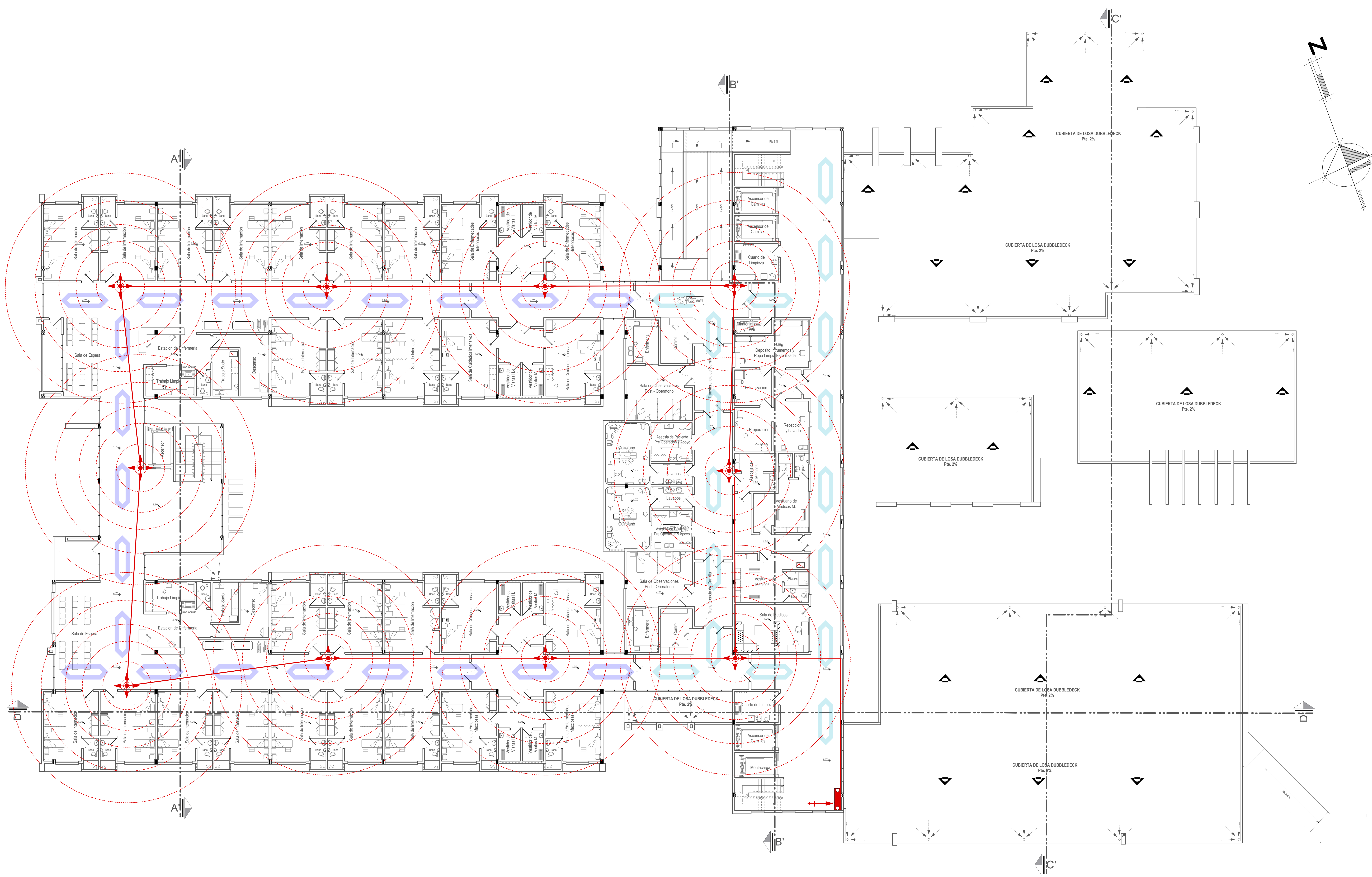
Esc: 1:120 Planta Alta Instalación Wifi
