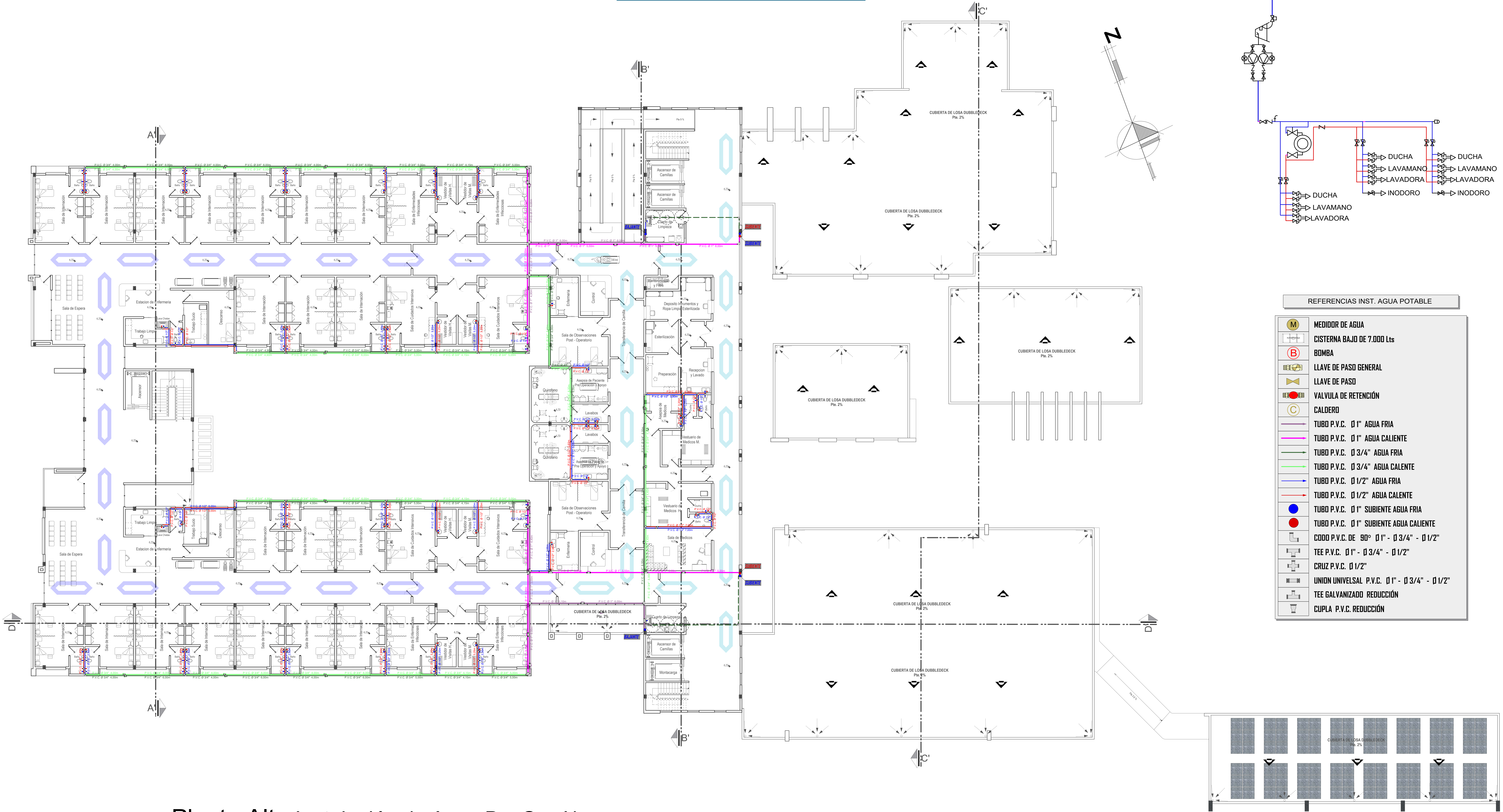
Esc: 1:120 Planta Alta Instalación de Agua P. - Gas N.
