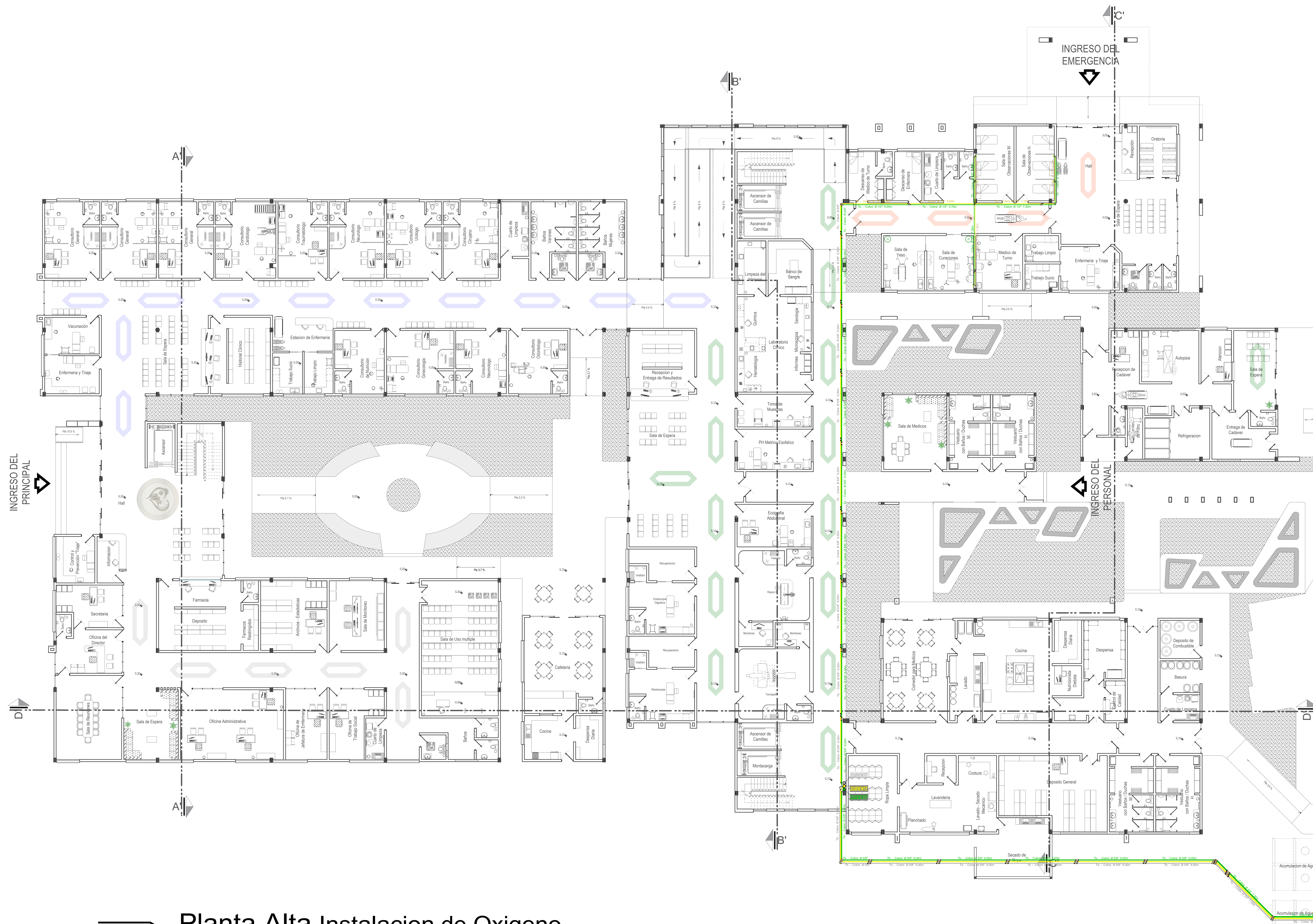
Esc: 1:120 Planta Alta Instalacion de Oxigeno
