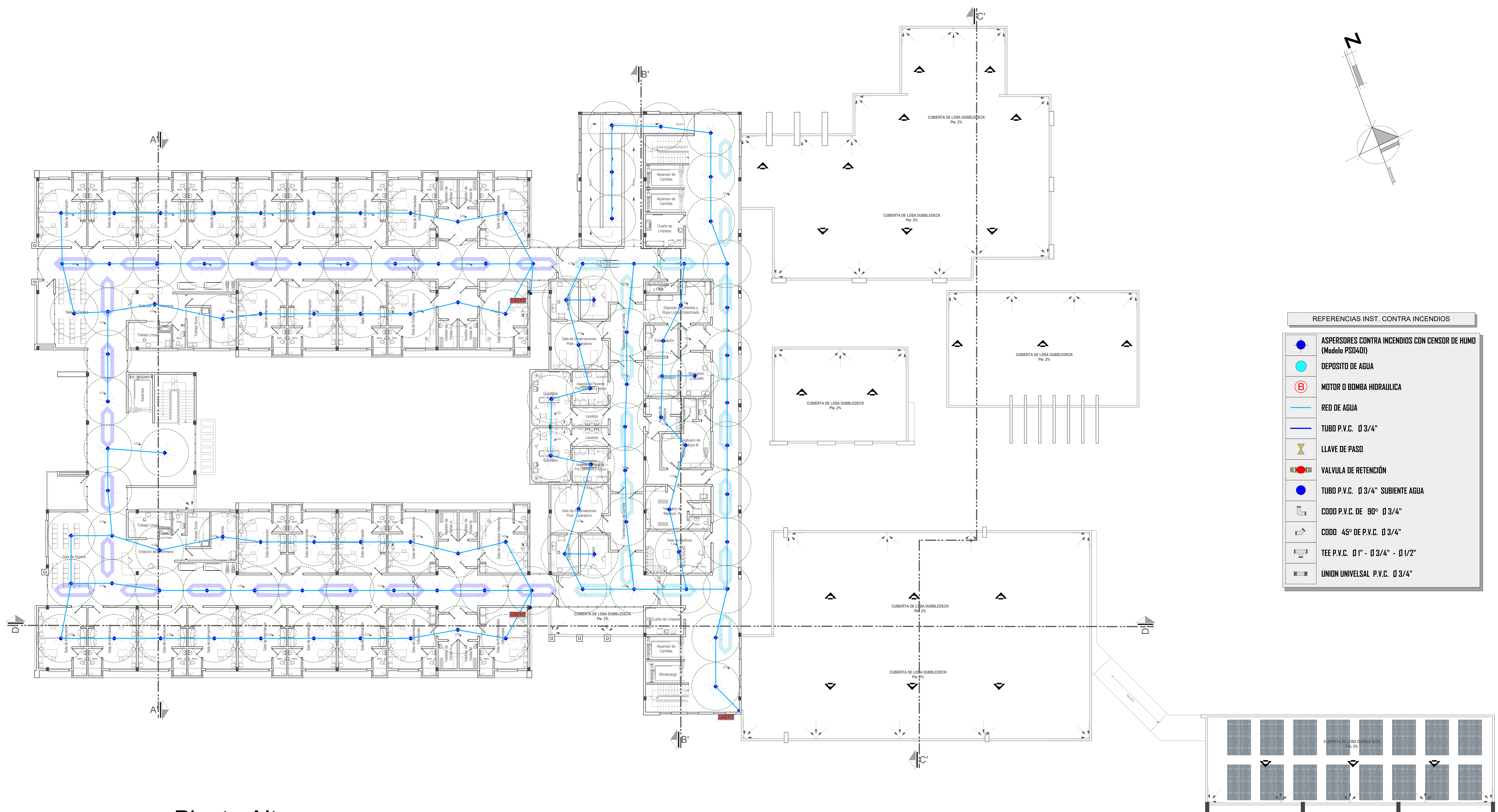
Esc: 1:120 Planta Alta Instalación Contra Incendios
