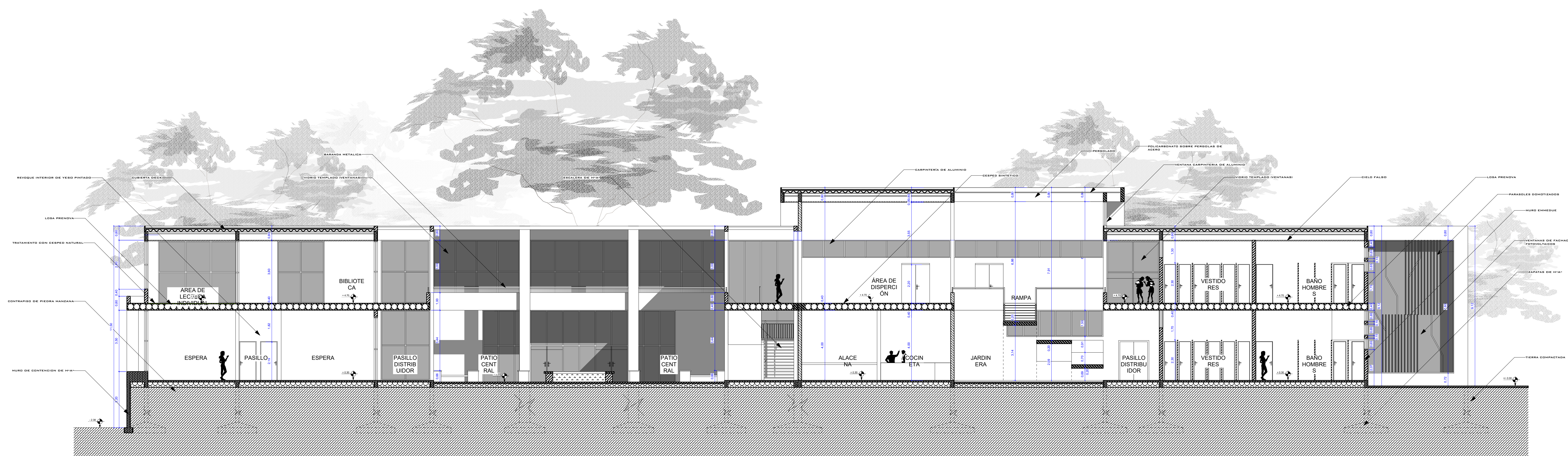
CORTE C-C
