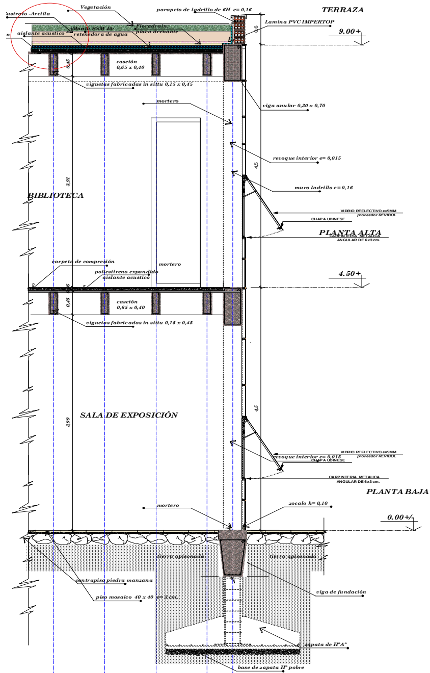
DETALLE MURO CORTINA ESC. 1:20
