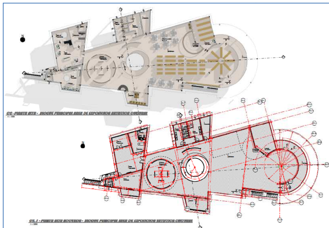
PLANTA BAJA –PLANO ACOTADO Y AMOBLADO DEL BLOQUE PRINCIPAL DE EXPOSICIÓN ARTÍSTICA
