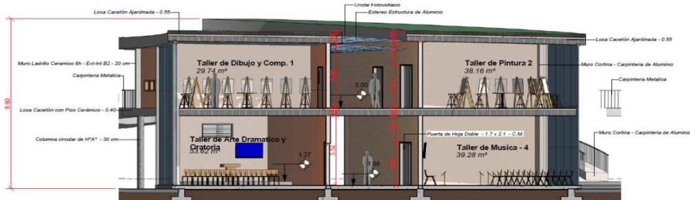
CORTE D - BLOQUE DE TALLERES - ESC: 1:100
