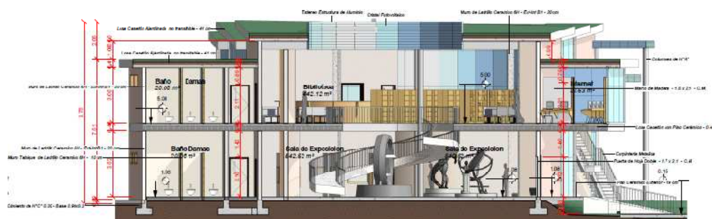
CORTE B- BLOQUE PRINCIPAL DE EXPOSICIÓN ARTÍSTICA- ESC: 1:100
