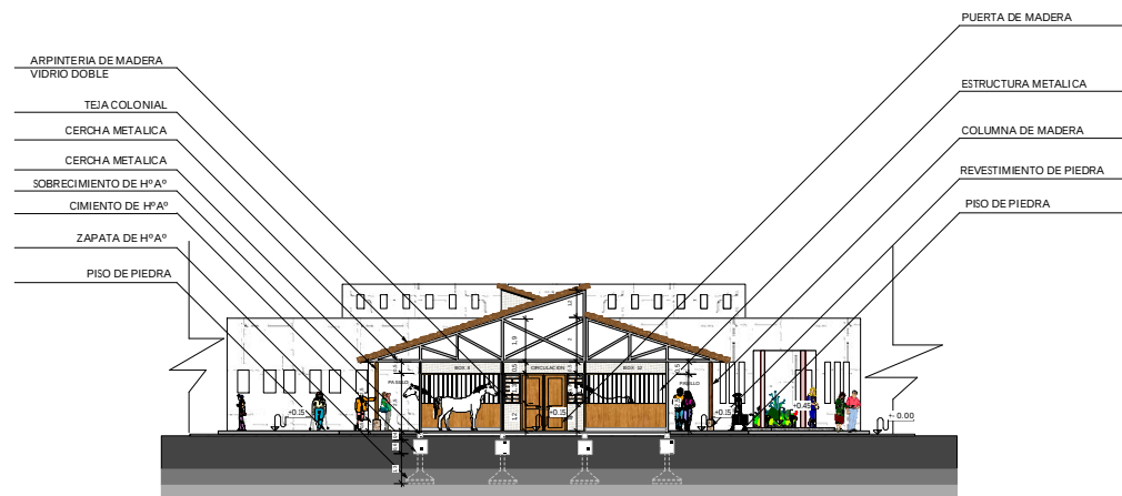
CORTE FACHADA A - A' ESC. 1:200
