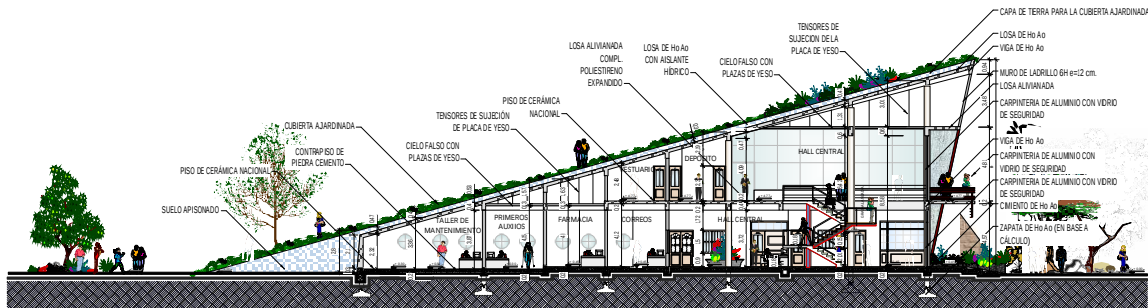
CORTE A - A' ESC. 1:200
