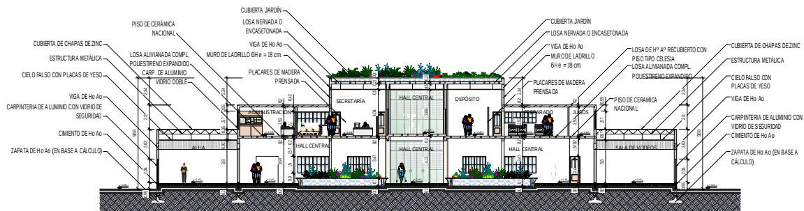
CORTE B - B' ESC. 1:200
