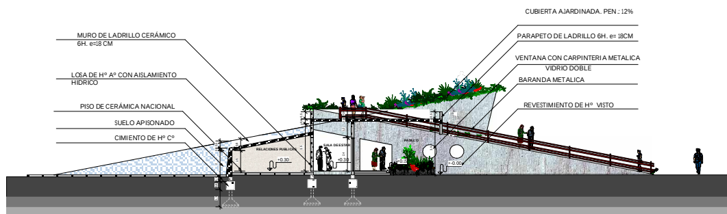
CORTE FACHADA B - B"
