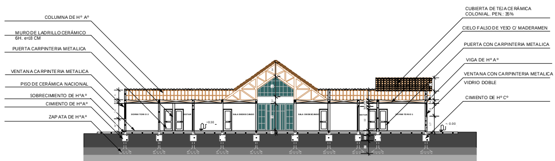
CORTE A - A" ESC. 1:200
