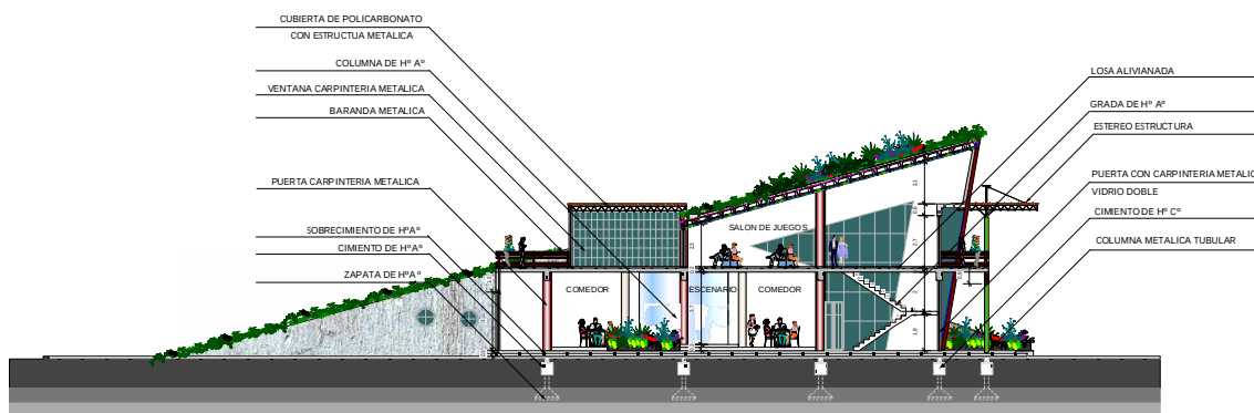
CORTE FACHADA A - A" ESC. 1:200
