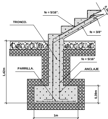
DETALLE DE CIMIENTO O ARRANQUE DE LA ESCALERA HELICOIDAL.
