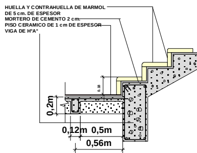
DETALLE REVESTIMIENTO DE ESCALERA
