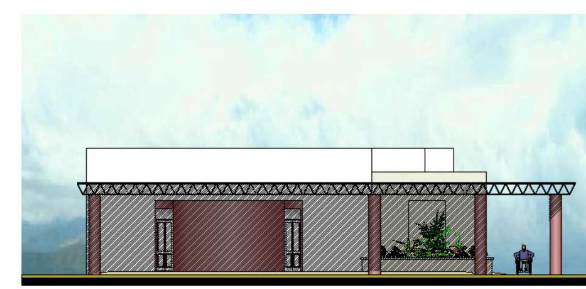
FACHADA FRONTAL DE SALON MULTIUSO Escala: 1:100
