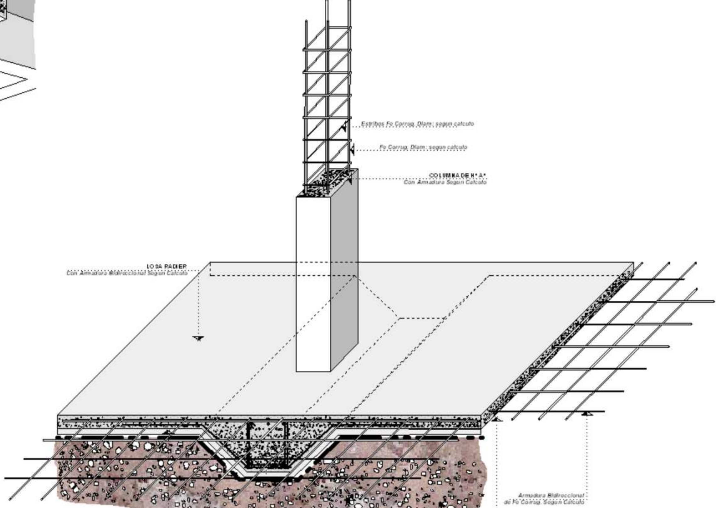
DETALLE FUNDACIONES Y COLUMNAS
