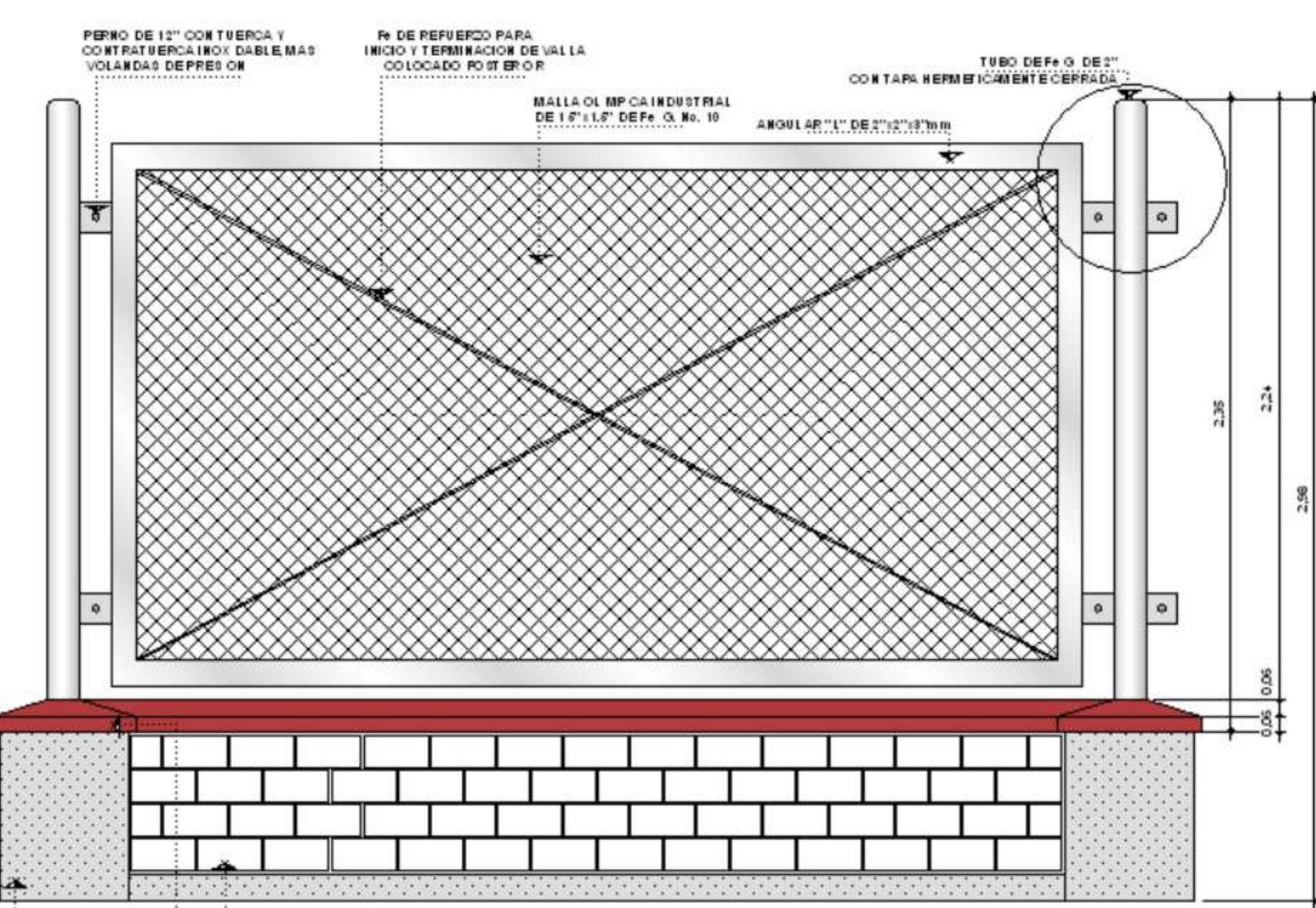
DETALLE CERRAMIENTO PERIMETRAL
