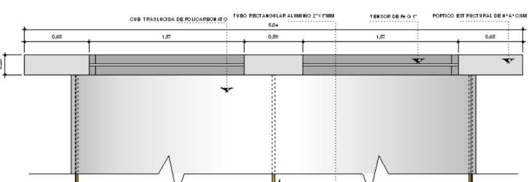
DETALLE ENTREPISO Y CUBIERTA
