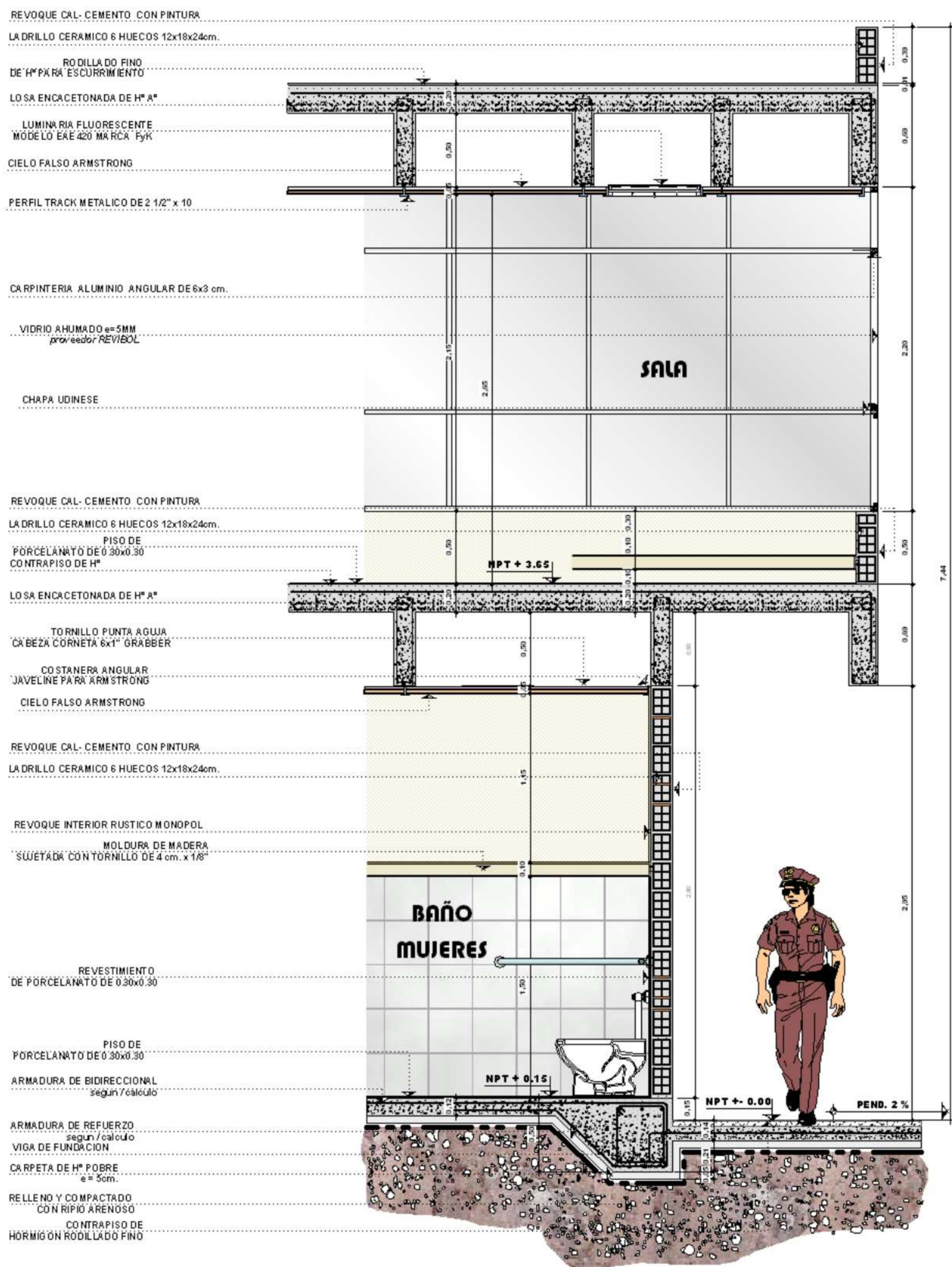
CORTE DE BORDE 01-RES
