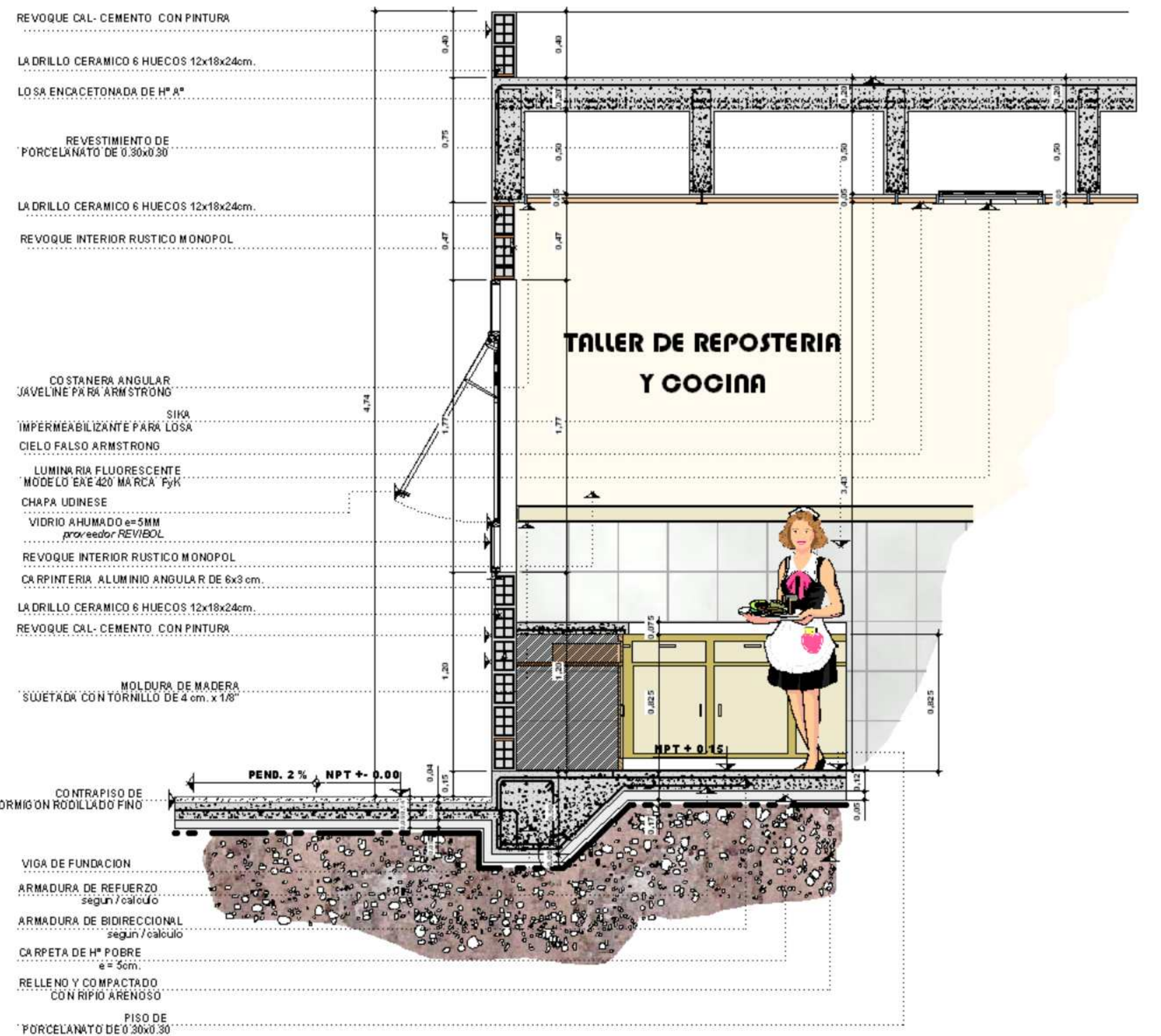
CORTE DE BORDE 02-TAL
