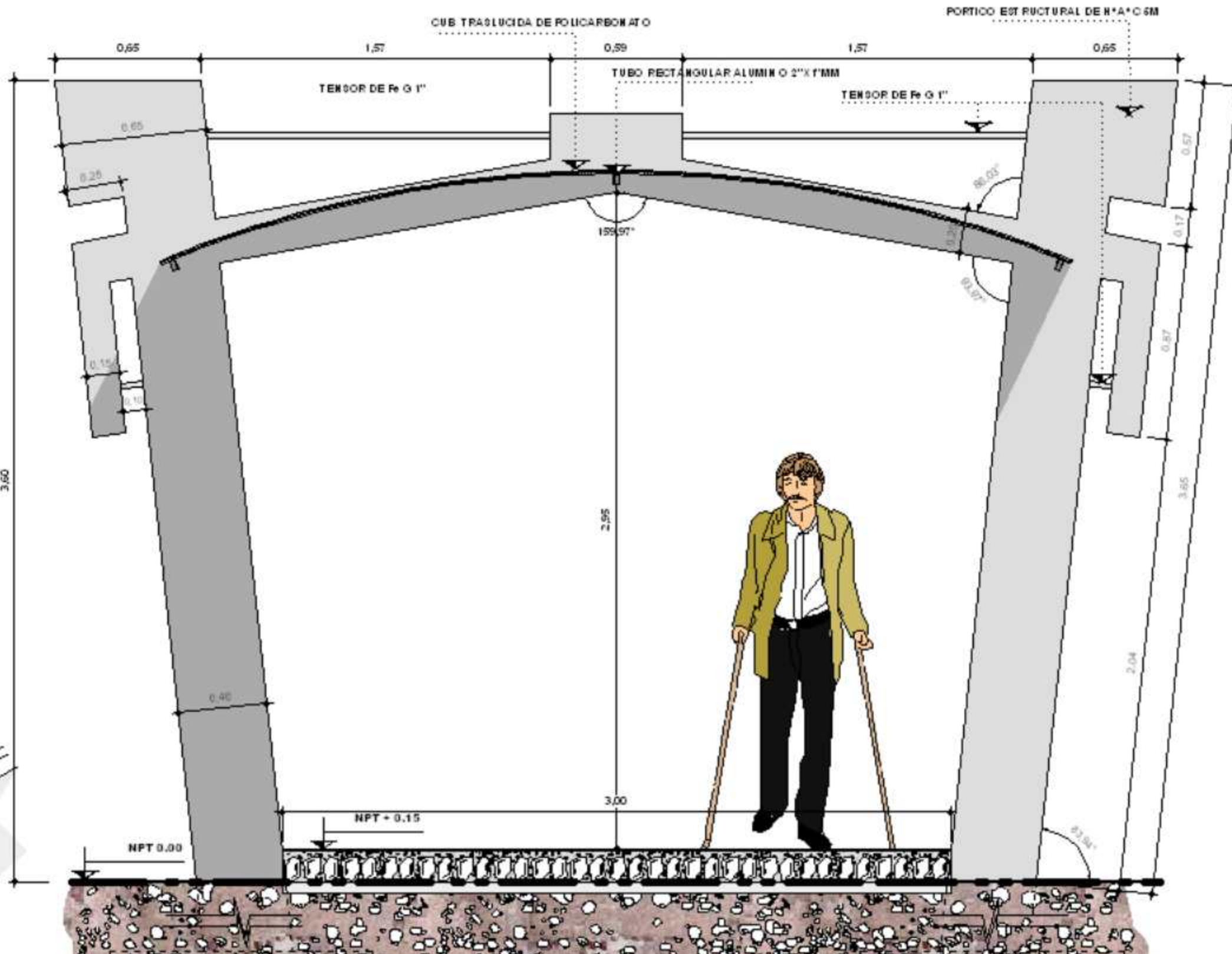
DETALLE CIRCULACION EXTERIOR CUBIERTA
