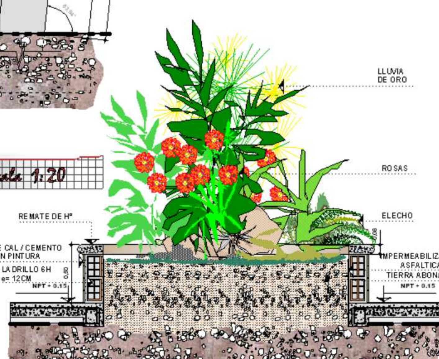
DETALLE JARDINERAS INTERNAS
