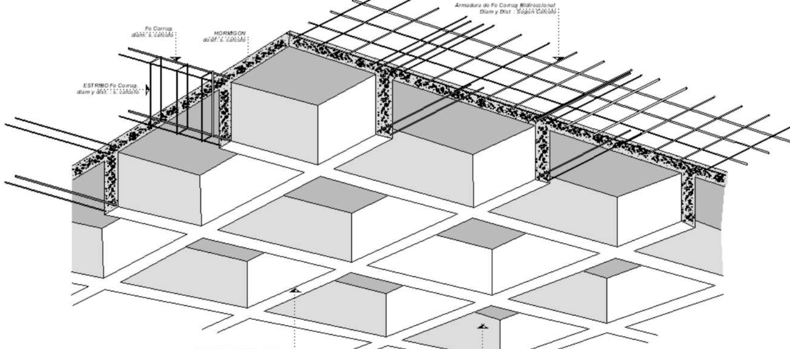
DETALLE ENTREPISO Y CUBIERTA
