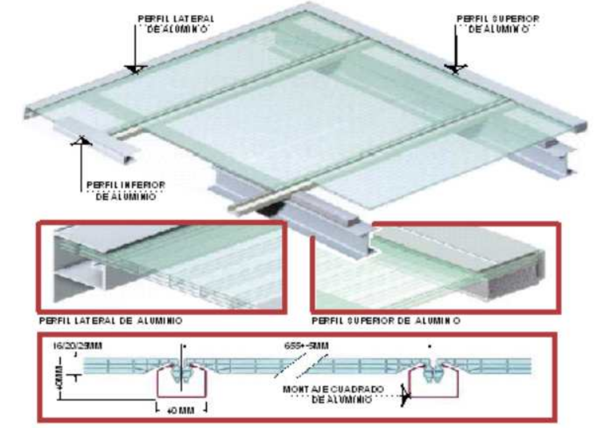
DETALLE CUBIERTAS TRASLUCIDAS
