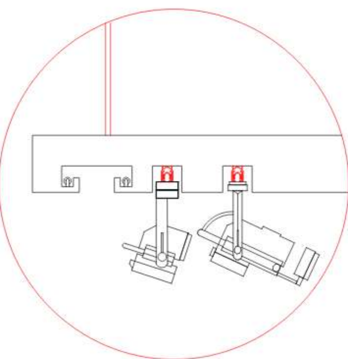
GARGANTA CON TUBOS FLUORESCENTES Y RIELES TRIFÁSICOS C/ PROYECTORES
