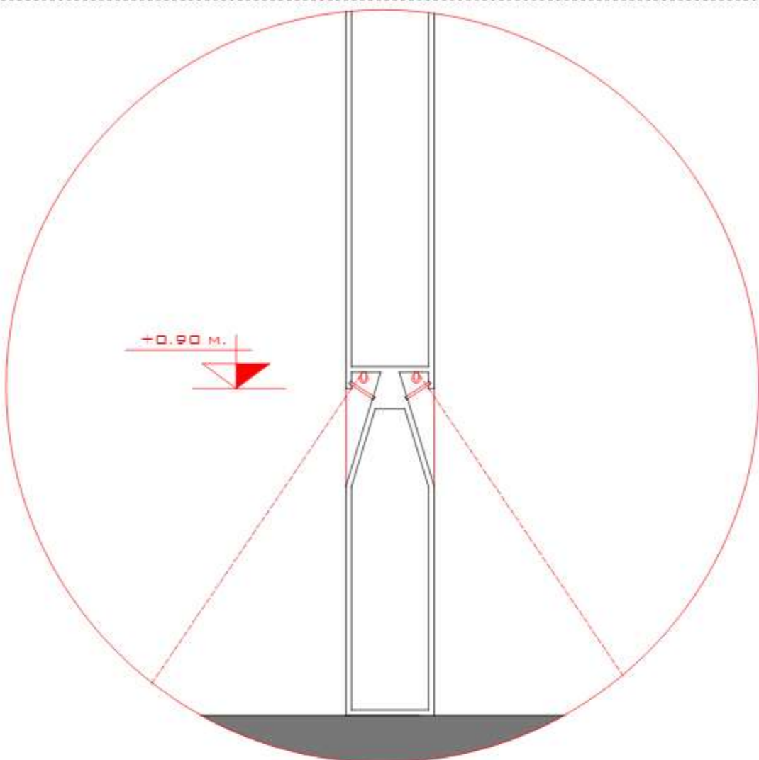
DET.22 Tubos fluorescentes p/efecto bañado de piso
