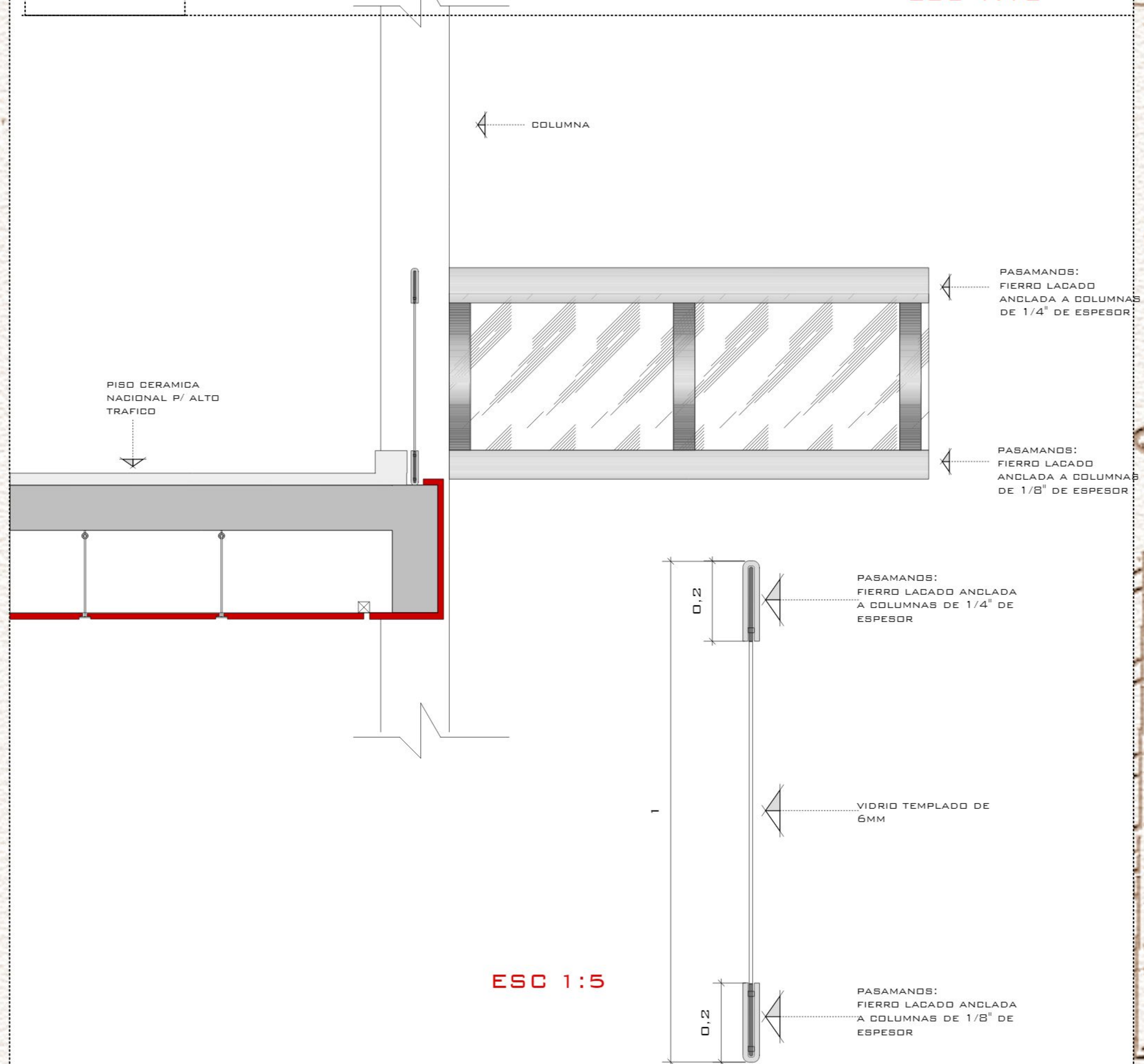
DET.17 DETALLE DE BARANDA
