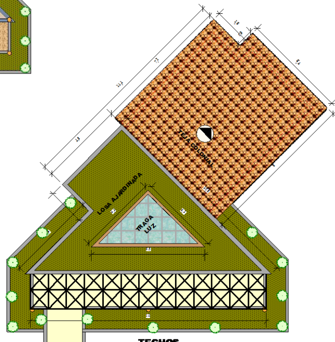
TECHOS ESC. 1:100
