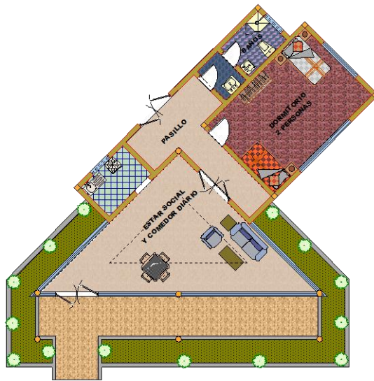
PLANTA AMOBLADA CABAÑA TIPO III PARA 2 PERSONAS ESC. 1:100
