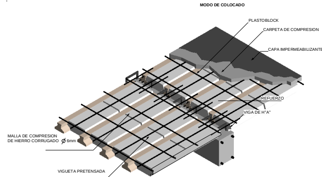
DETALLE DE LOSA ALIVIANADA COMPLEMENTO DE LADRILLO
