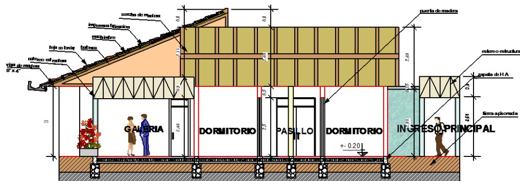
CORTE A A' ESC. 1:100
