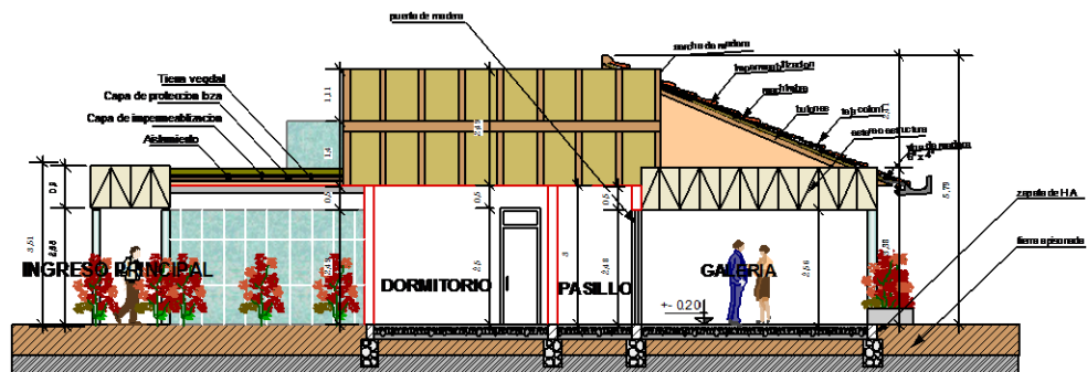
CORTE A A' ESQ. 1.100
