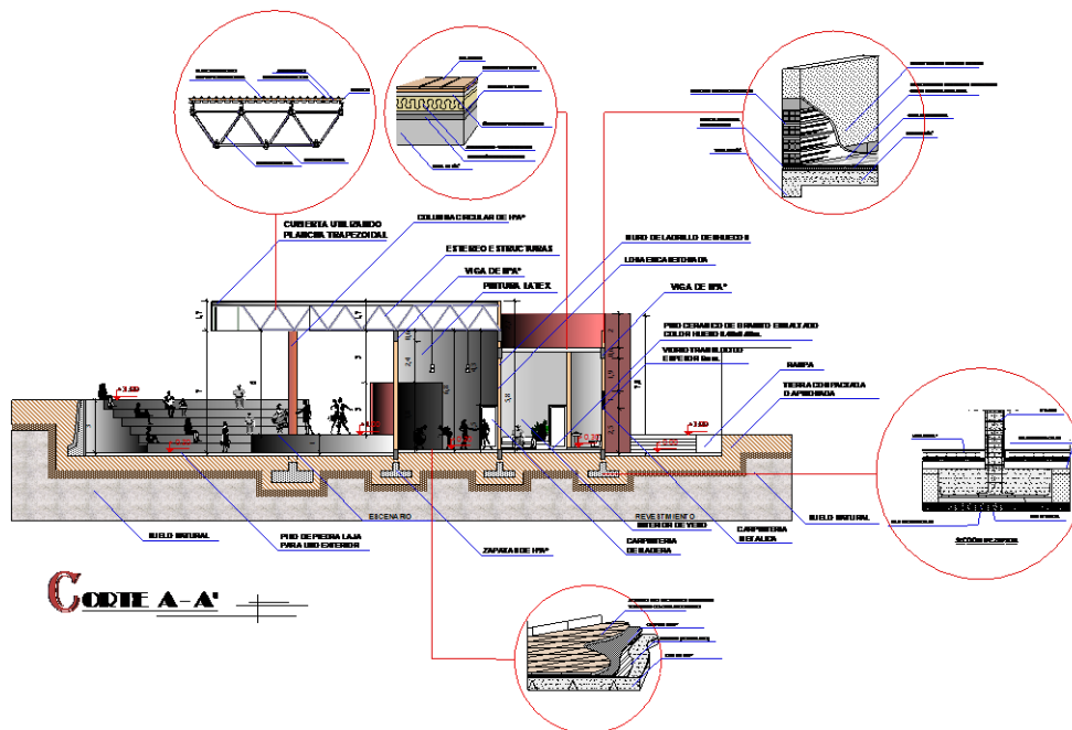
CORTE A-A'
