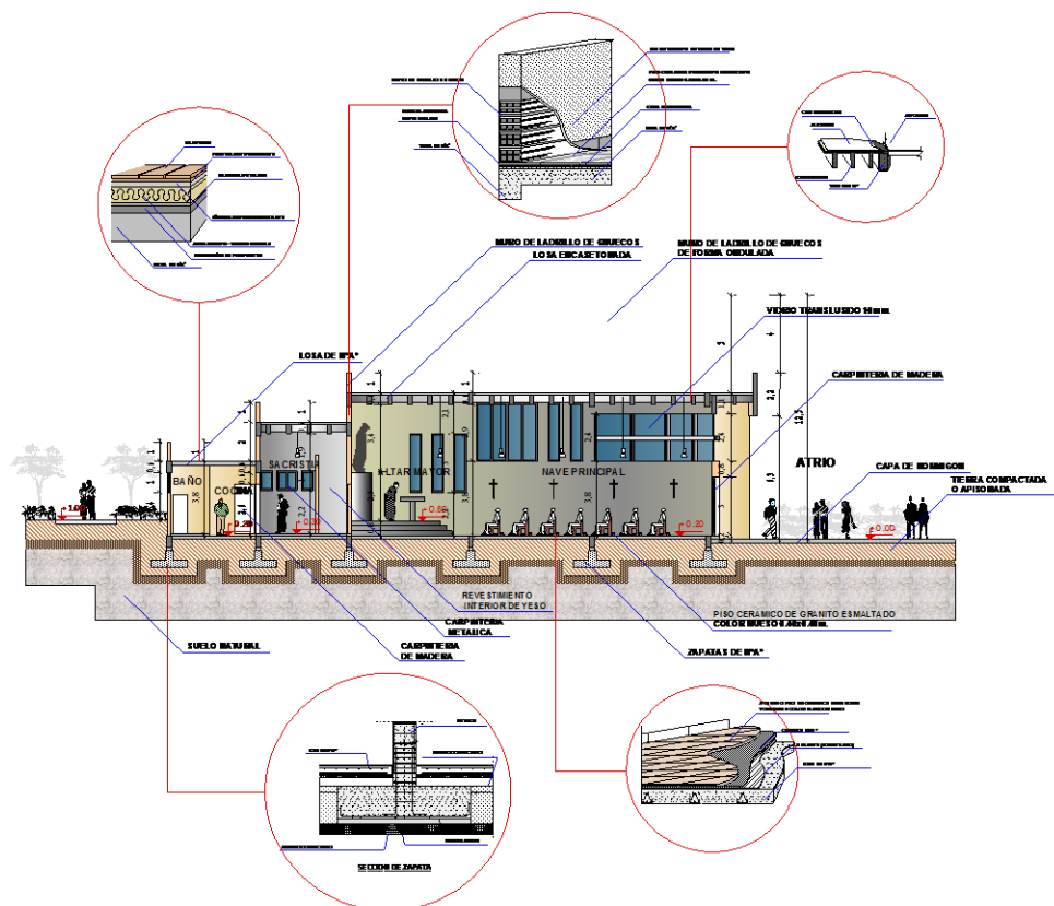
CORTE A-A'
