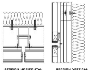
DETALLE DE PERFIL DE ACERO
