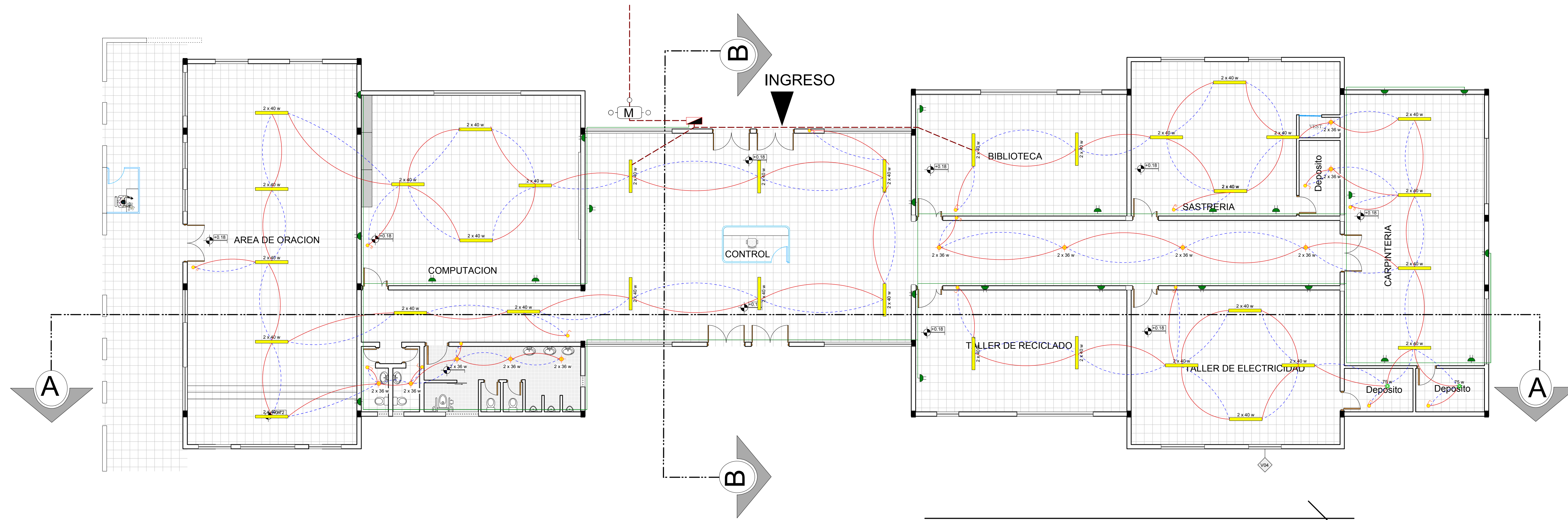
PLANO DE INSTALACION ELECTRICA
