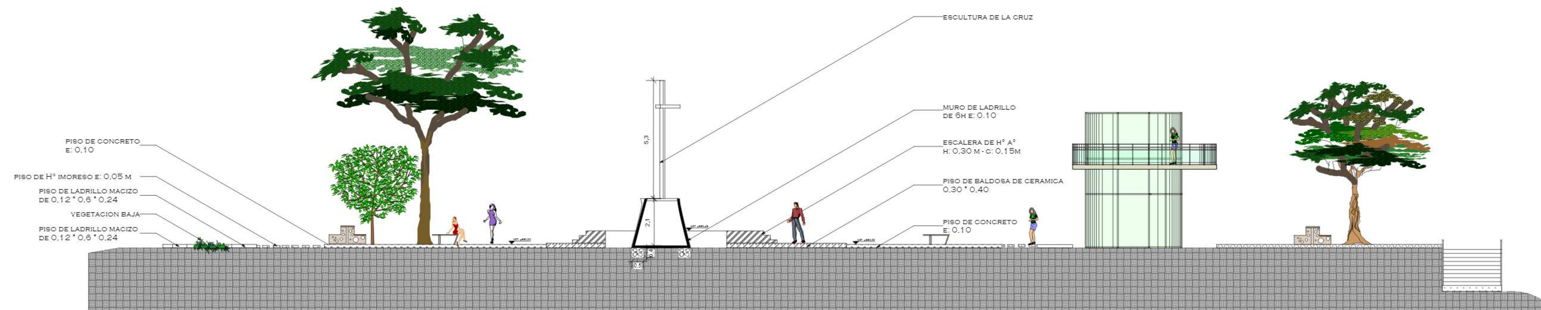
CORTE LONGITUDINAL "A- A"
