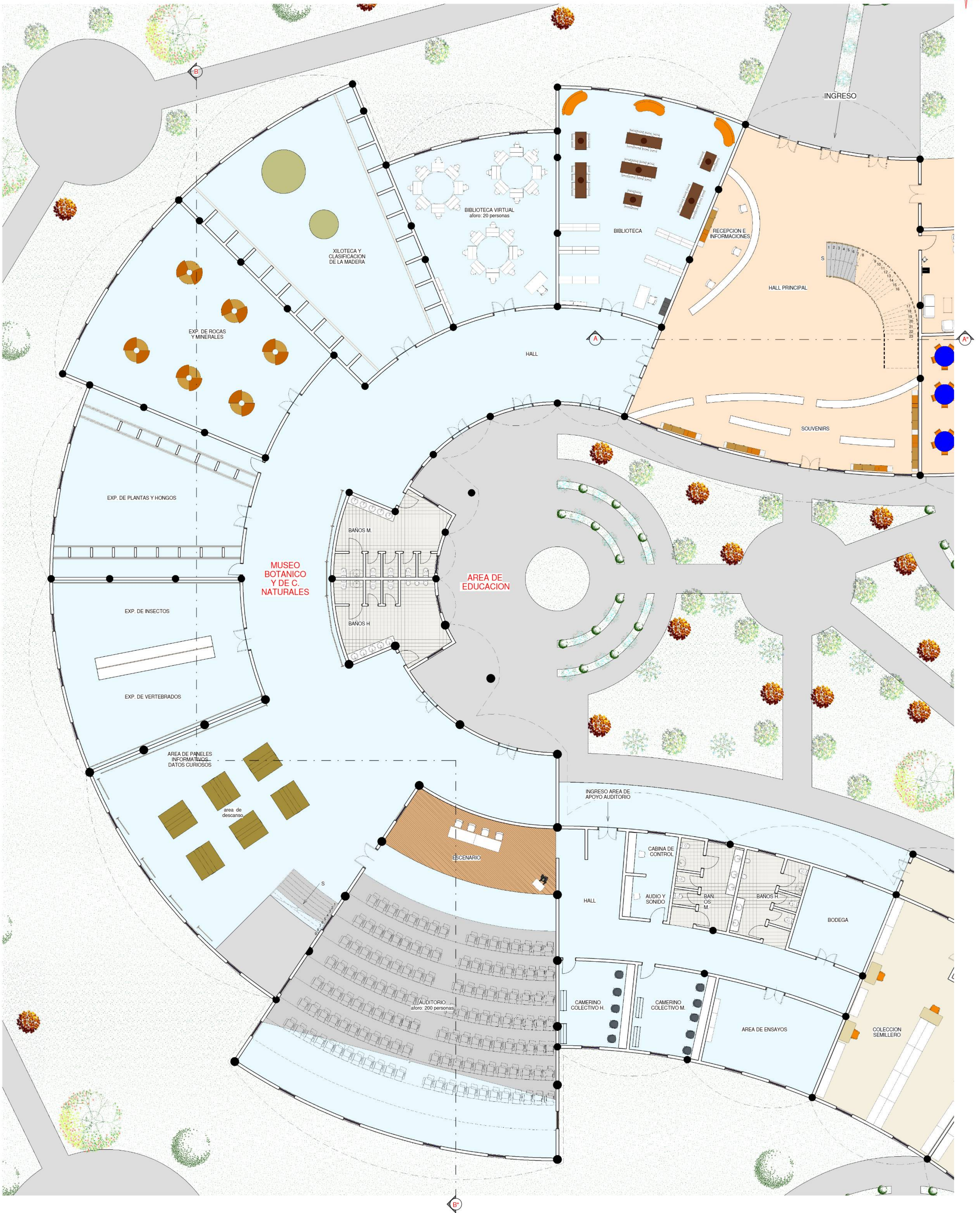
PLANTA BAJA AMOBLADA BLOQUE EDUCACION ESC..... 1:100
