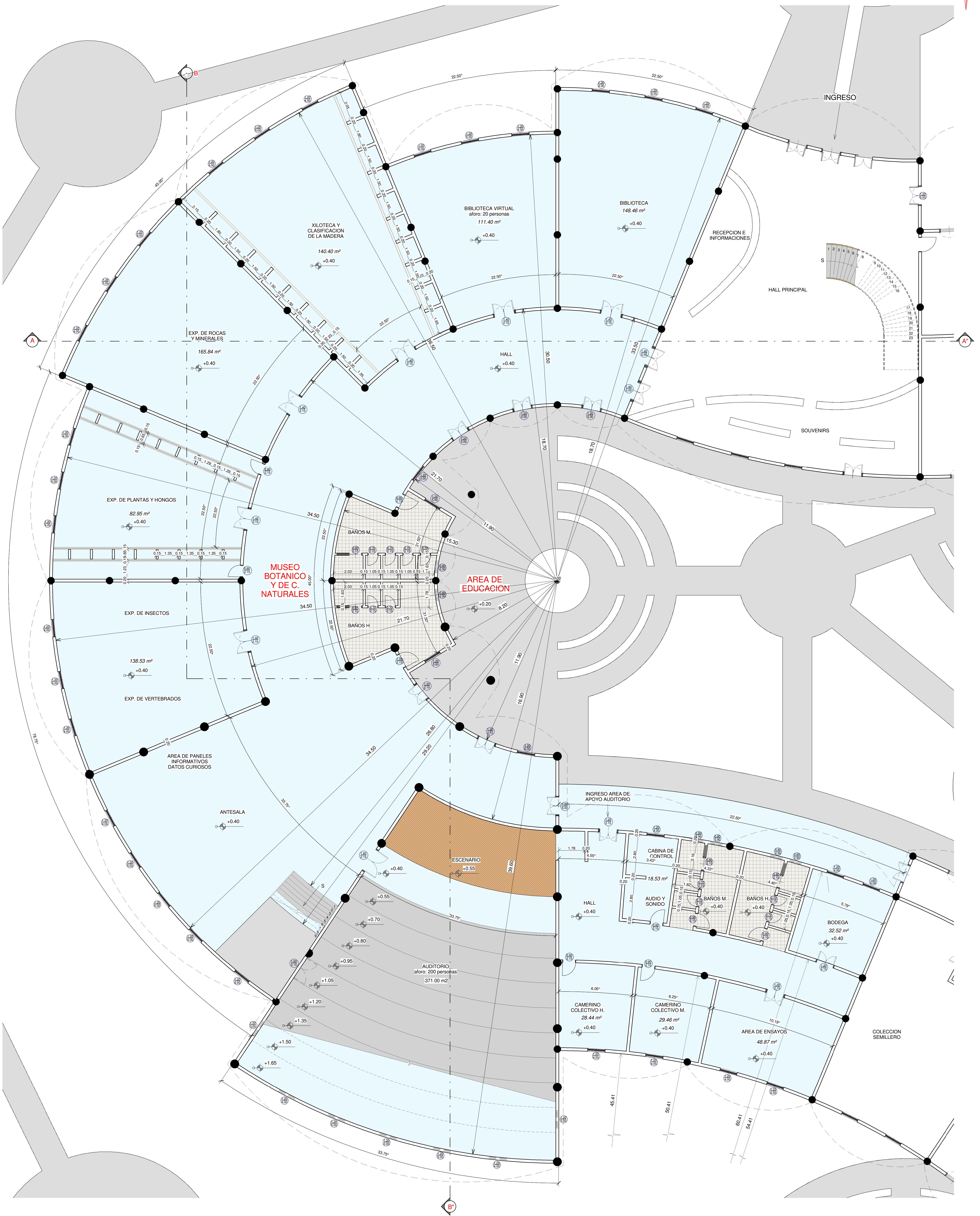
PLANTA BAJA ACOTADA BLOQUE EDUCACION ESC.....1:100
