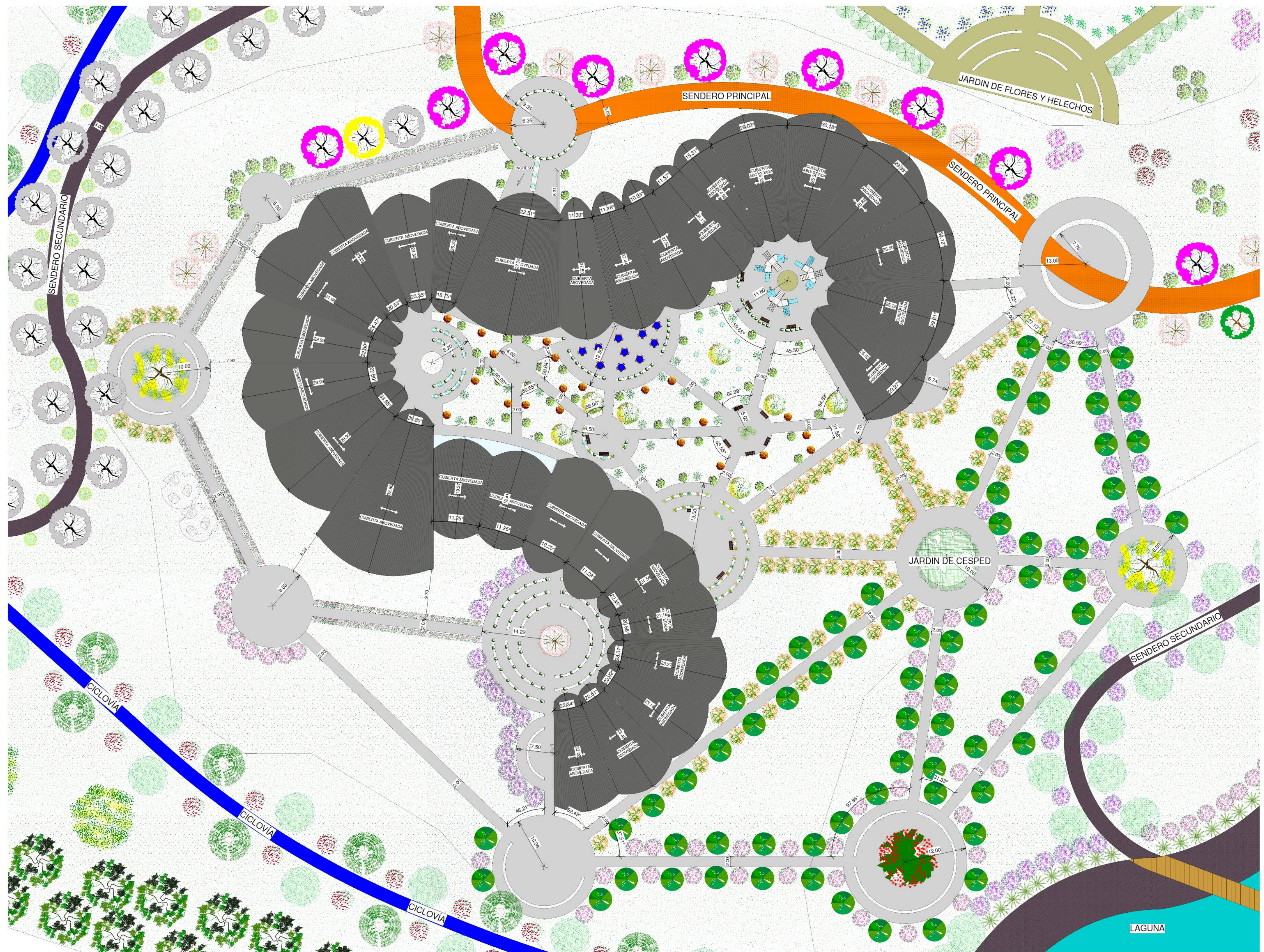
PLANO DE SITIO Y TECHOS ESC..... 1:300
