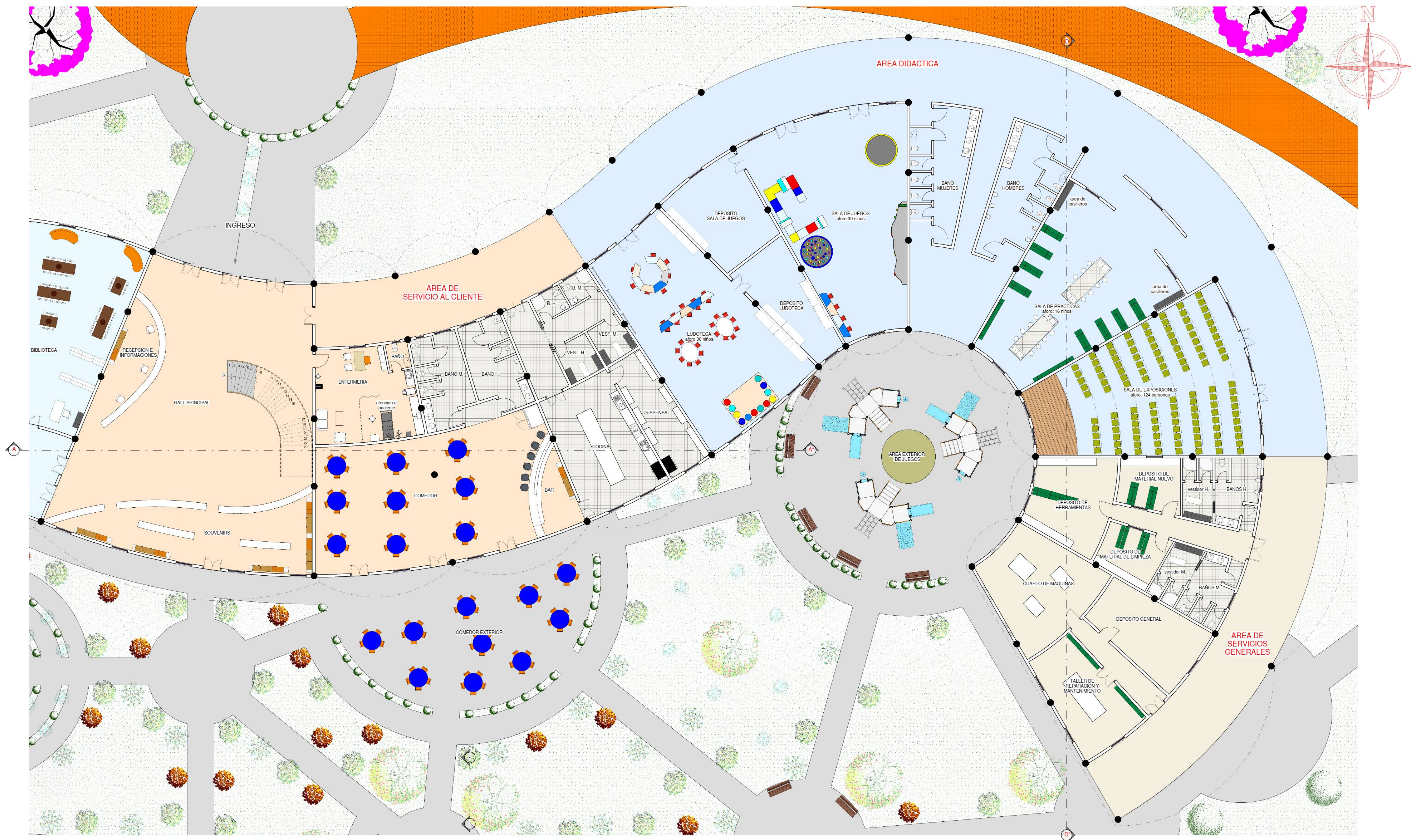
PLANTA BAJA AMOBLADA BLOQUE AREA DIDACTICA ESC.....1:100
