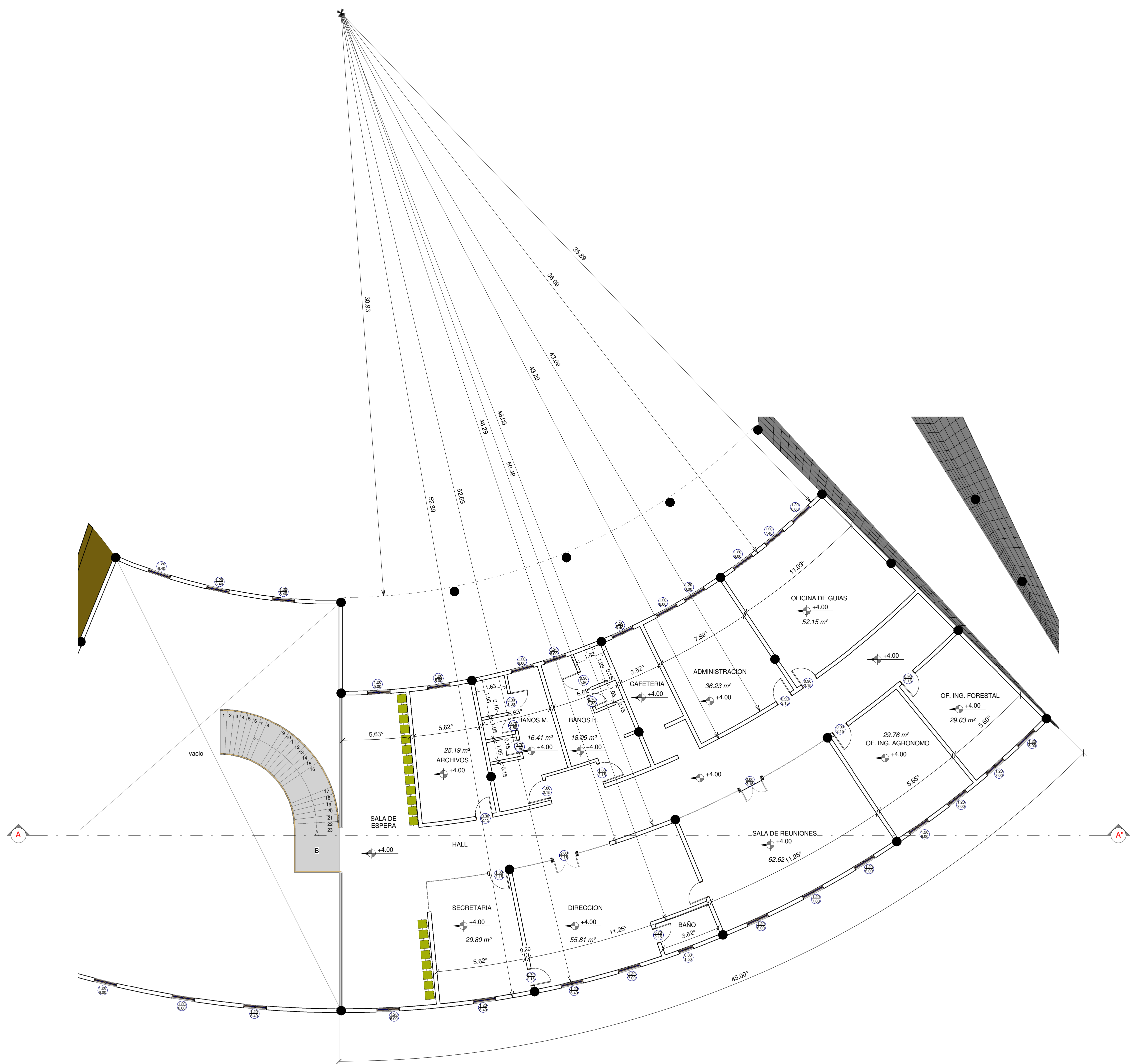
PLANTA ALTA ACOTADA ESC..... 1:100
