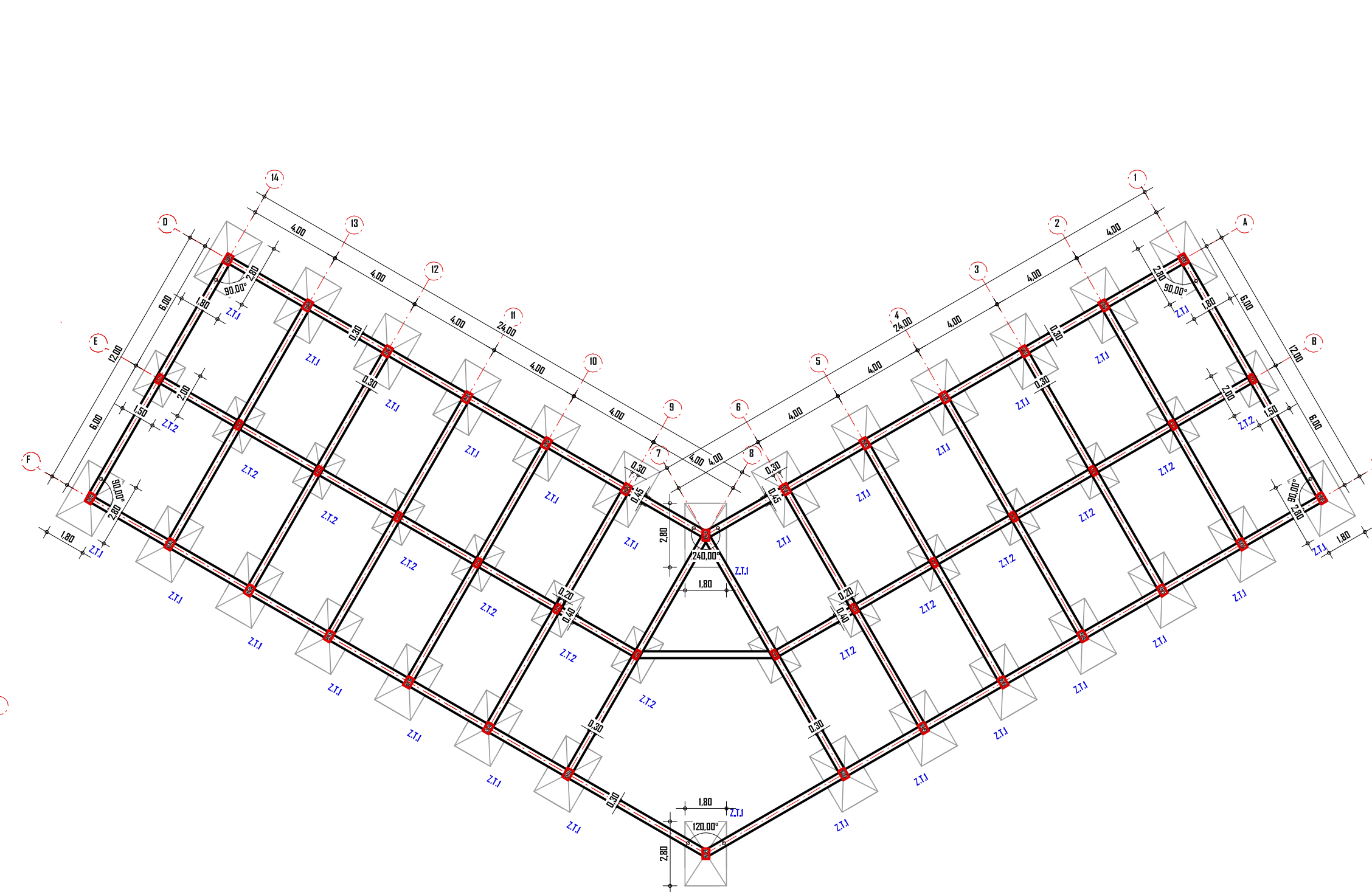
PLANO DE FUNDACIONES - BLOQUE DE MANTENIMIENTO ESC: 1:200
