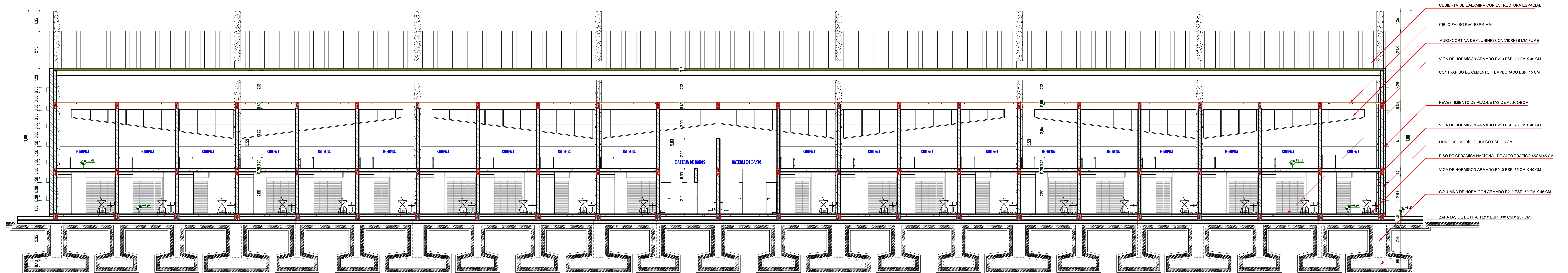
CORTE D' D'' - BLOQUE DE BODEGAS "I" ESC: 1:100
