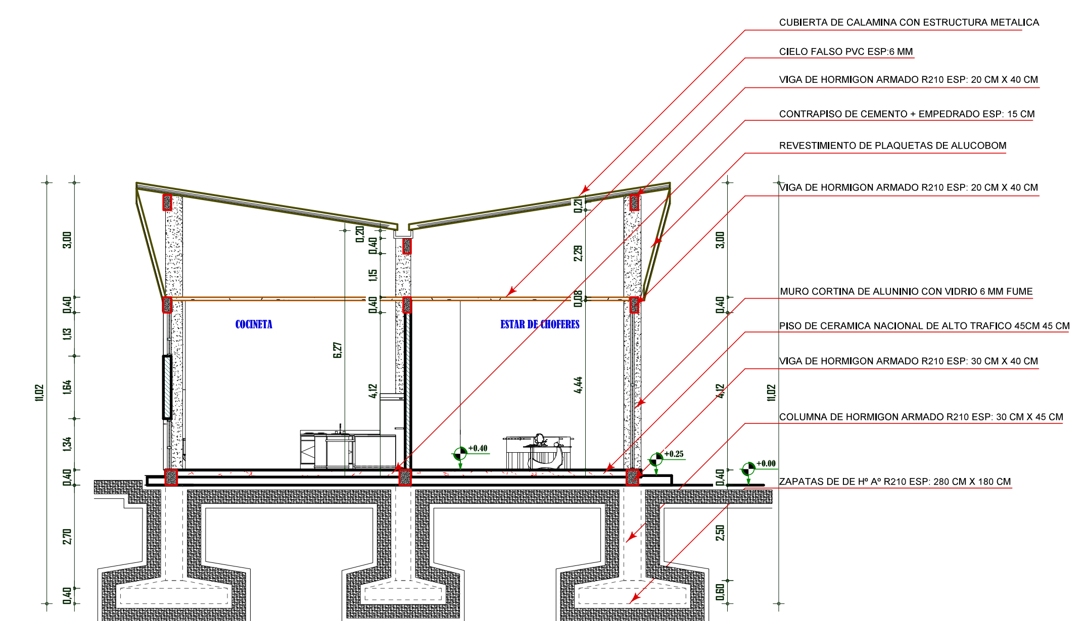
CORTE G' G'' - BLOQUE DE OPERADORES DE BUCES ESC: 1:100
