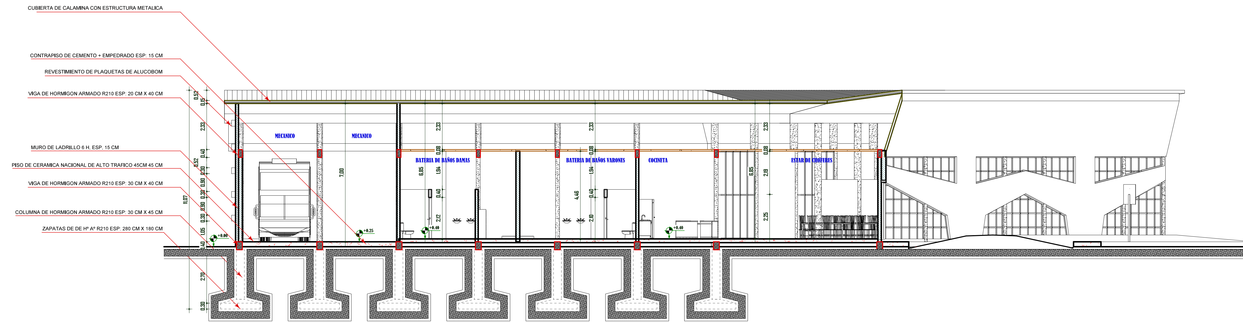
CORTE H' H'' - BLOQUE DE OPERADORES DE BUCES ESC: 1:100
