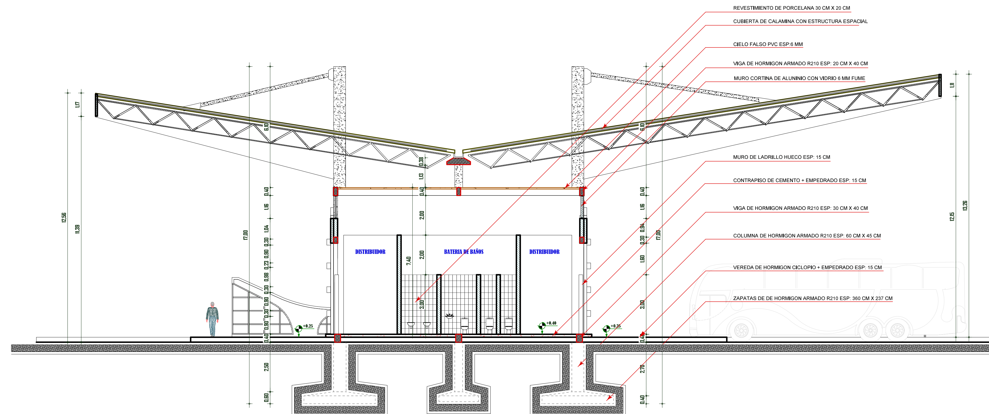
CORTE C' C'' - BLOQUE DE BODEGAS "I" ESC: 1:100
