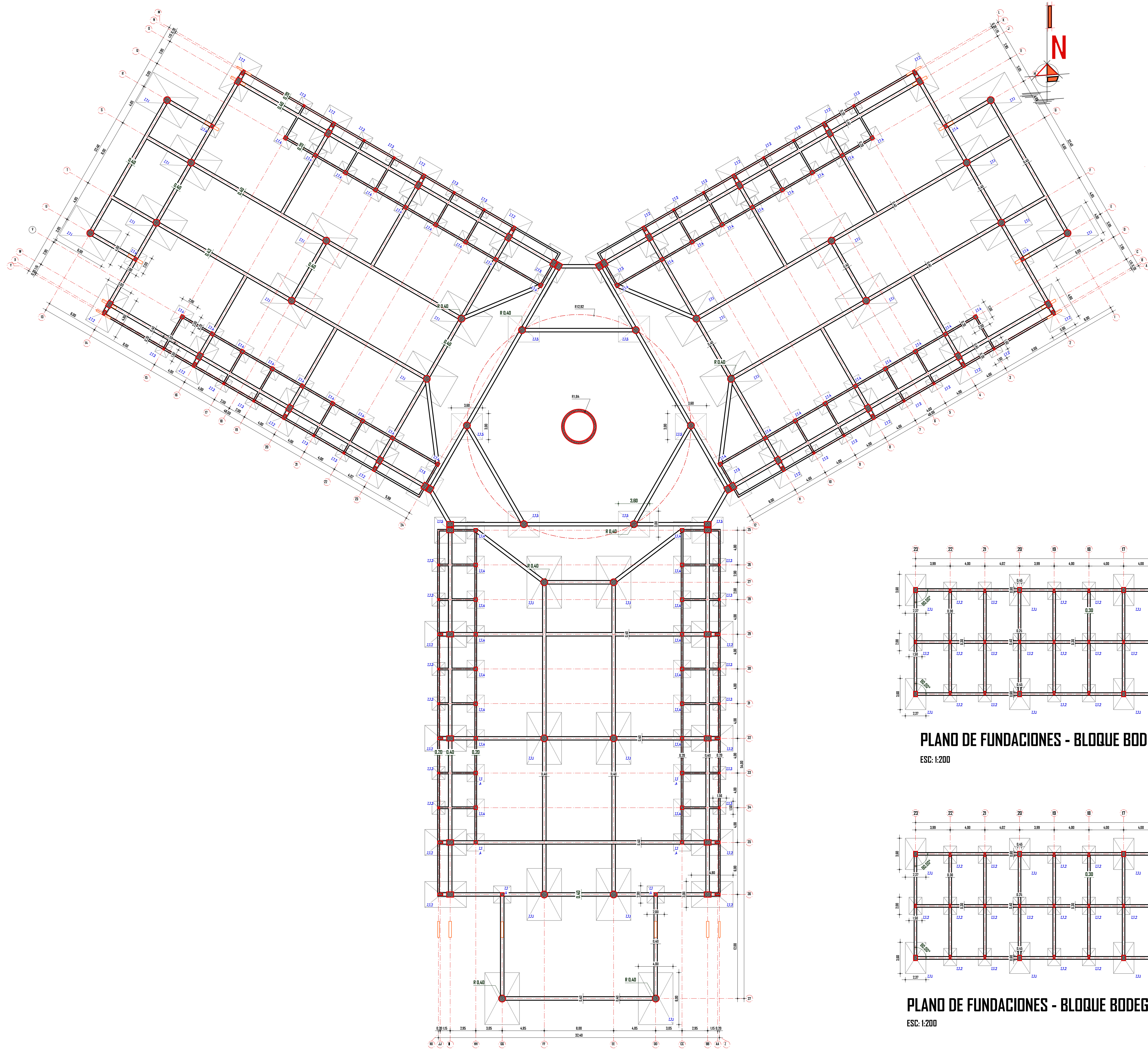
PLANO DE FUNDACIONES - BLOQUE PRINCIPAL ESC: 1:200
