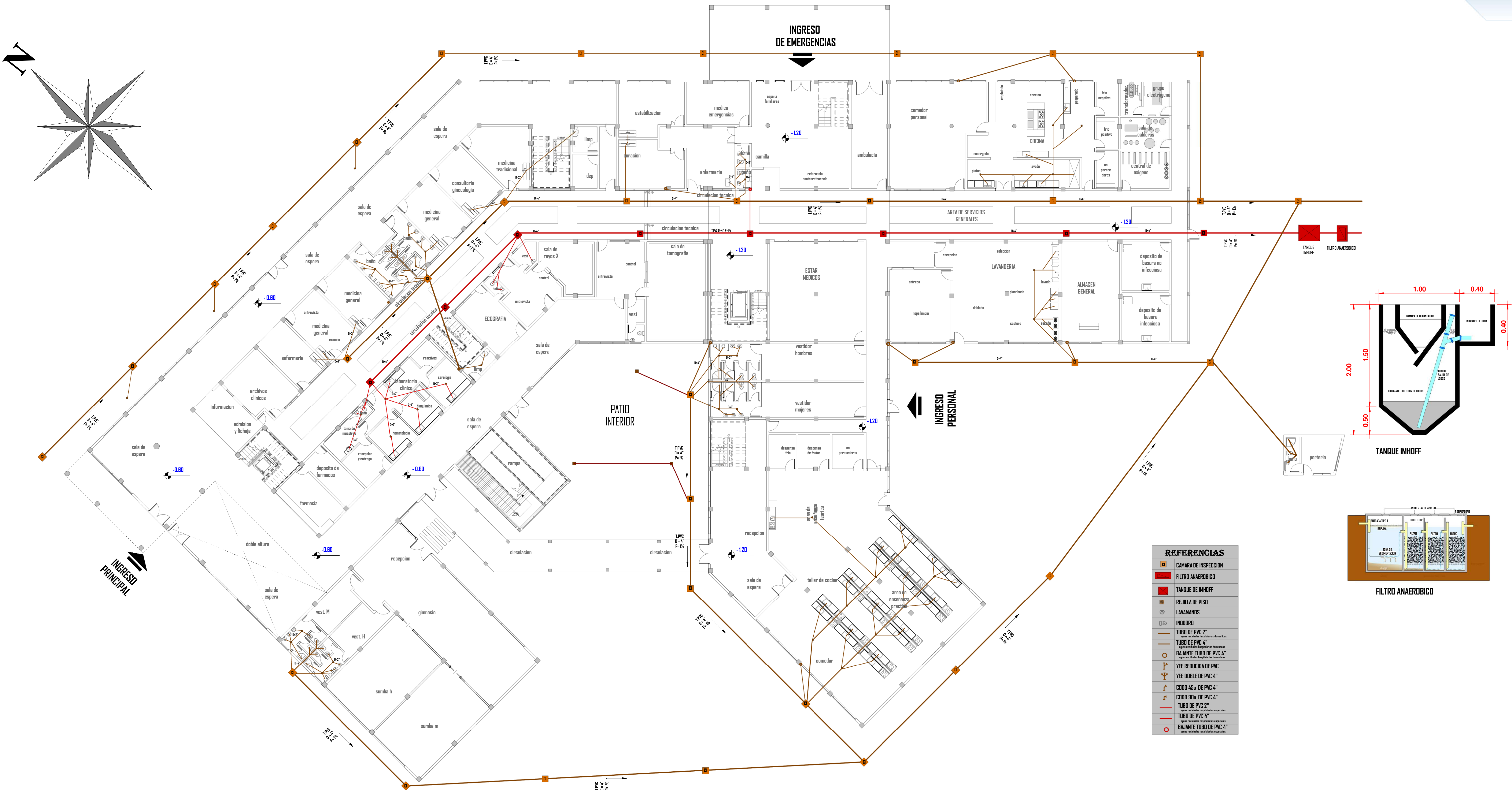
PLANTA BAJA INST. SANITARIA ESC. 1:150
