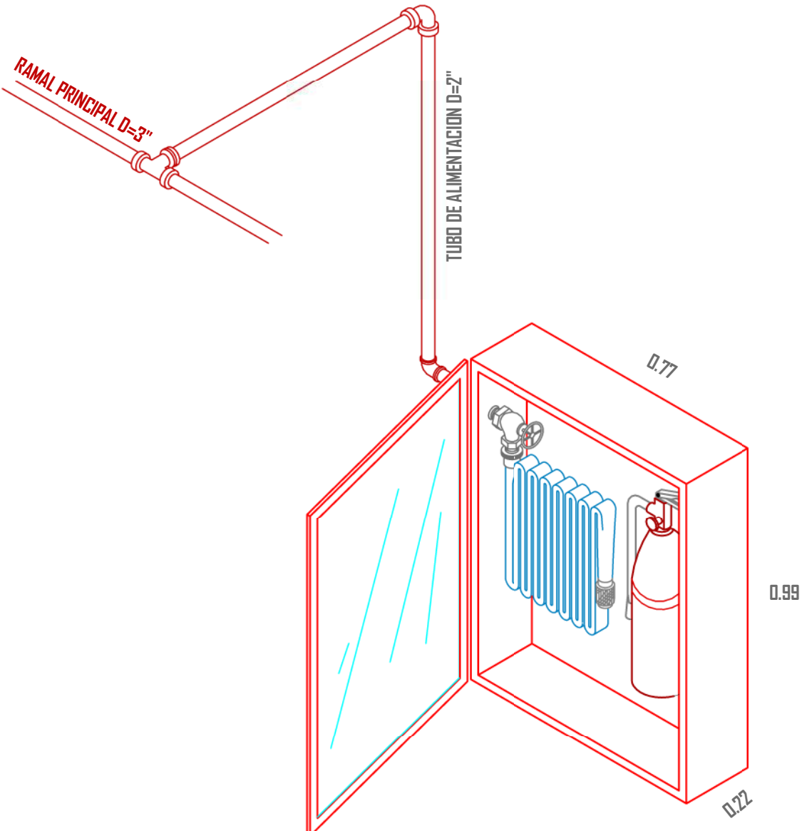
DETALLE DE GABINETE DE PROTECCION CONTRA INCENDIO
