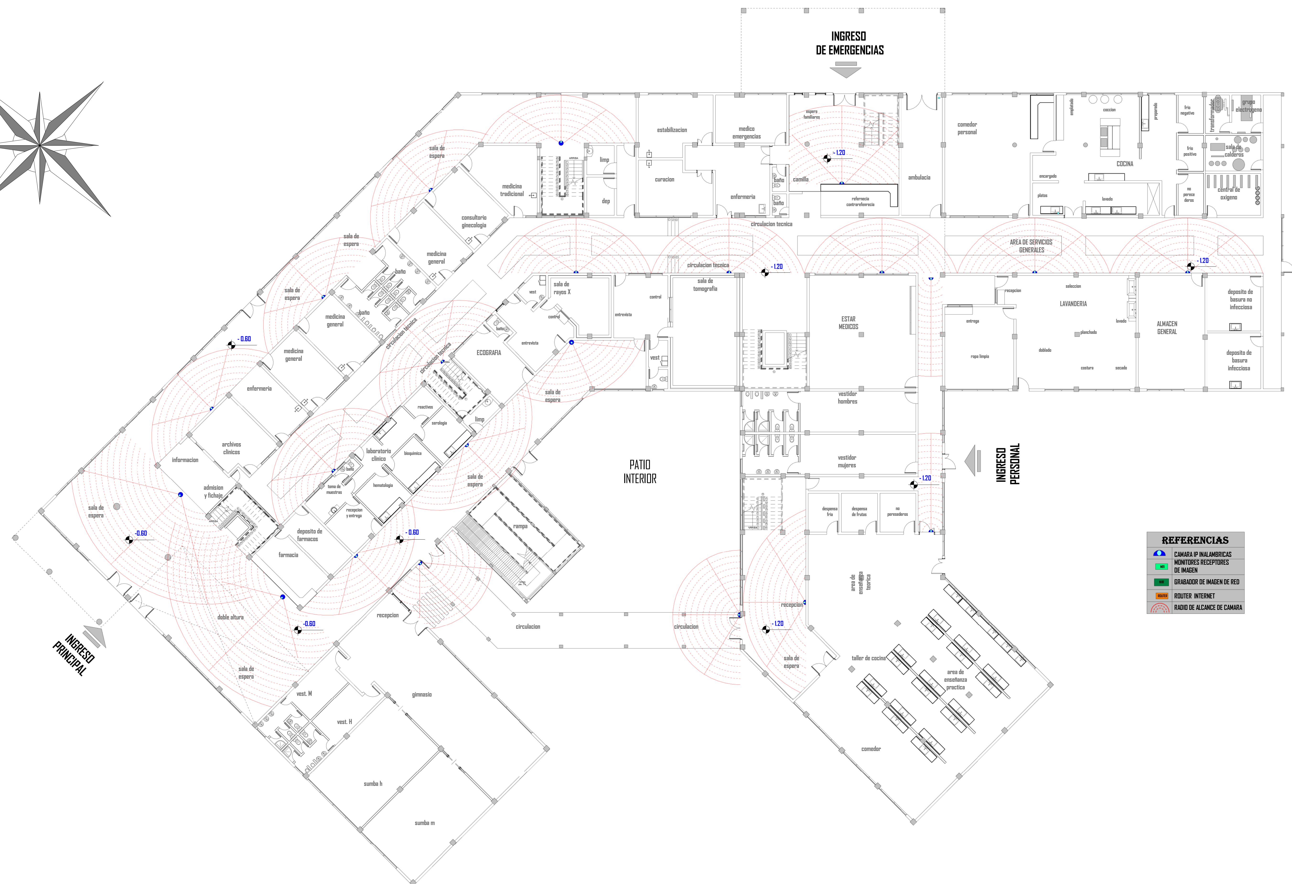
PLANTA BAJA INST. DE SISTEMA DE SEGURIDAD ESC. 1:150
