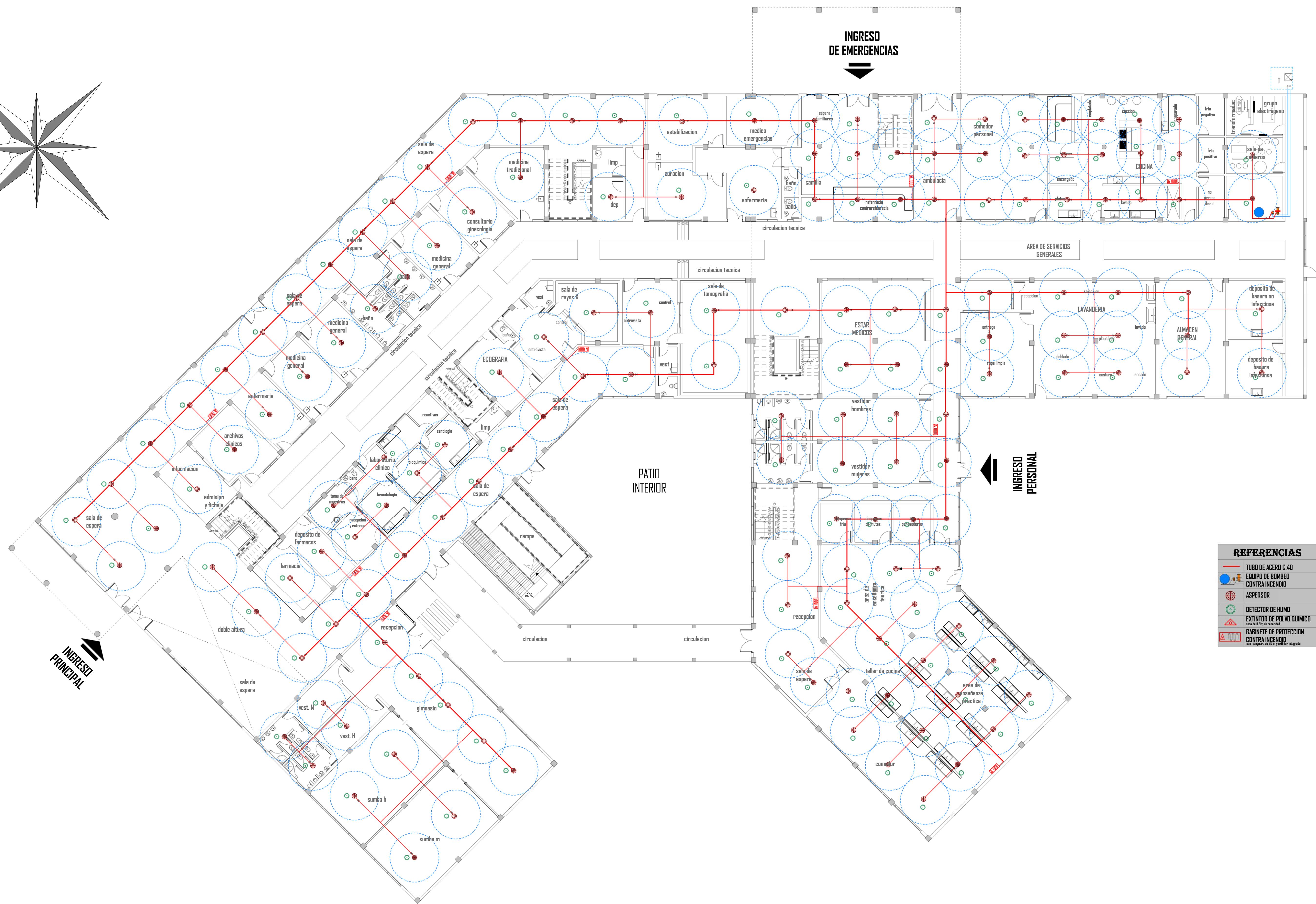
PLANTA BAJA INST. CONTRA INCENDIO ESC. 1:150
