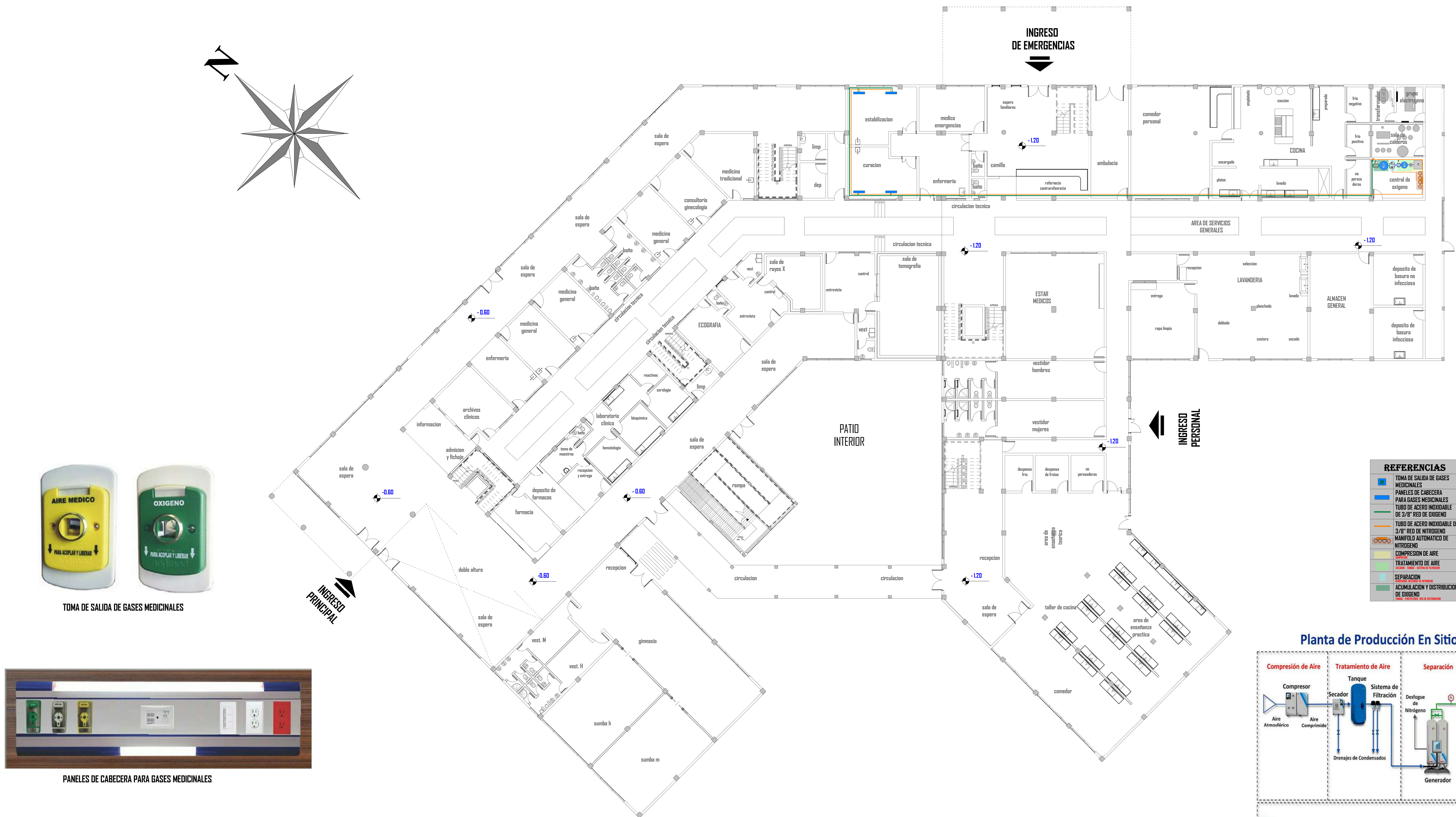
PLANTA BAJA INST. GASES MEDICINALES ESC. 1:150
