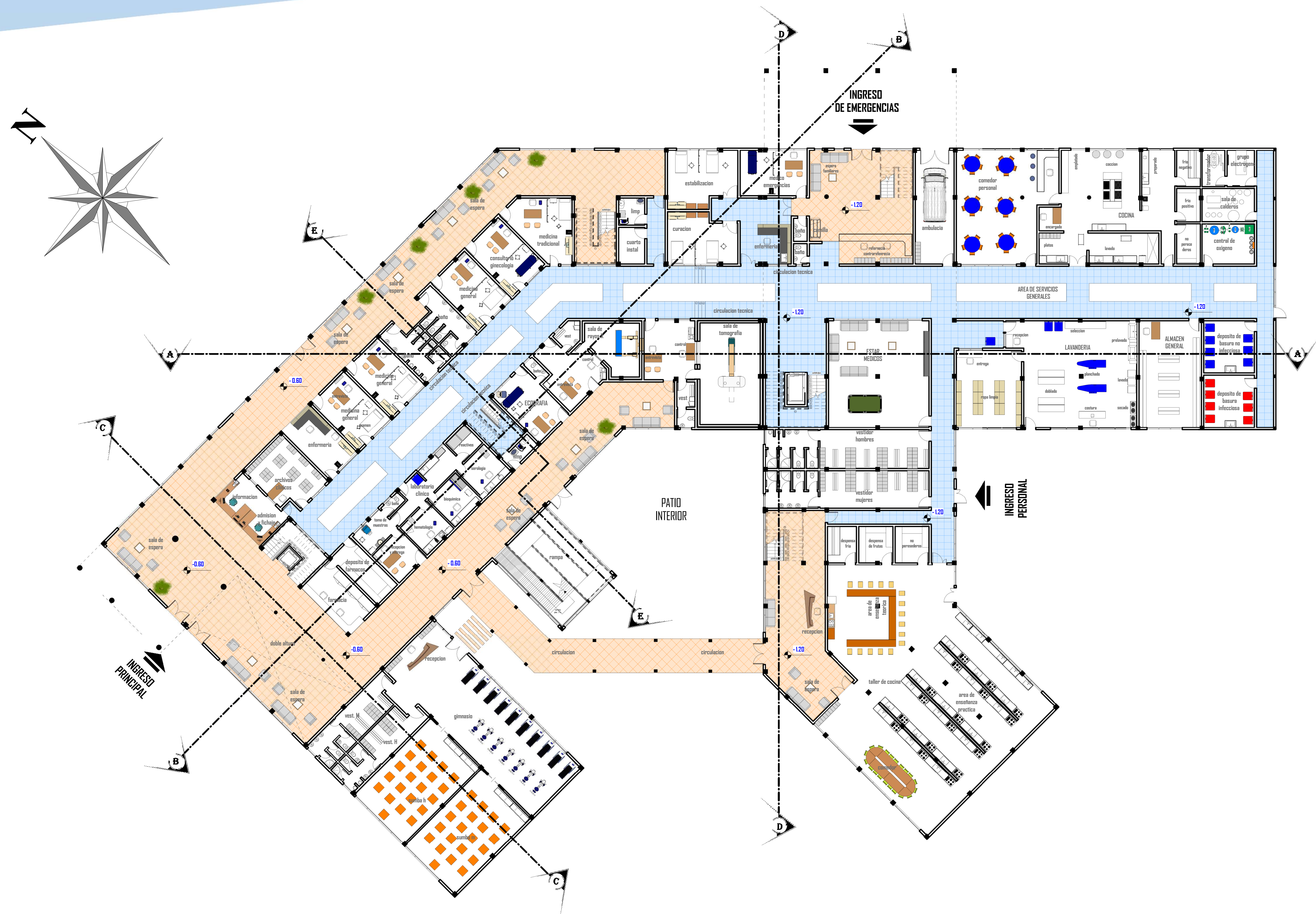
PLANTA BAJA AMOBLADA ESC. 1:150
