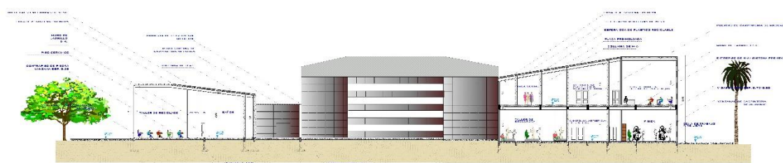
CORTE D-D''
