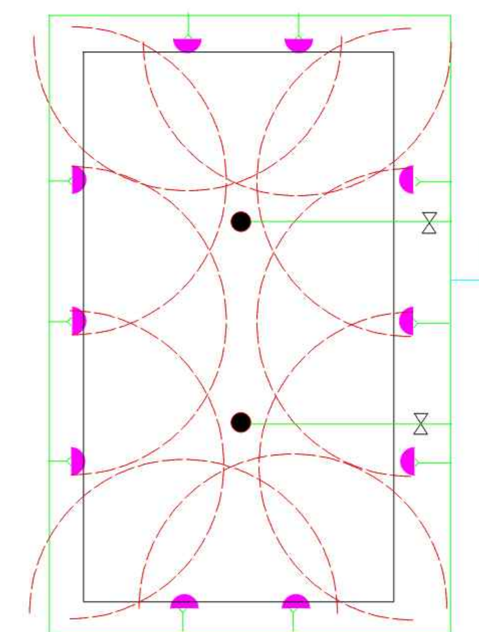
DETALLE DEL FUNCIONAMIENTO DE LOS ASPERSORES
