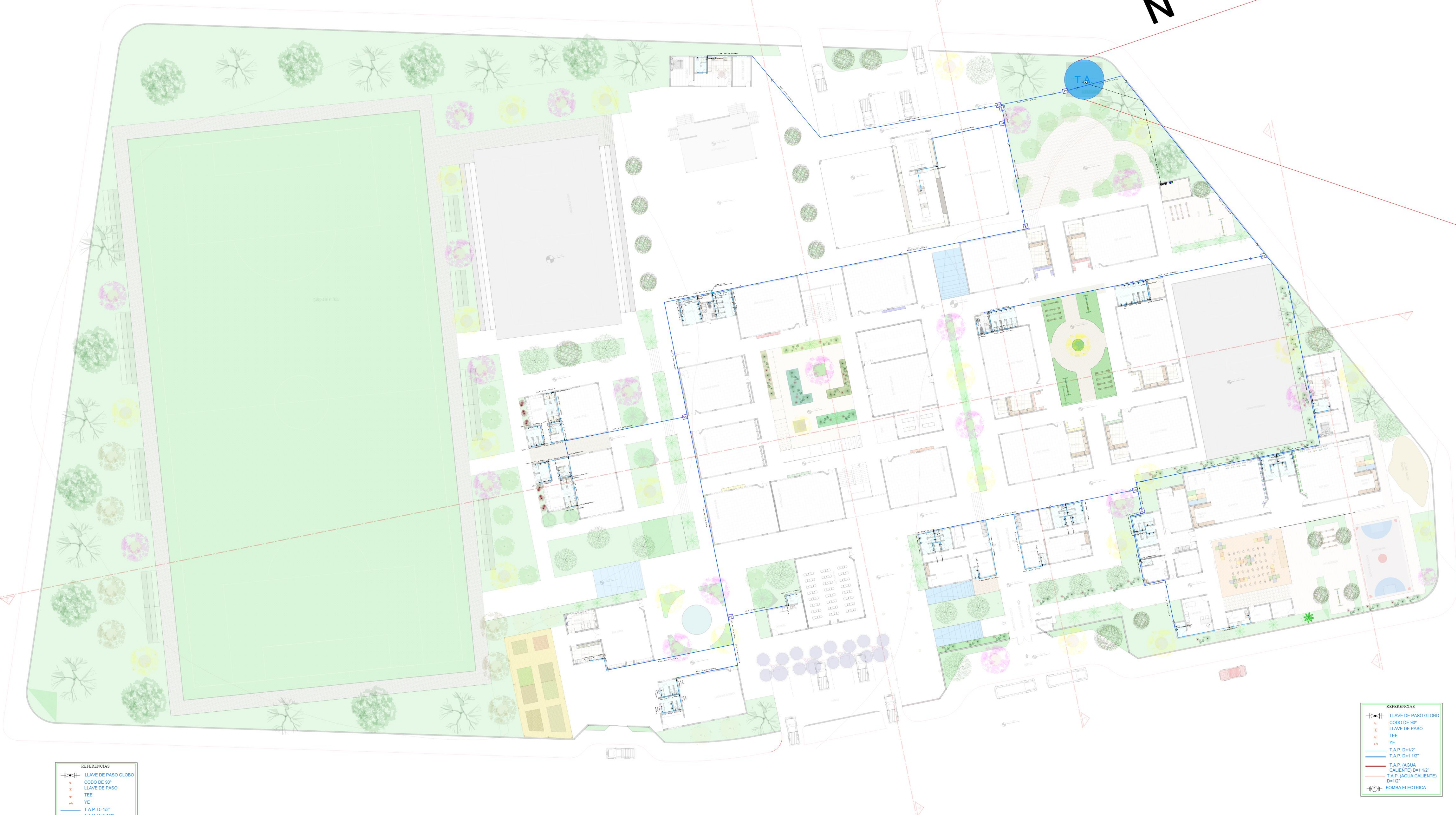
...INSTALACION DE AGUA POTABLE PLANTA BAJA...
