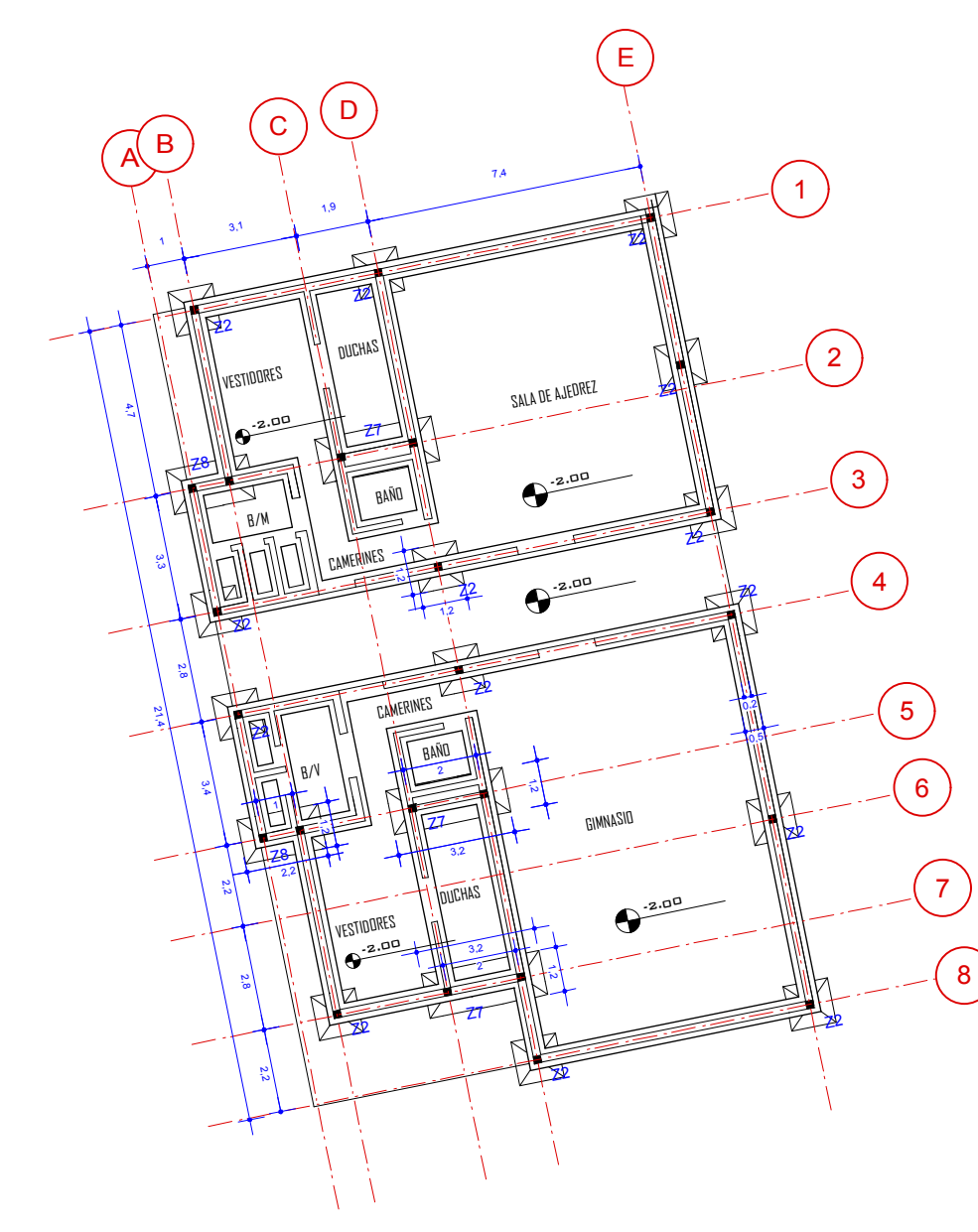
BLOQUE GIMNASIO-SALA DE AJEDREZ.
