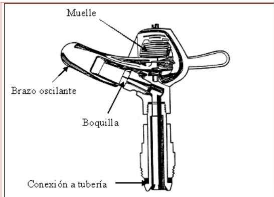
Figura 9.1. Componentes de un aspersor de impacto
