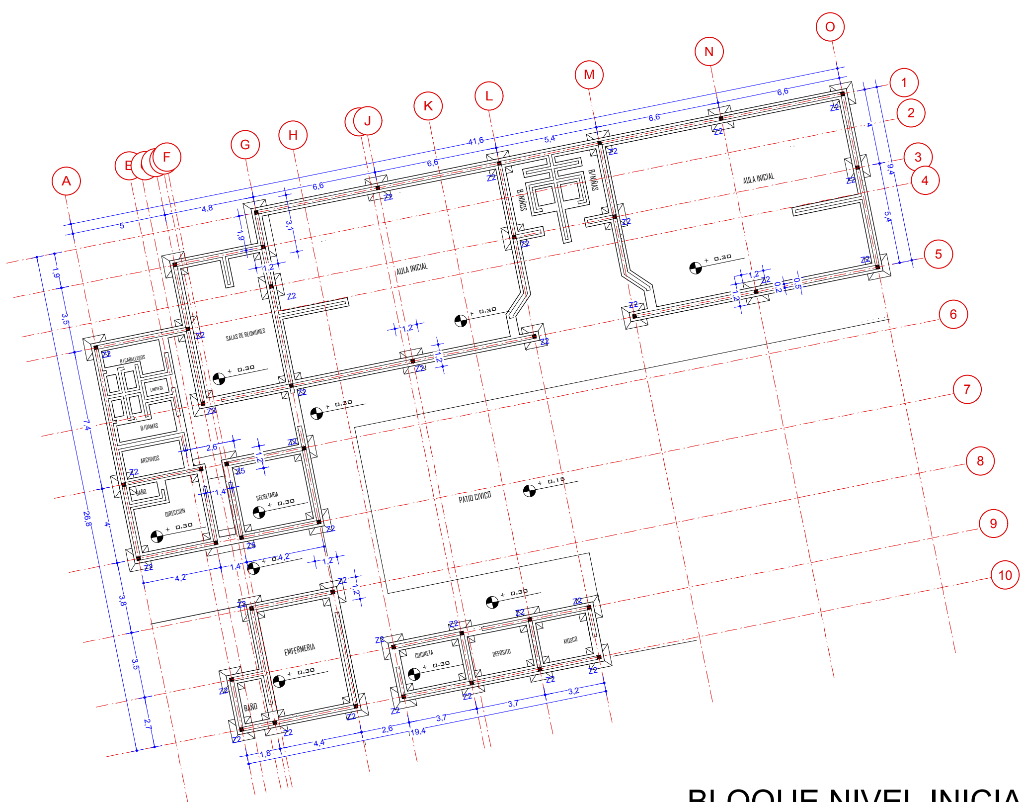
BLOQUE NIVEL INICIAL
