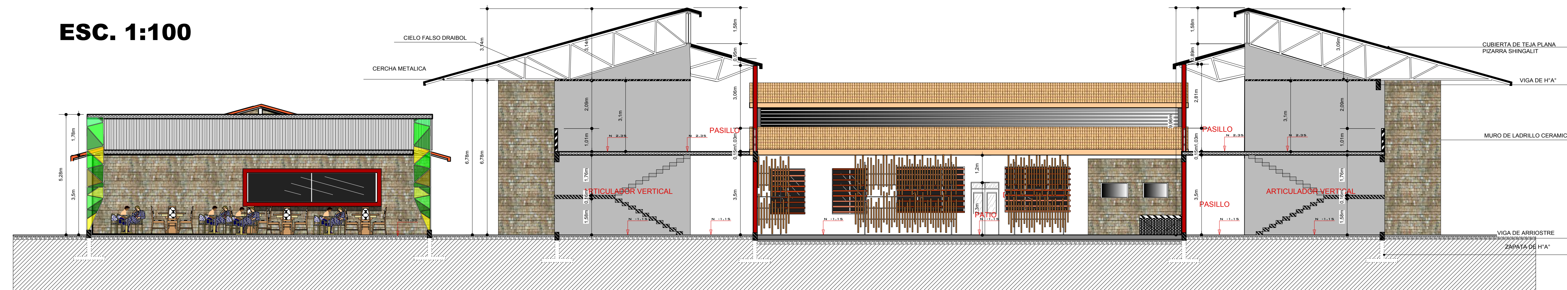
CORTE C - C'
