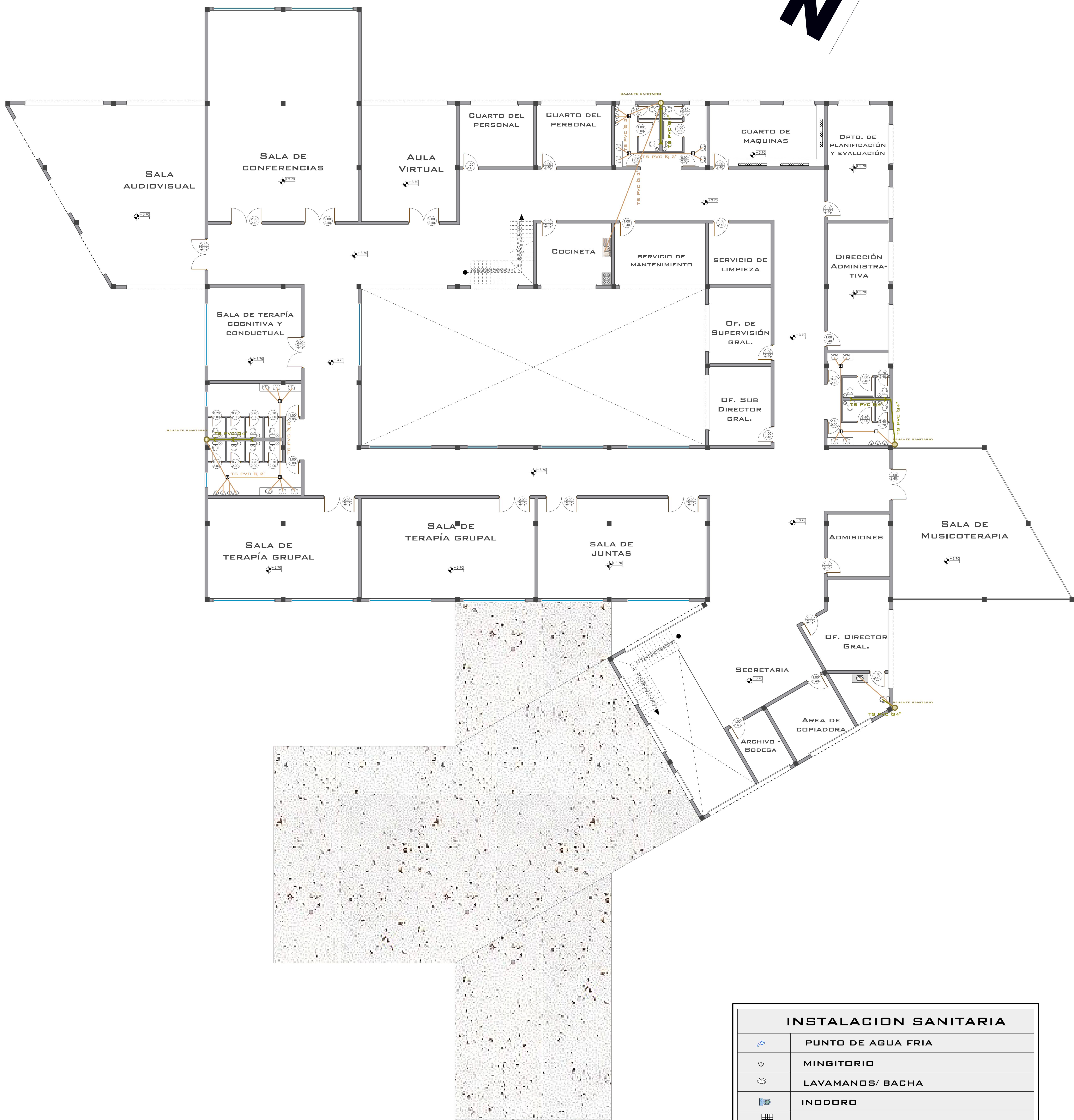
PLANTA ALTA INSTALACIÓN SANITARIA ESCALA 1: 100
