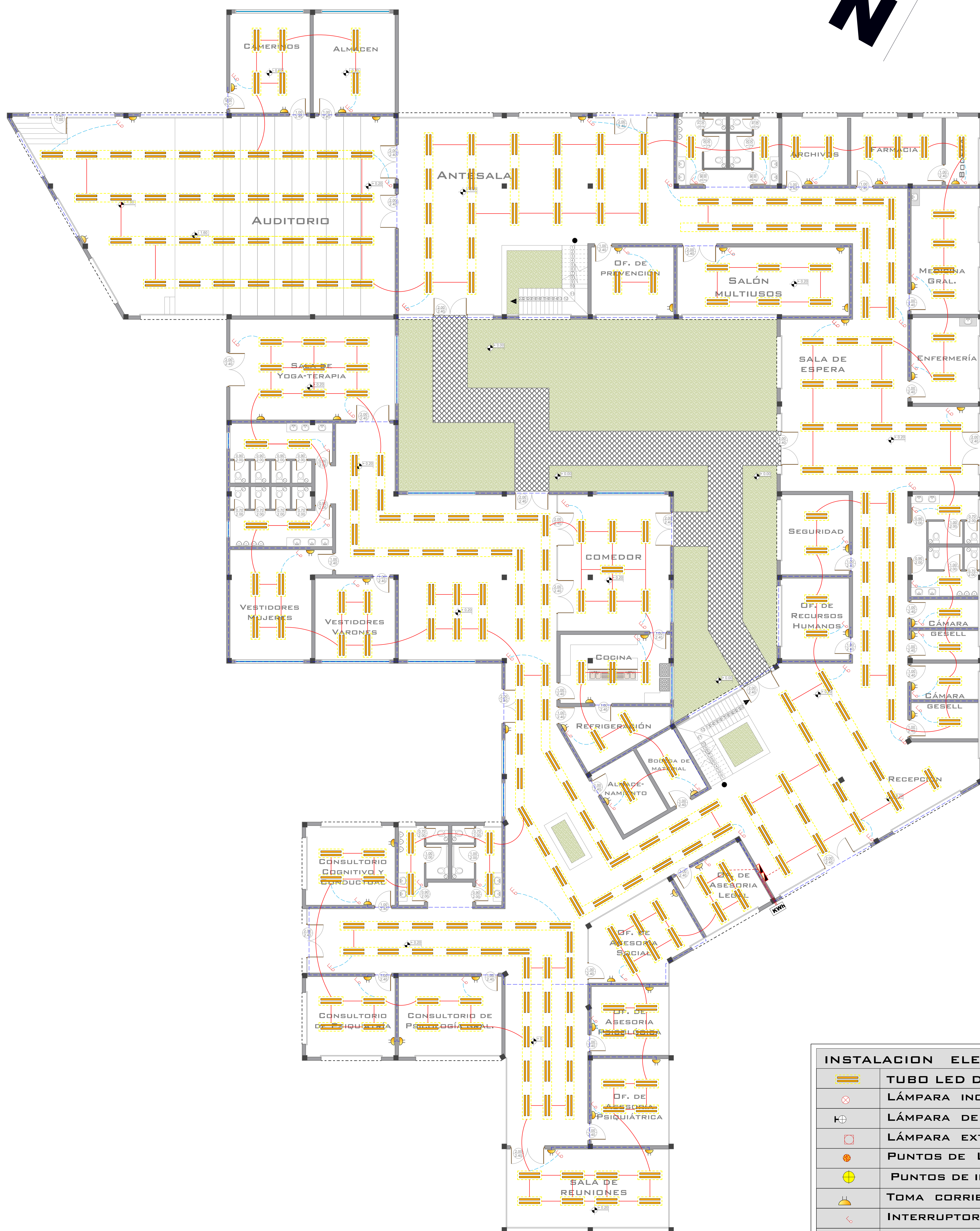
PLANTA BAJA INSTALACIÓN ELÉCTRICA ESCALA 1: 100
