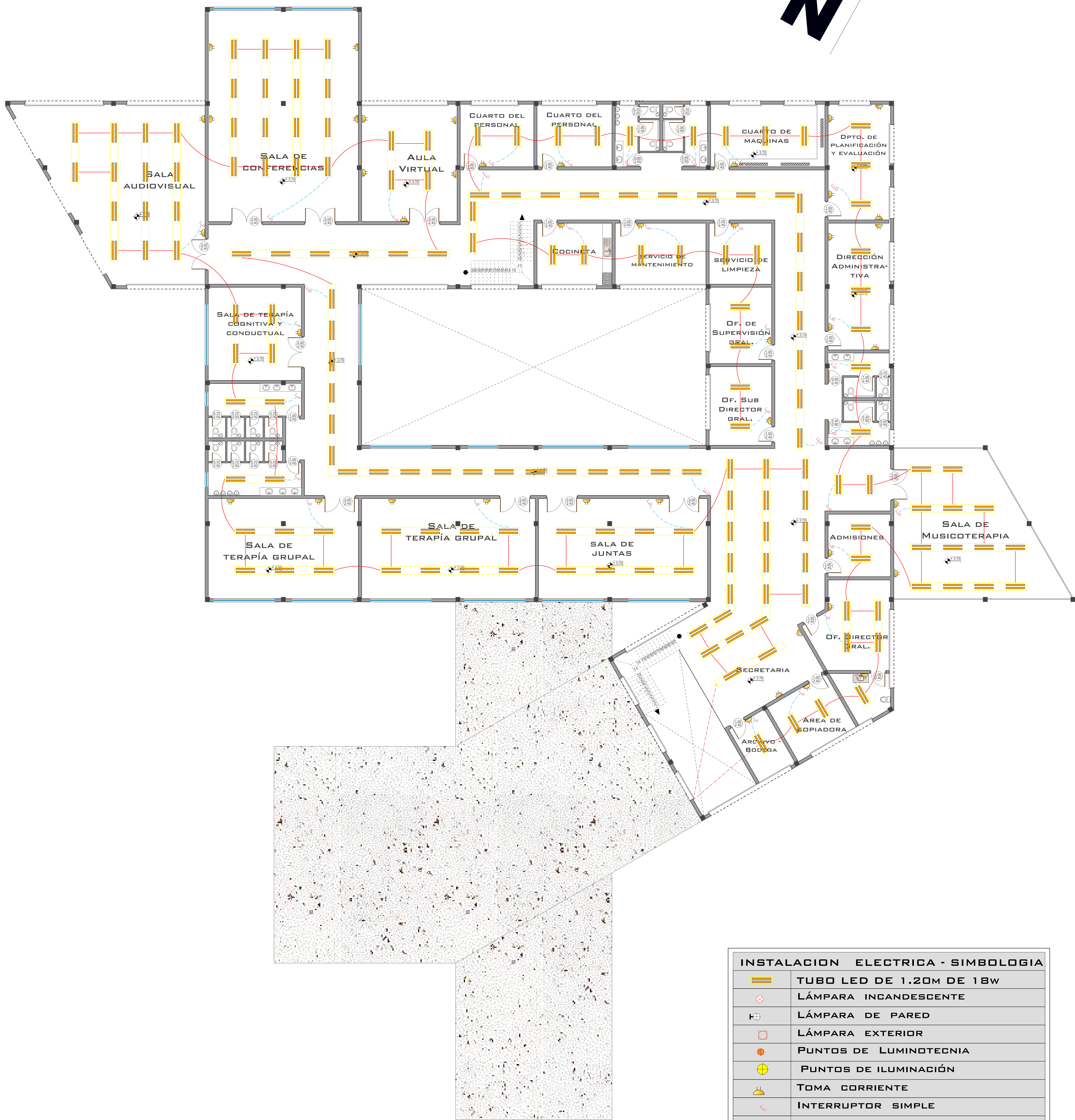
PLANTA ALTA INSTALACIÓN ELÉCTRICA ESCALA 1: 100
