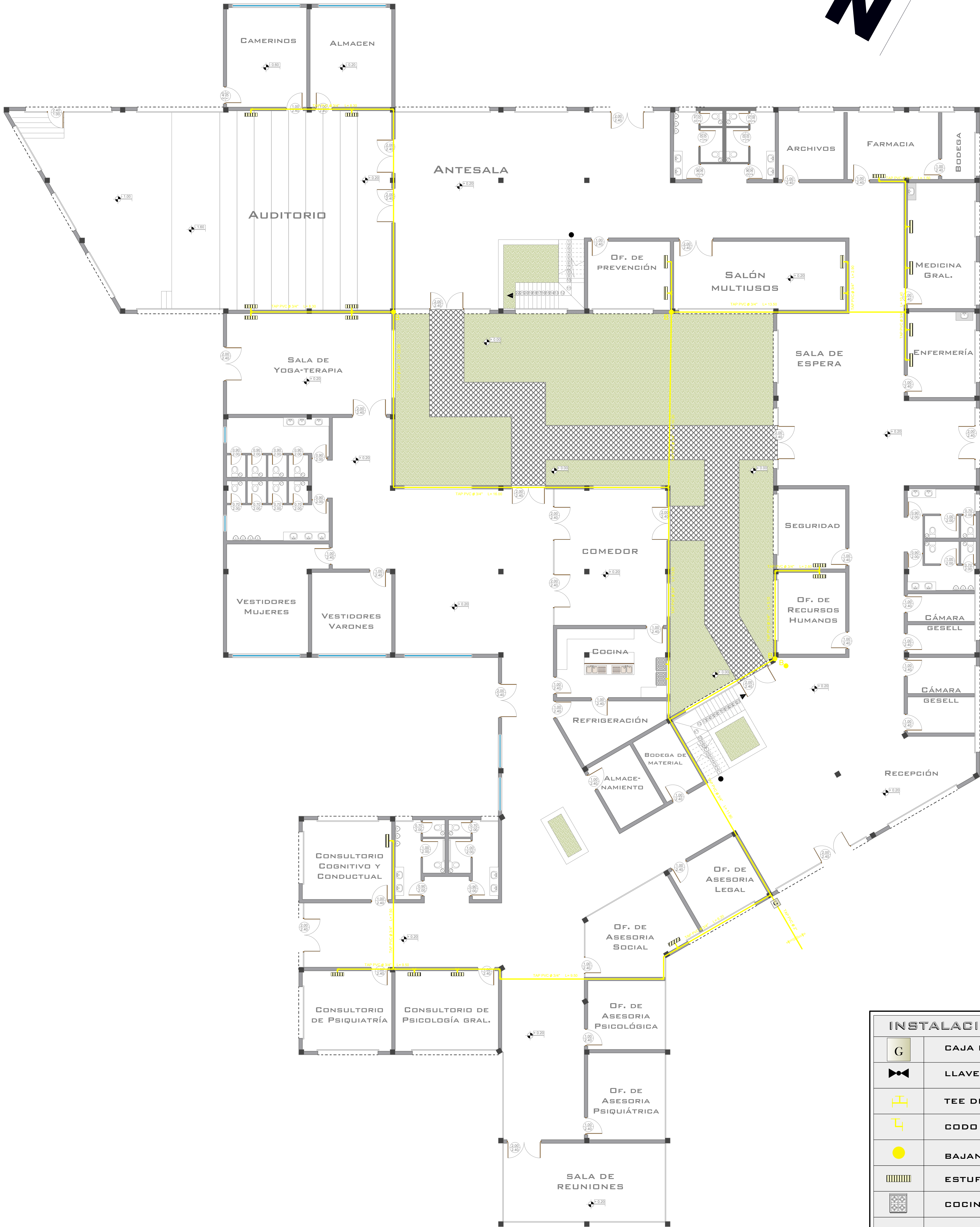
PLANTA BAJA INSTALACIÓN DE GAS ESCALA 1: 100
