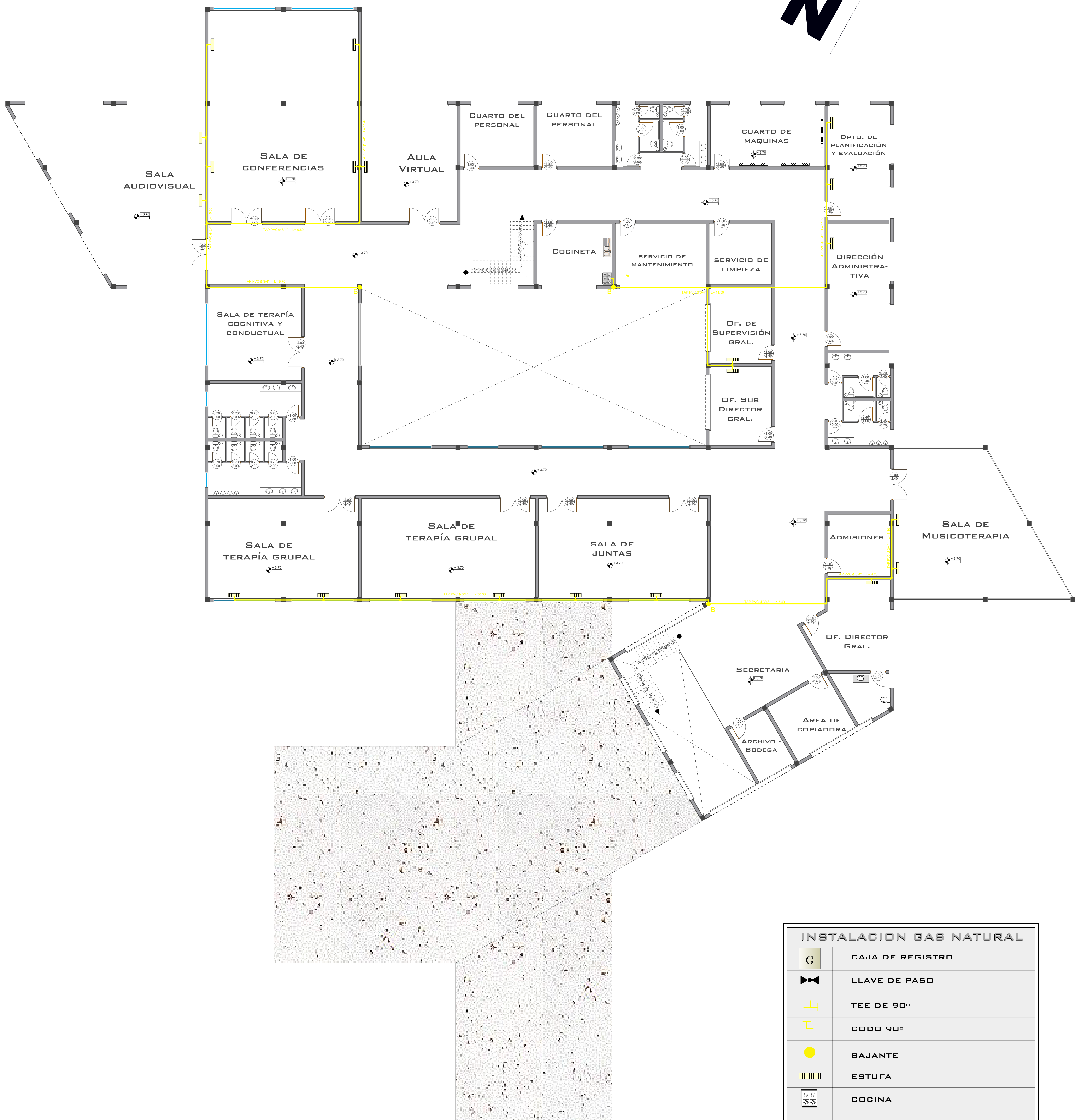
PLANTA ALTA INSTALACIÓN DE GAS ESCALA 1: 100
