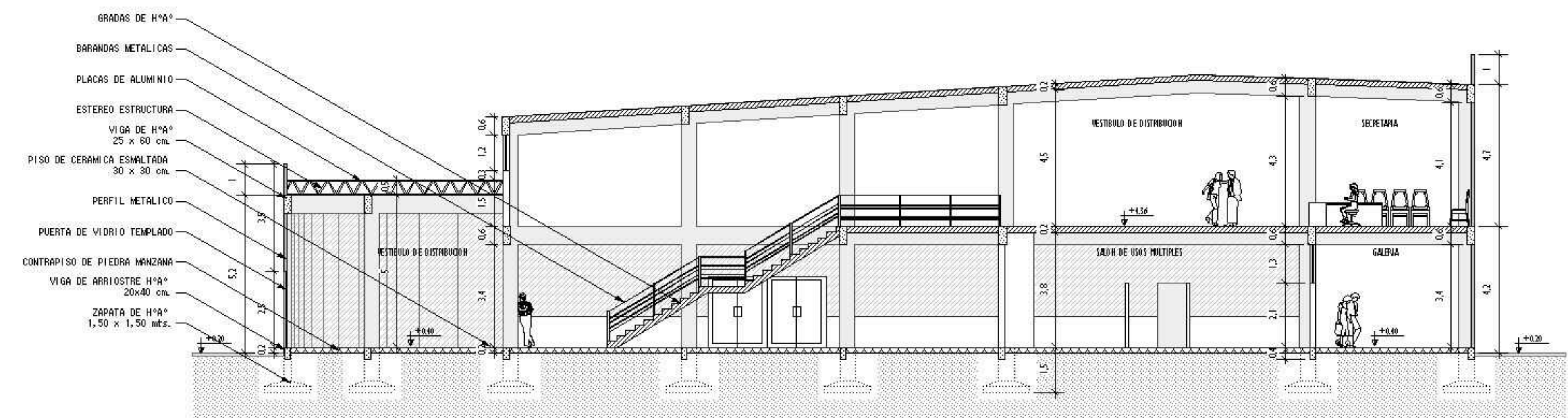
CORTE B-B
