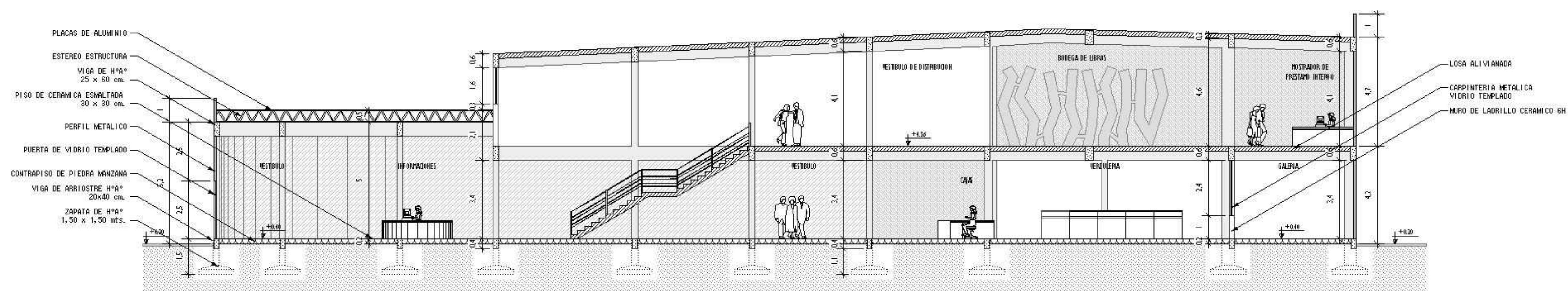
CORTE D-D
