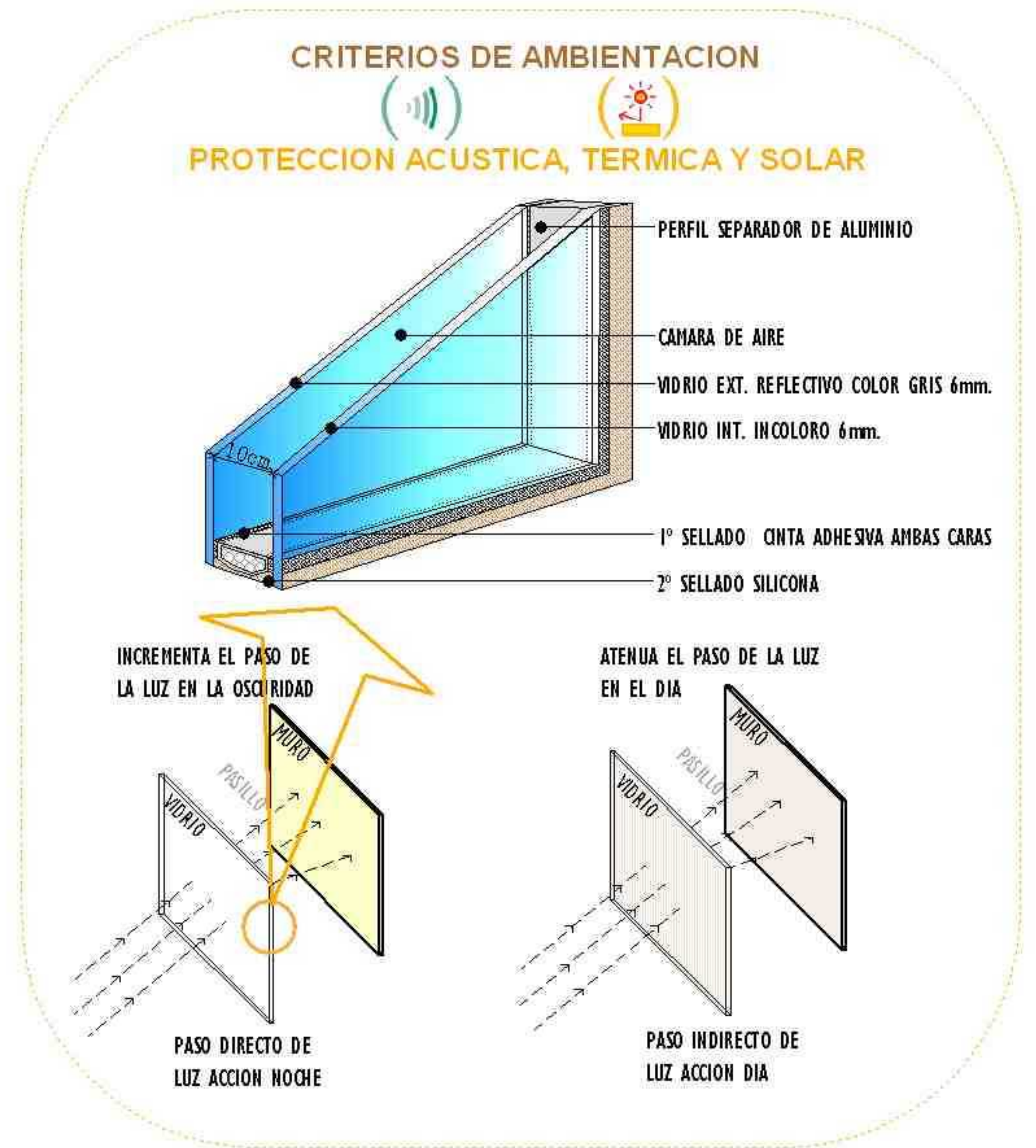
FACHADA CORTINA
