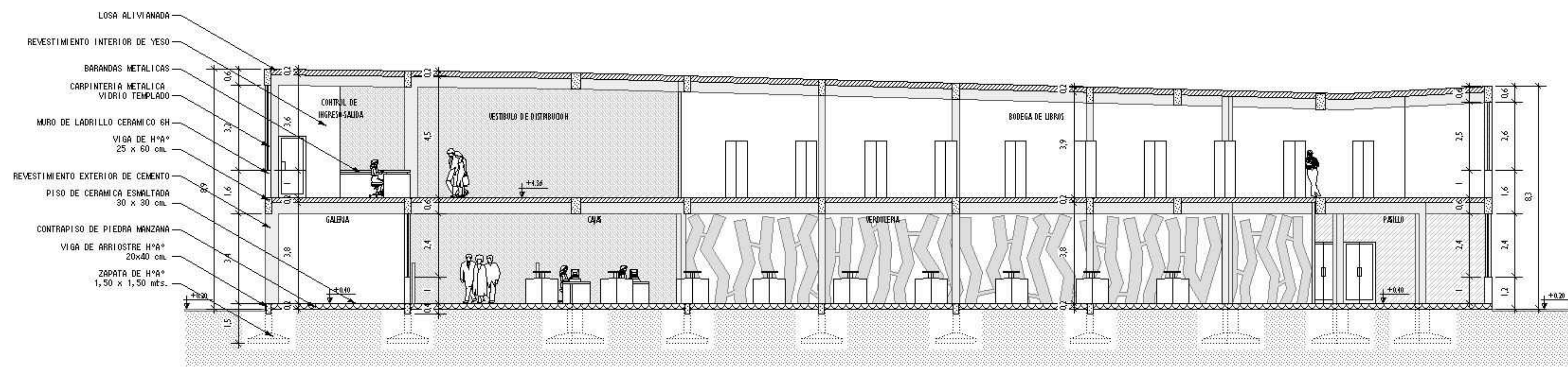
CORTE C-C
