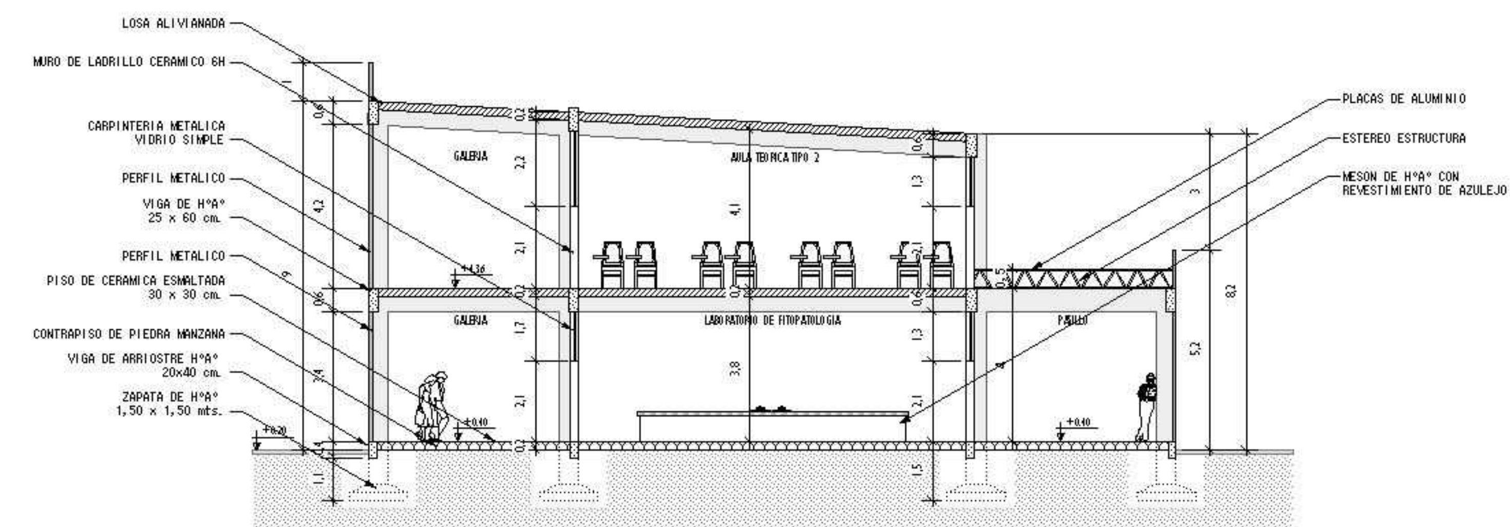
CORTE E-E
