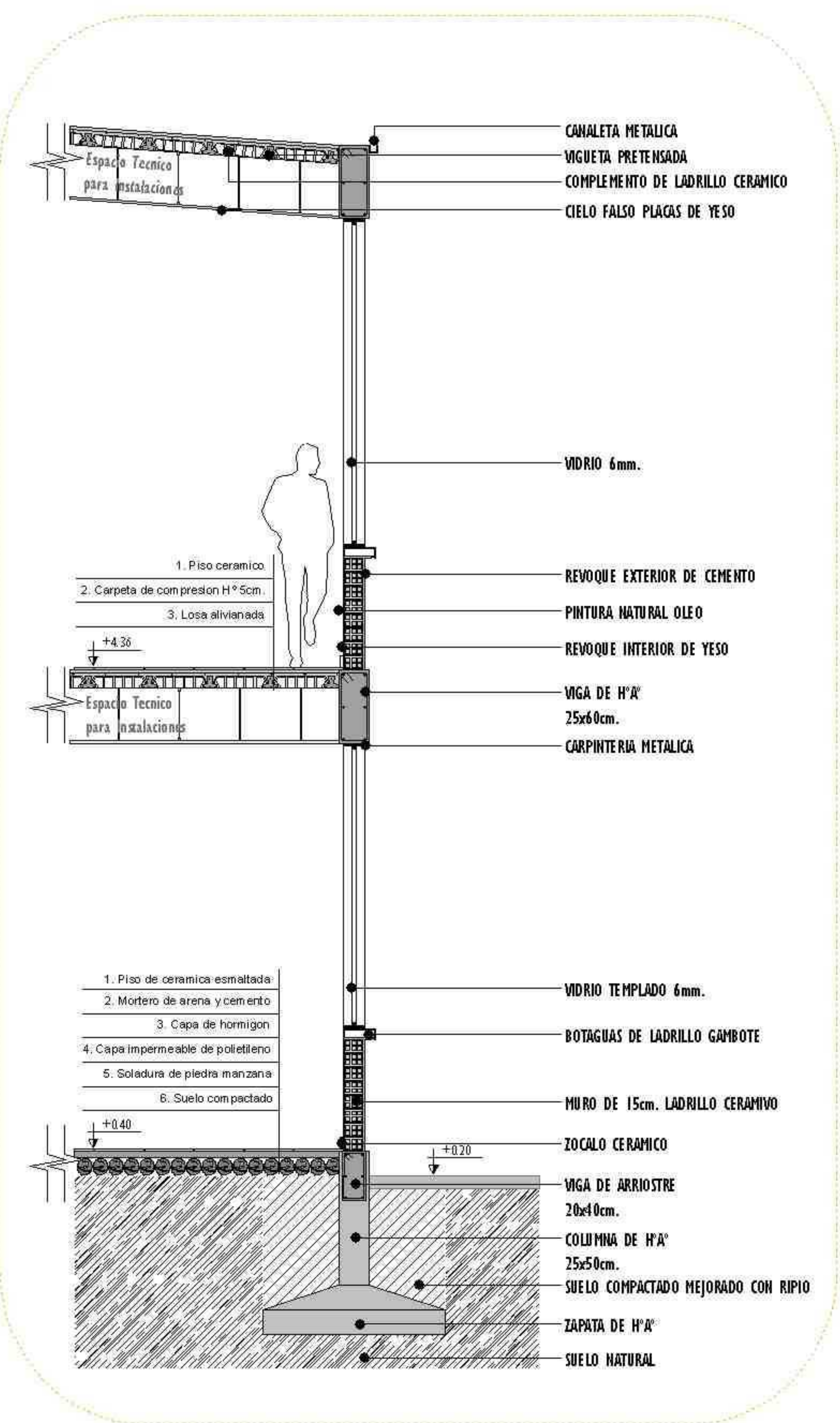
CORTE DE BORDE ESC. 1:25
