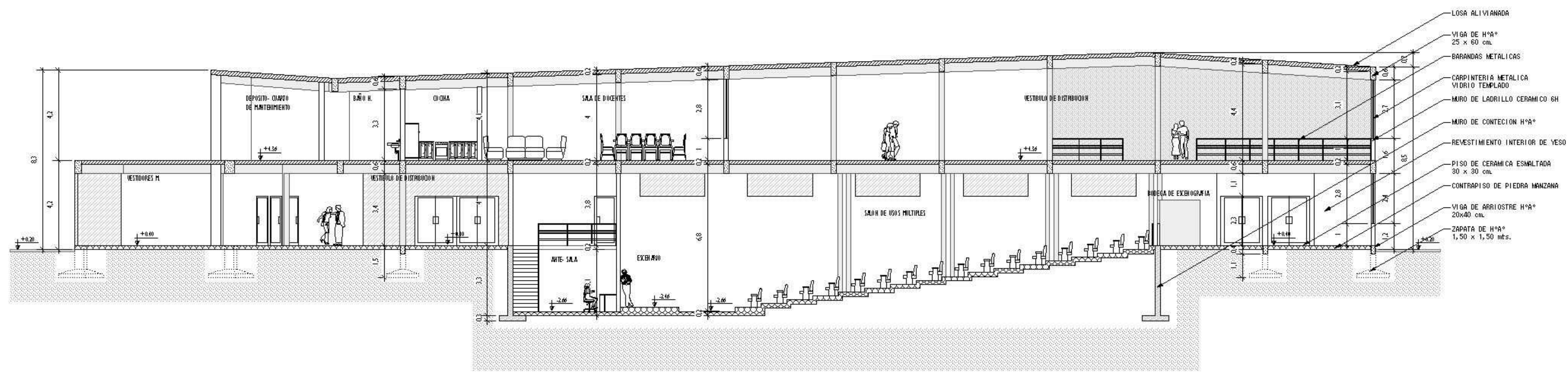
CORTE A-A
