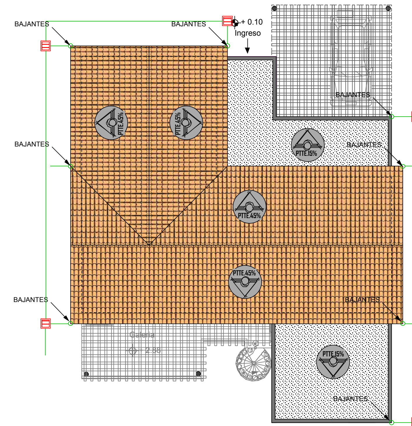
PLANO DE TECHOS VIVIENDA BIFAMILIAR Esc. 1:100
