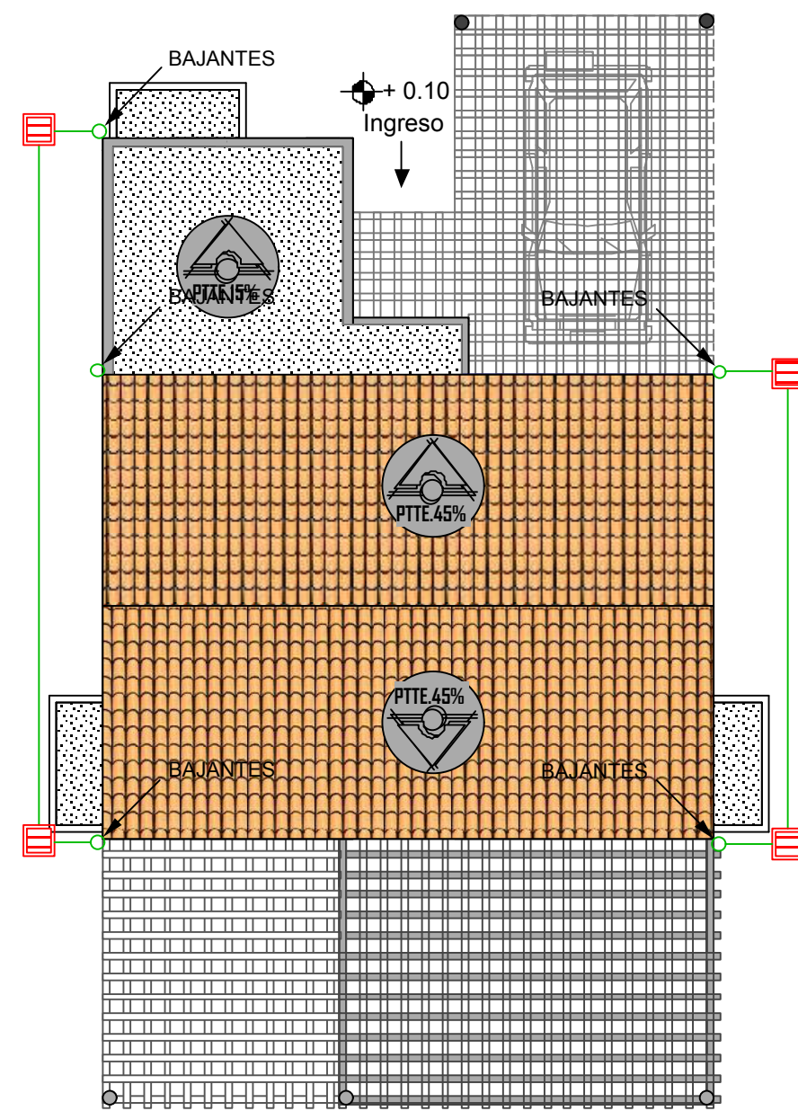
PLANO DE TECHOS VIVIENDA UNIFAMILIAR Esc. 1:100
