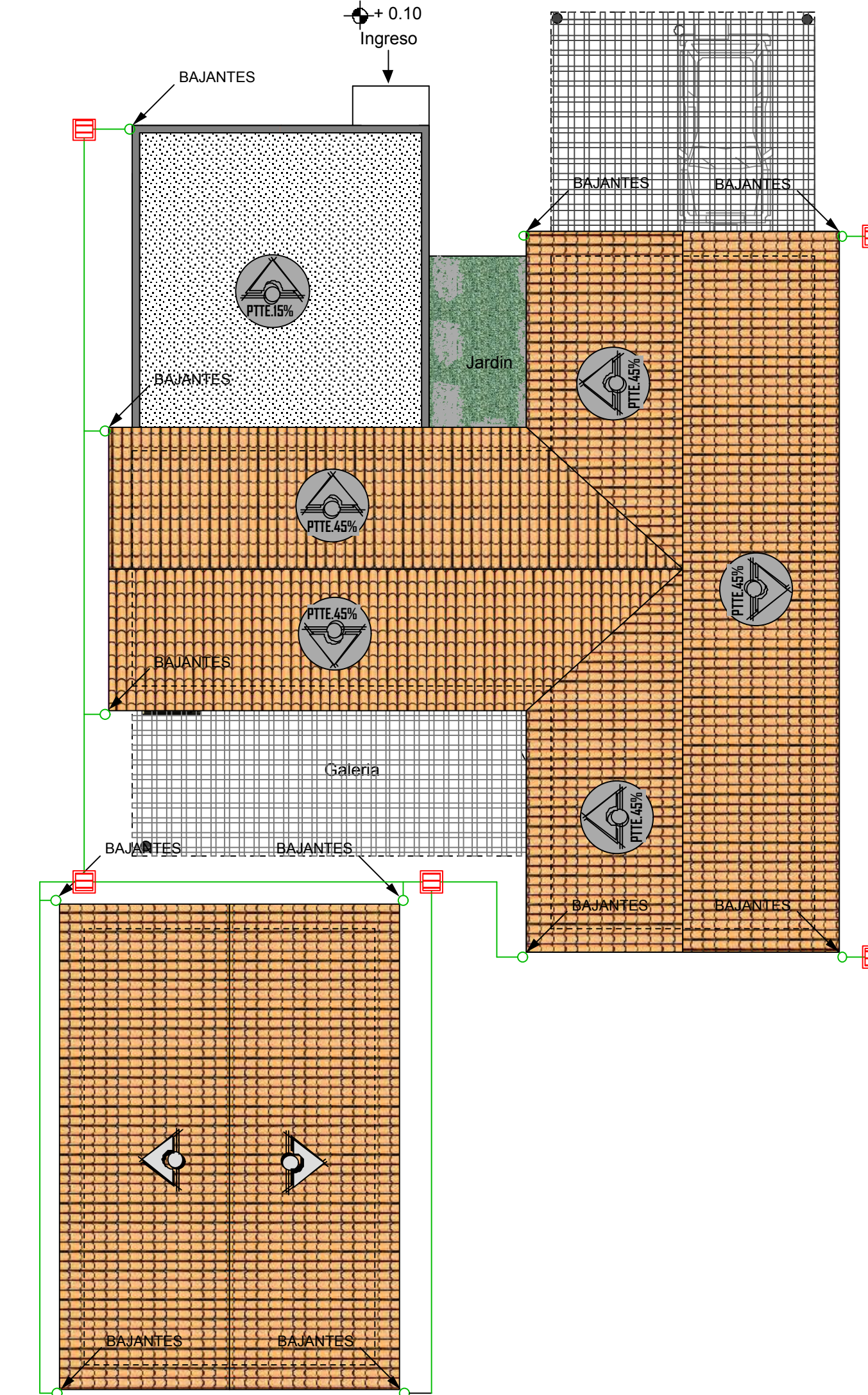
PLANO DE TECHOS VIVIENDA PRODUCTIVA Esc. 1:100
