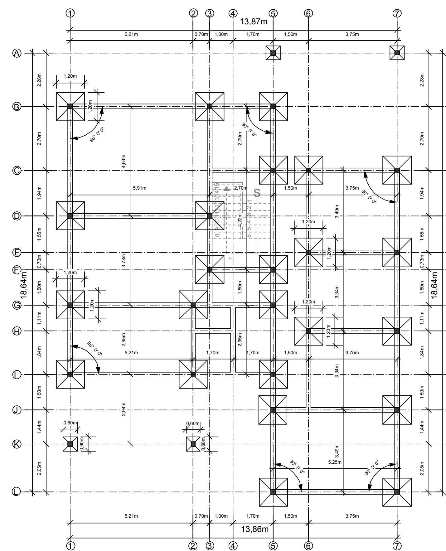
PLANO DE VIGAS Y ARRIOSTRE PLANTA BIFAMILIAR Esc. 1:100
