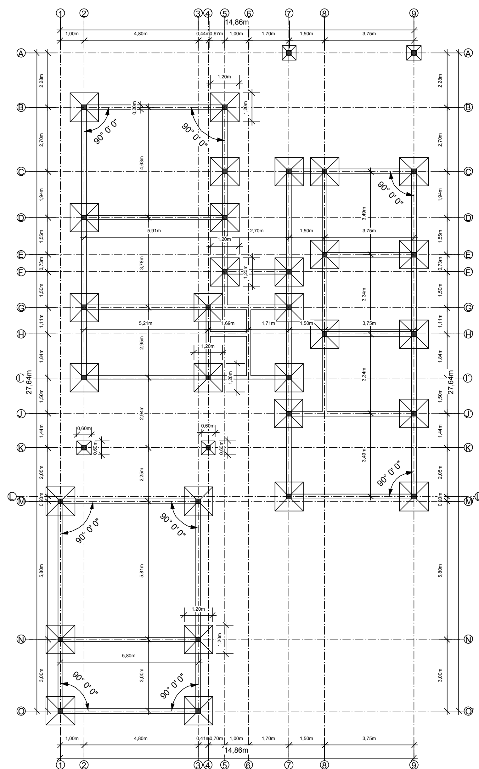
PLANO DE VIGAS Y ARRIOSTRE PLANTA PRODUCTIVA Esc. 1:100
