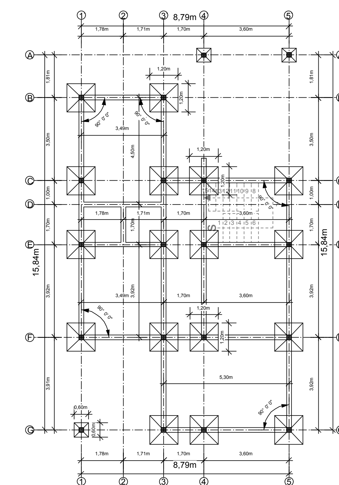
PLANO DE VIGAS Y ARRIOSTRE PLANTA UNIFAMILIAR Esc. 1:100
