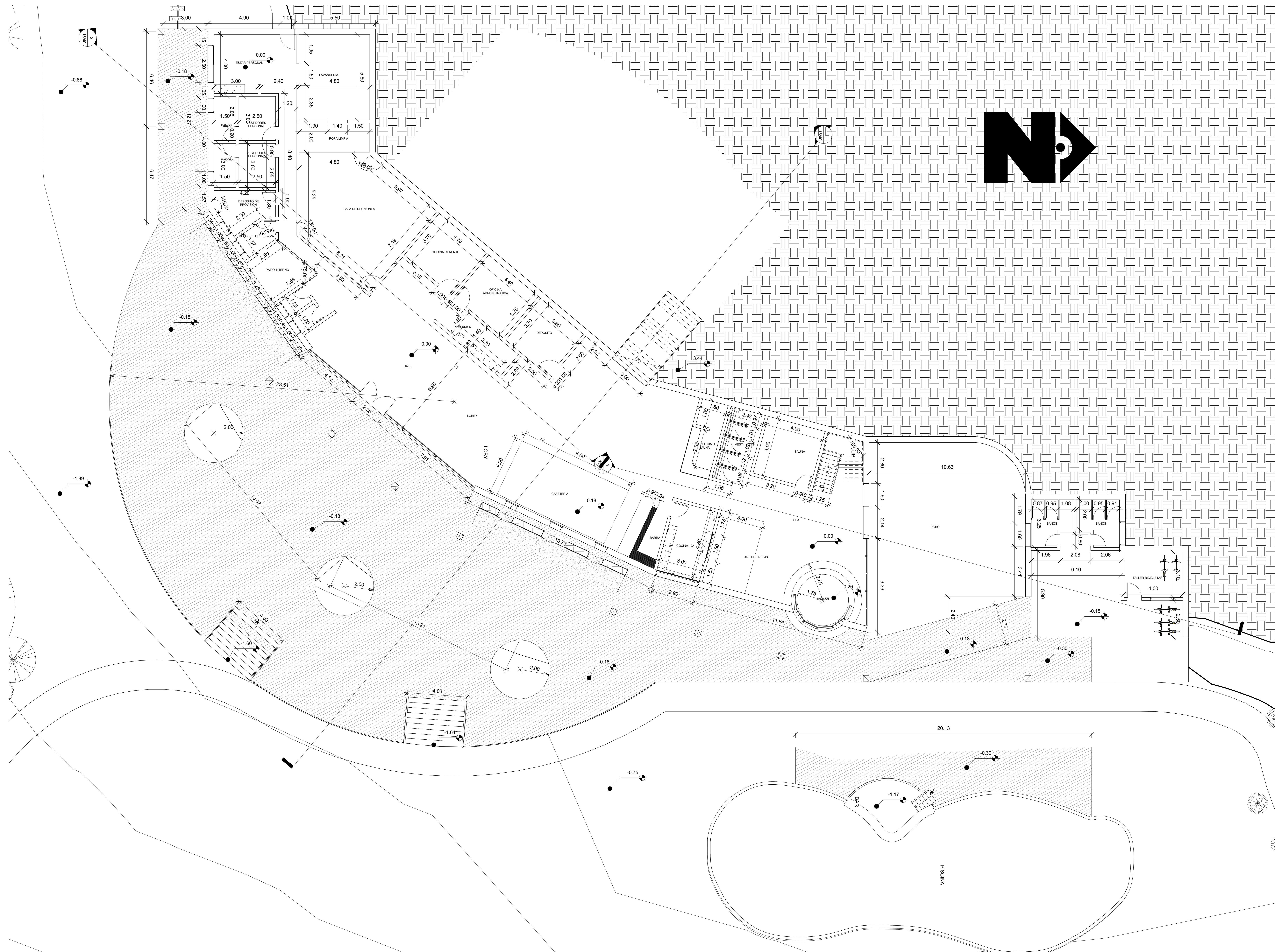
PLANTA BAJA ACOTADA
