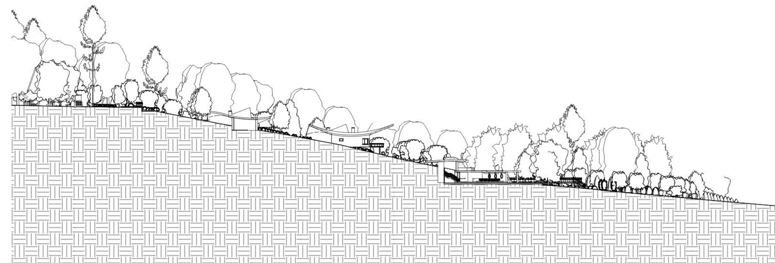
CORTE LONGITUDINAL NORESTE
