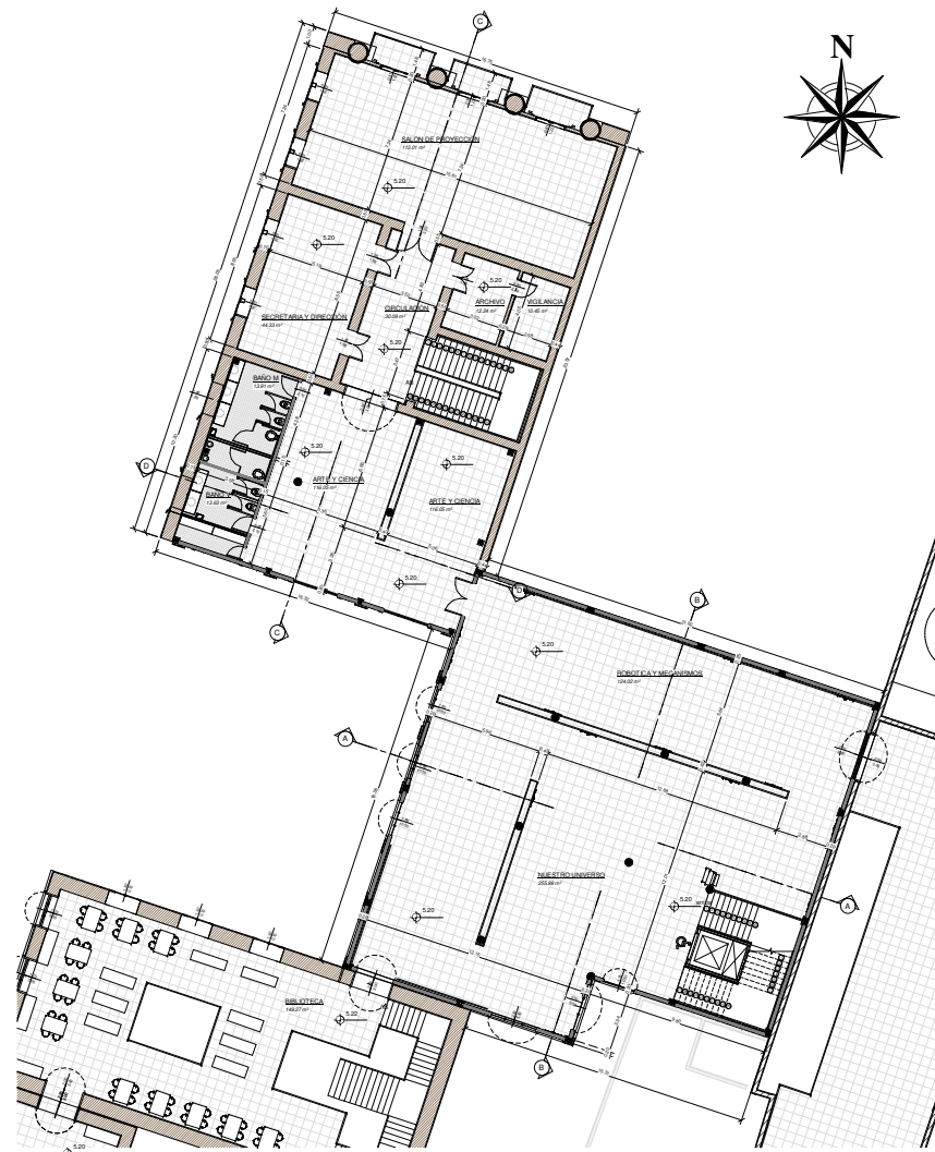
PRIMERA PLANTA ACOTADA ESC. 1:100
