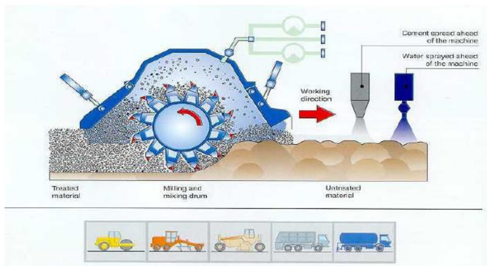
Figura 20 Mezclado – escarificado, aplicando agua y cemento simultáneamente
