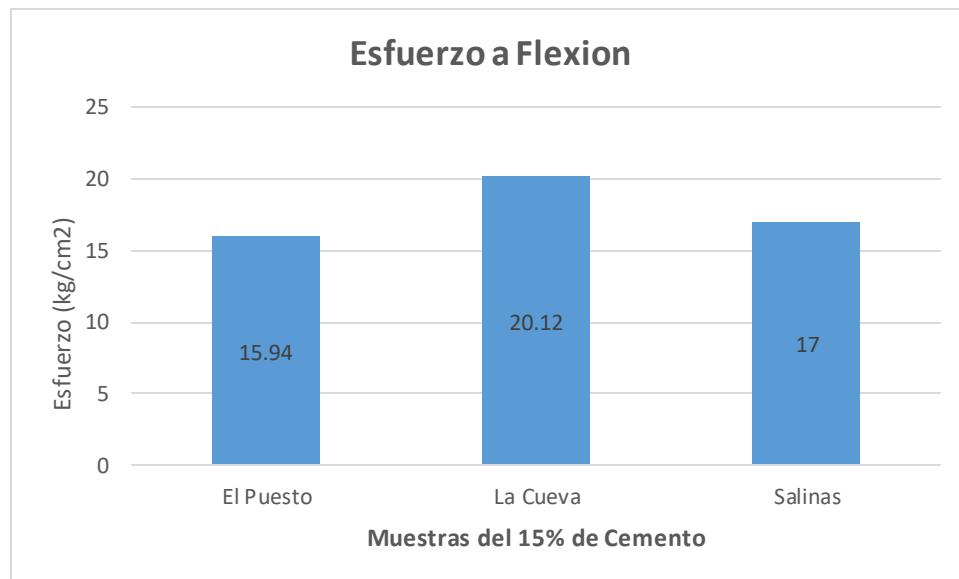
Gráfica 17 Resultados promedios de esfuerzos a flexión
