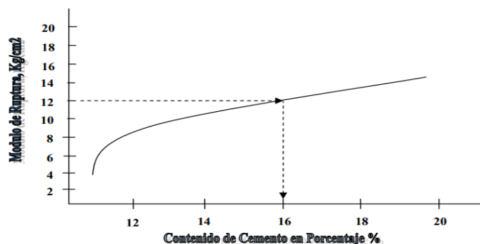
Figura 12 Módulo de Ruptura vs. Porcentaje de Cemento
