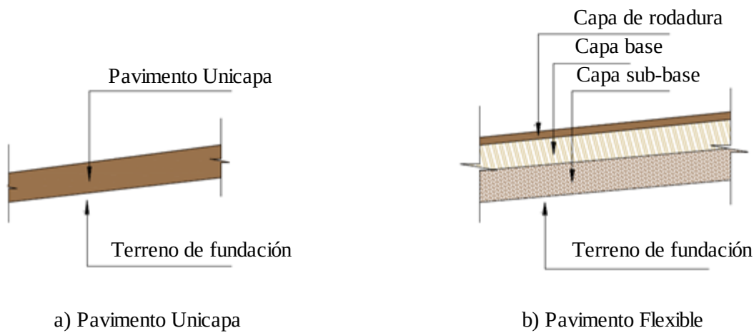
Figura 7 Tipos de pavimento
