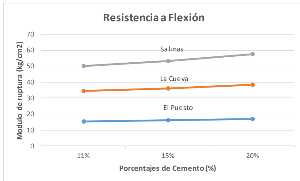
Gráfica 25 Resistencia versus porcentaje de cemento
