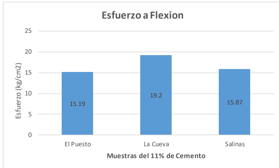
Gráfica 16 Resultados promedios de esfuerzos a flexión
