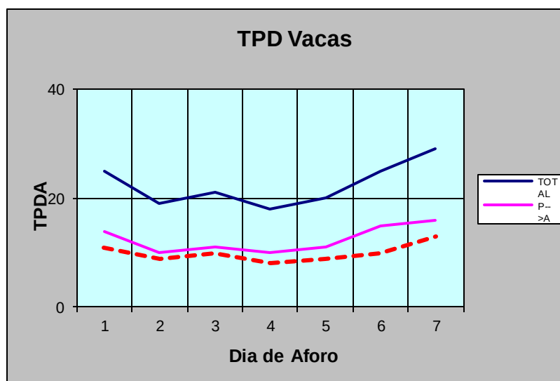
Gráfica 26 TPD Promedio
