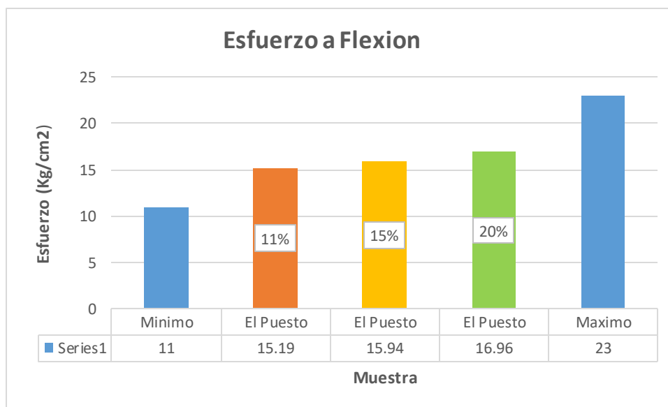
Gráfica 19 Esfuerzo de flexión El Puesto
