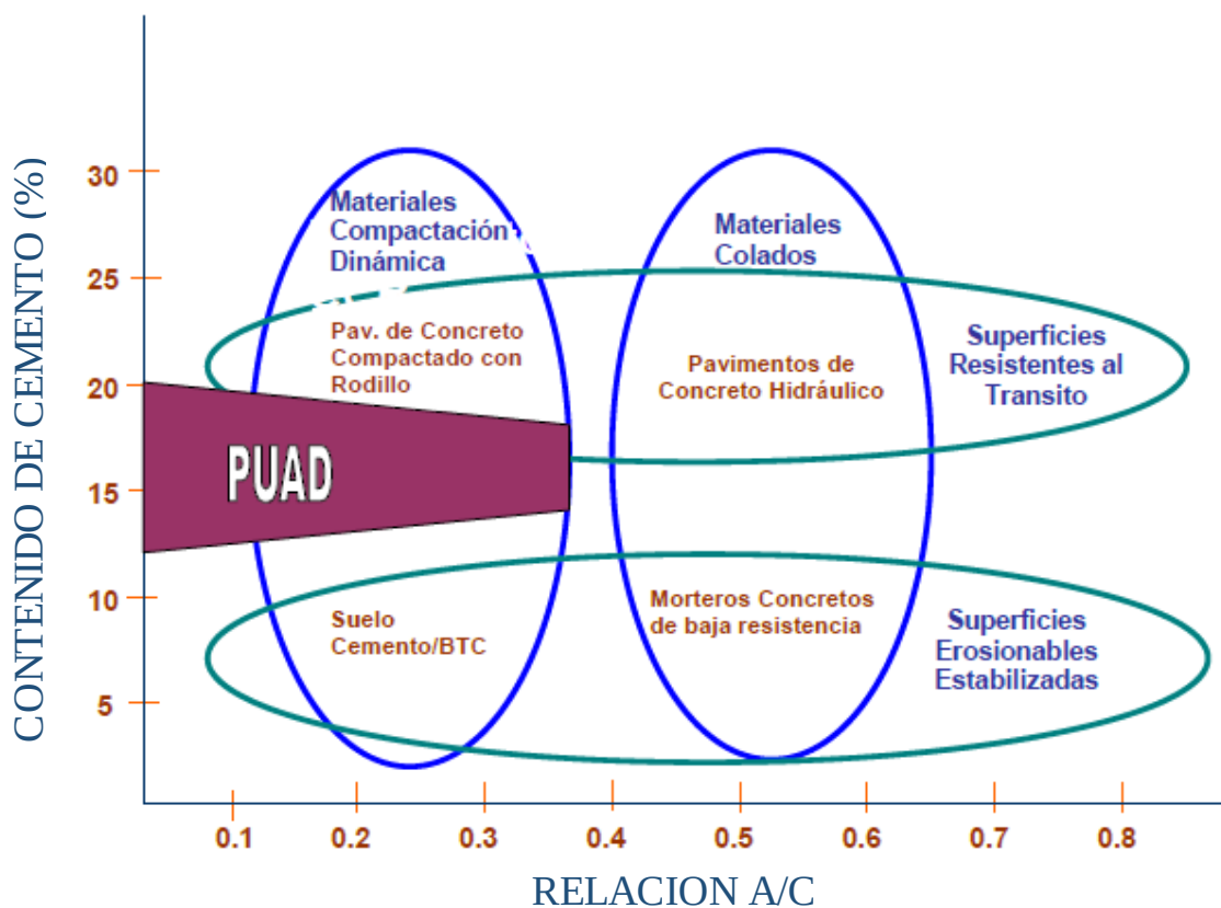
Figura 8 Ubicación de los PU en el conjunto de estructuras de pavimentos disponibles
