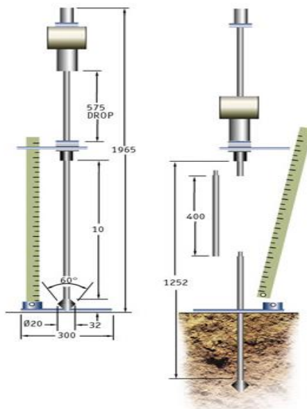
Figura 11 Penetrómetro dinámico de cono (DCP)
