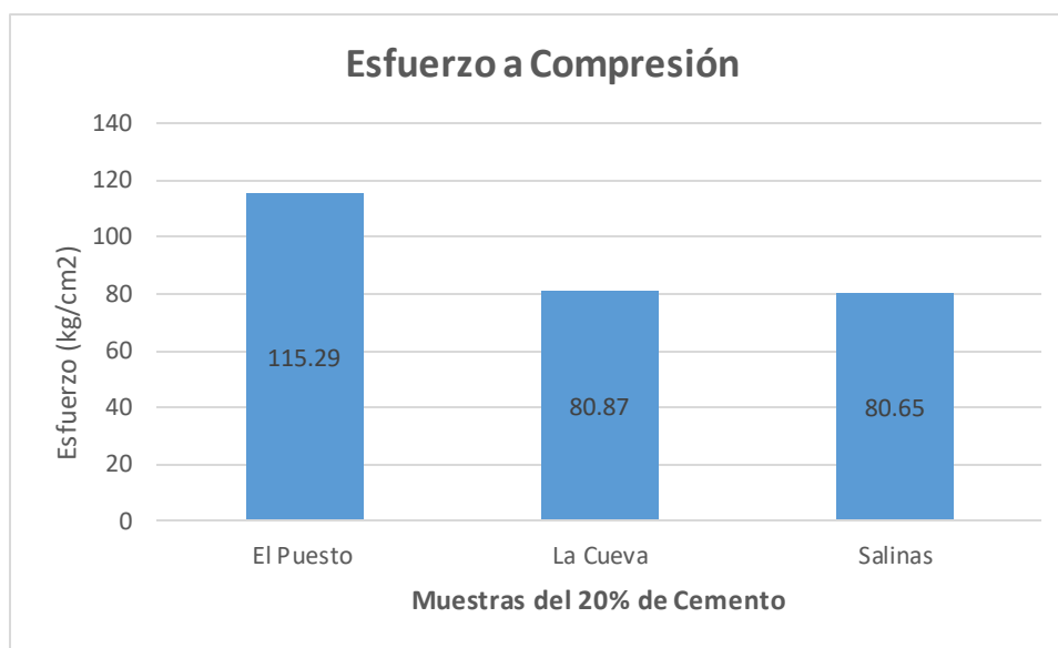
Gráfica 6 Resultados promedios de esfuerzos a compresión
