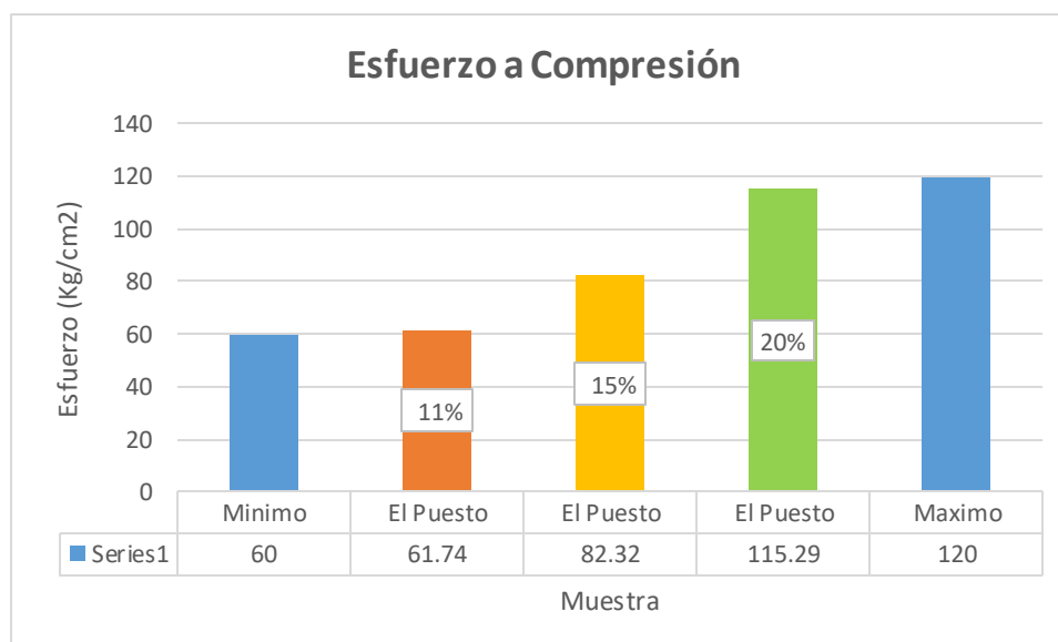
Gráfica 7 Esfuerzo de compresión El Puesto
