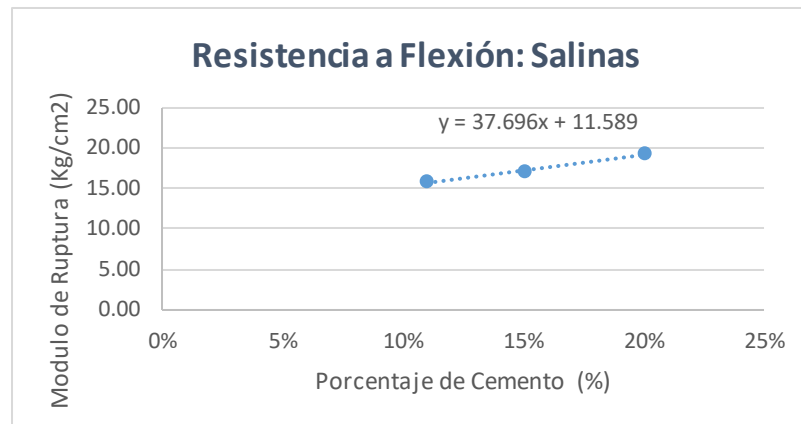
Gráfica 24 Resistencia versus porcentaje de cemento
