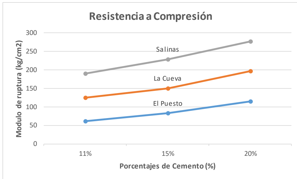
Gráfica 13 Resistencia versus porcentaje de cemento
