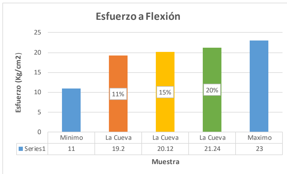
Gráfica 20 Esfuerzo de flexión La Cueva
