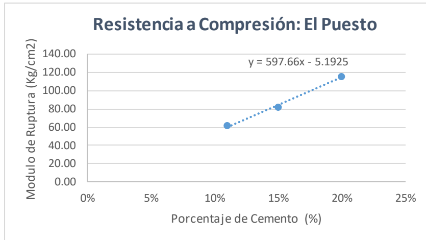
Gráfica 10 Resistencia versus porcentaje de cemento
