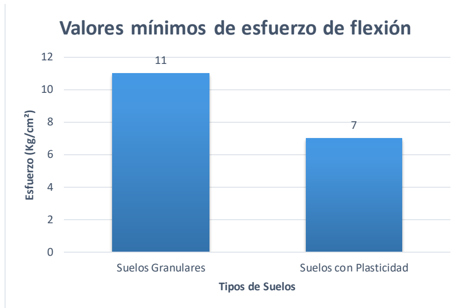
Gráfica 14 Valores mínimos de esfuerzo de flexión
