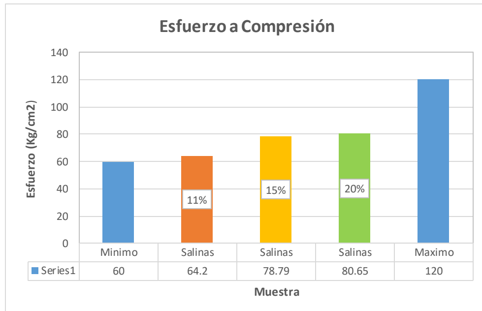
Gráfica 9 Esfuerzo de compresión de Salinas
