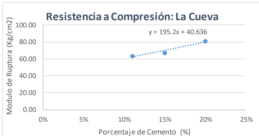
Gráfica 11 Resistencia versus porcentaje de cemento
