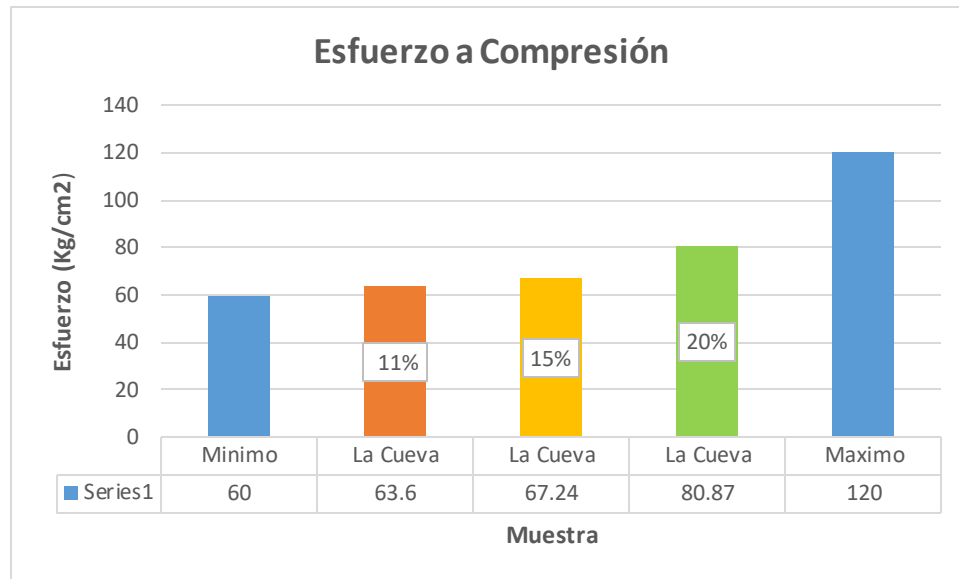
Gráfica 8 Esfuerzo de compresión La Cueva
