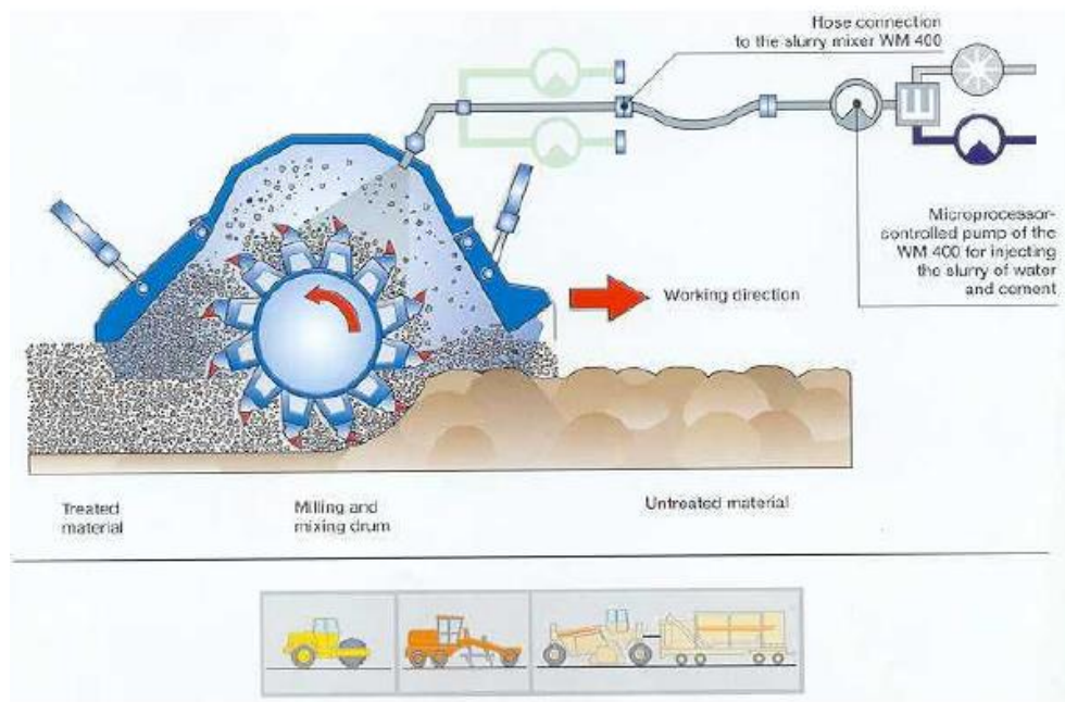
Figura 22 Procesos de forma simultánea
