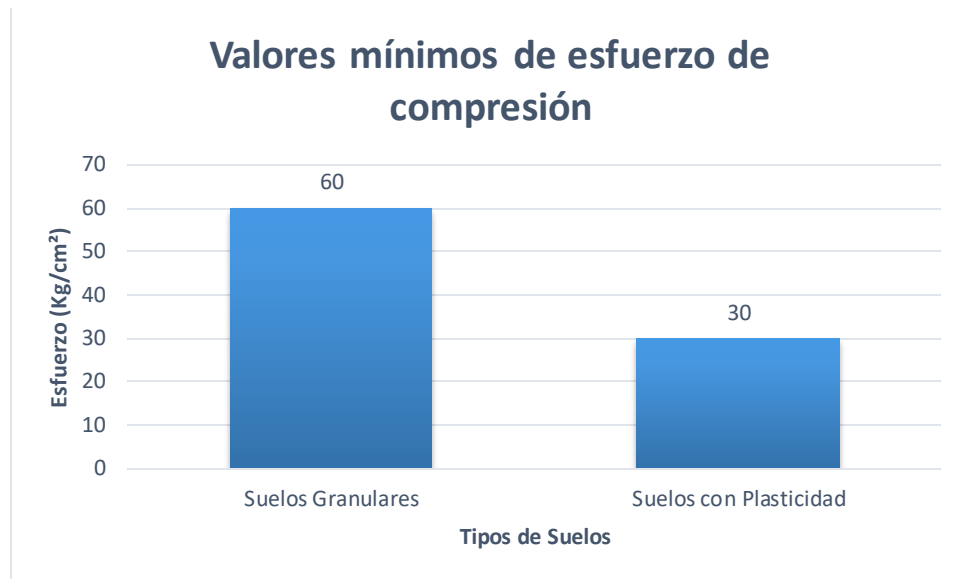
Gráfica 2 Valores mínimos de esfuerzos de compresión
