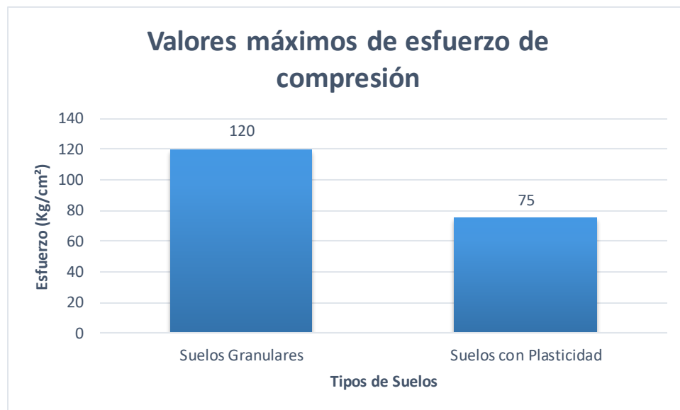
Gráfica 3 Valores máximos de esfuerzo de compresión
