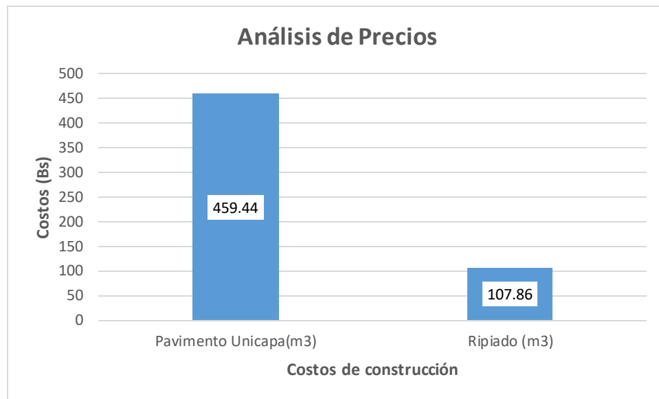
Gráfica 40 Análisis de precios
