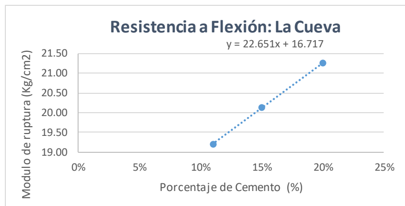
Gráfica 23 Resistencia versus porcentaje de cemento
