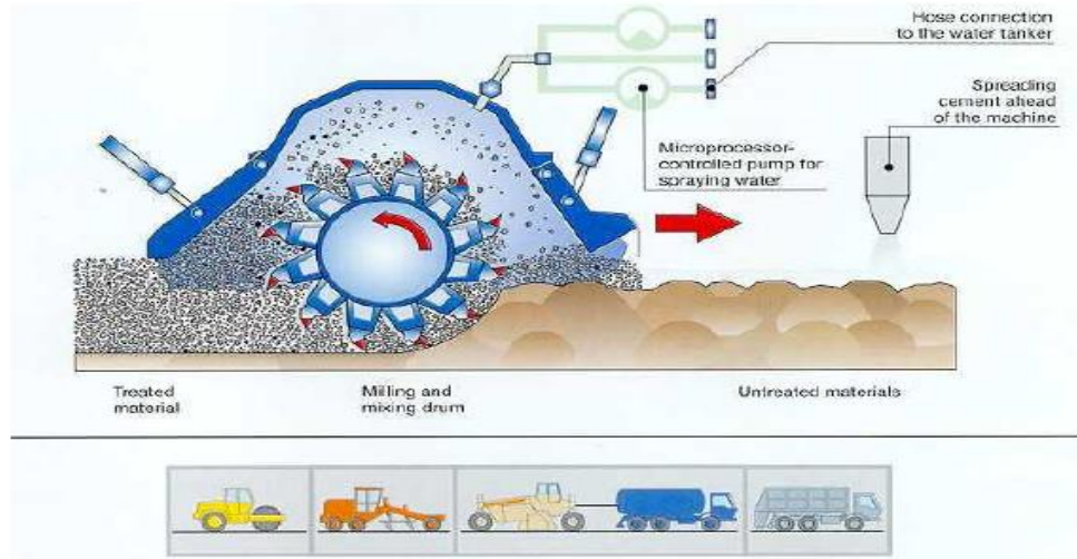
Figura 21 Aplicando el cemento y posteriormente escarificando
