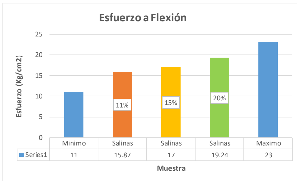
Gráfica 21 Esfuerzo de flexión de Salinas
