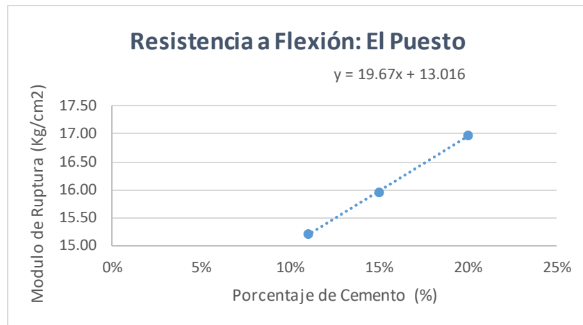
Gráfica 22 Resistencia versus porcentaje de cemento
