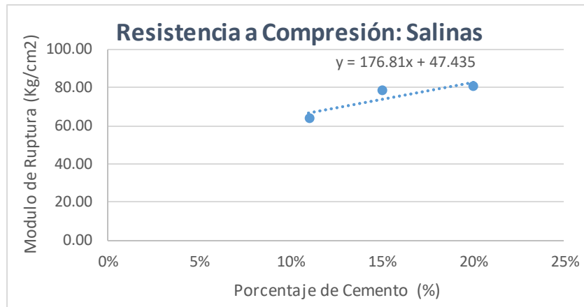
Gráfica 12 Resistencia versus porcentaje de cemento
