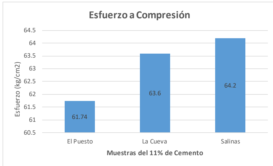
Gráfica 4 Resultados promedios de esfuerzos a compresión
