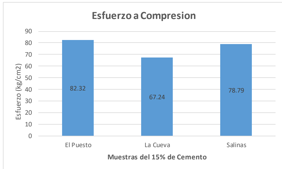
Gráfica 5 Resultados promedios de esfuerzos a compresión
