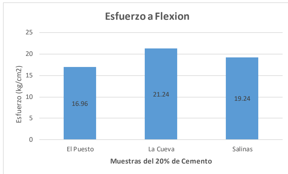
Gráfica 18 Resultados promedios de esfuerzos a flexión
