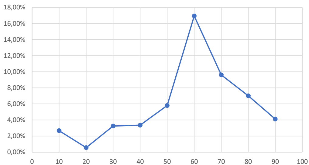
Demora relativa (Veh/hr) Vs Enlace rotonda Aeropuerto (m)
