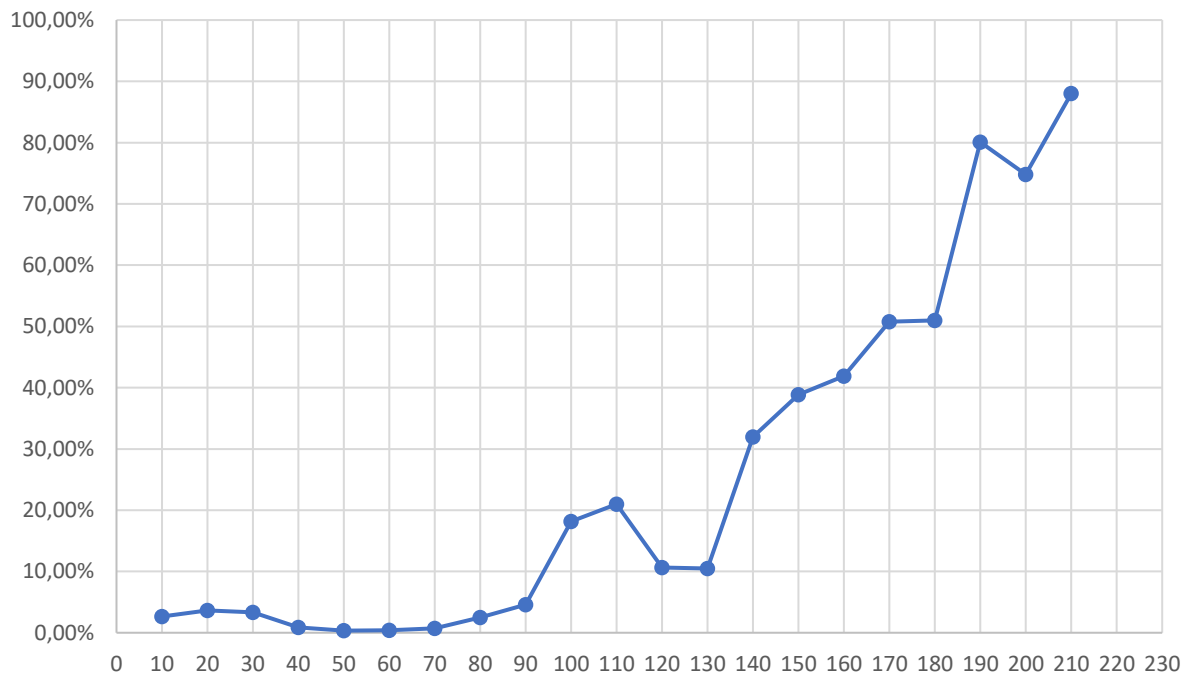
Demora relativa (Veh/hr) Vs Enlace rotonda Puente San Martin (m)
