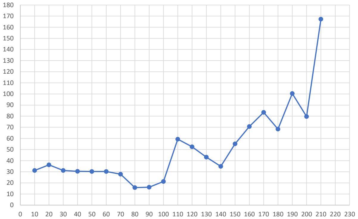
Densidad Vehicular (Veh/hr) Vs Enlace rotonda Puente San Martin(m)
