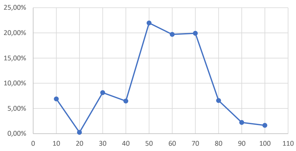
Demora relativa (Veh/hr) Vs Enlace rotonda UAJMS (m)
