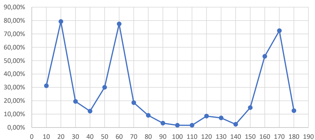
Demora relativa (Veh/hr) Vs Enlace rotonda fuente de los deseos (m)
