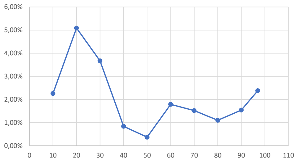
Demora relativa (Veh/hr) Vs Enlace rotonda Tabladita (m)
