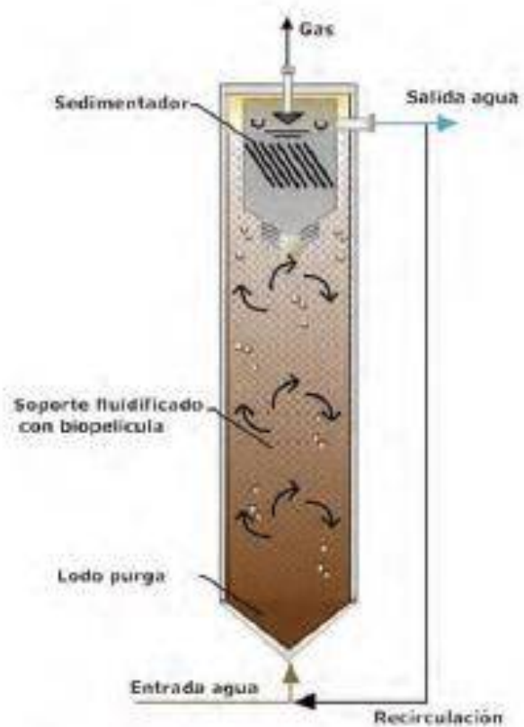
Reactor anaerobio de lecho fluidificado (100% expandido)
