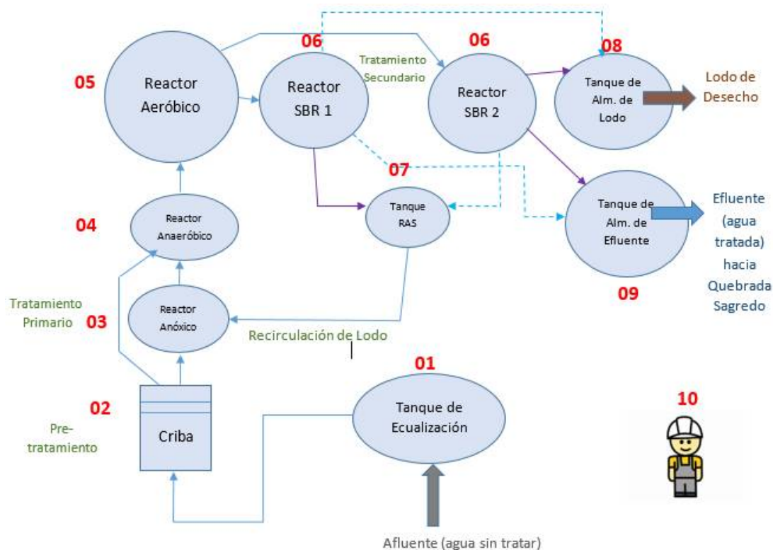
Figura 2. 17. Flujo de Proceso de PTAR – Barrio Catedral
