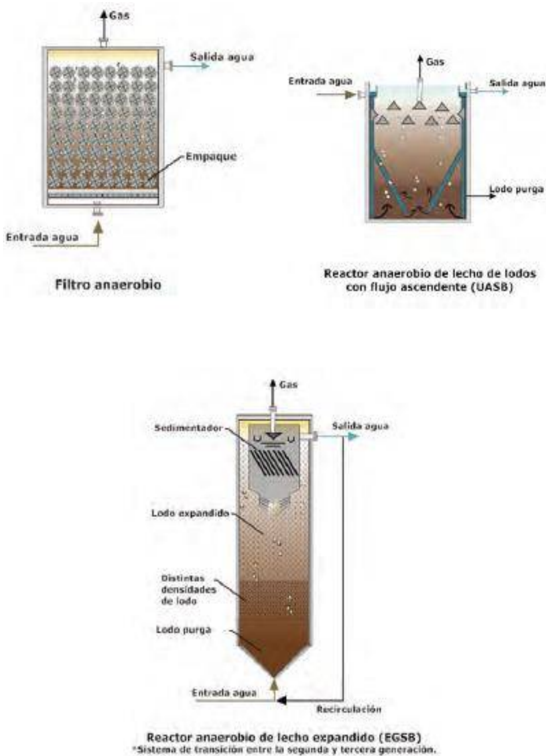
Figura 2. 10. Procesos anaerobios para el tratamiento de aguas residuales segunda generación
