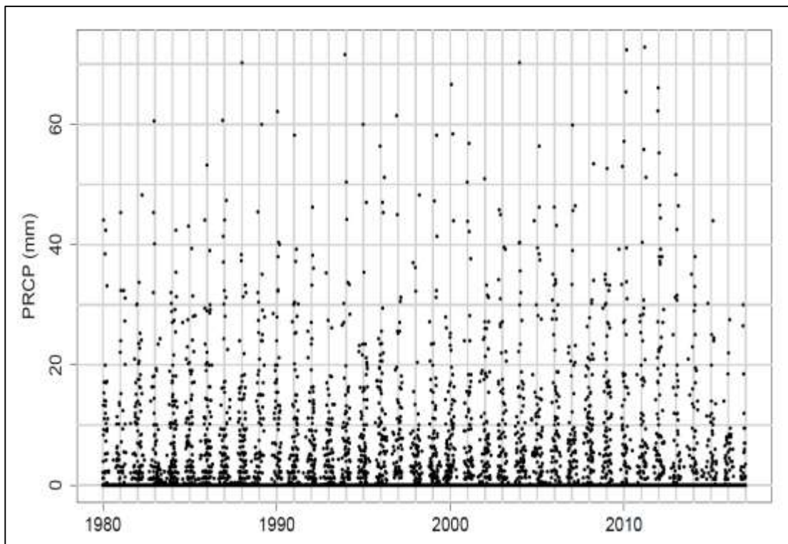
Anexo 1.18 Estación Chocloca Precipitaciones diarias
