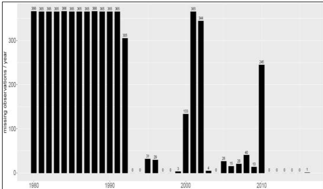
Anexo 1.17 Estación Ce.Na.Vit. Histograma de datos faltantes de temperaturas mínimas diarias
