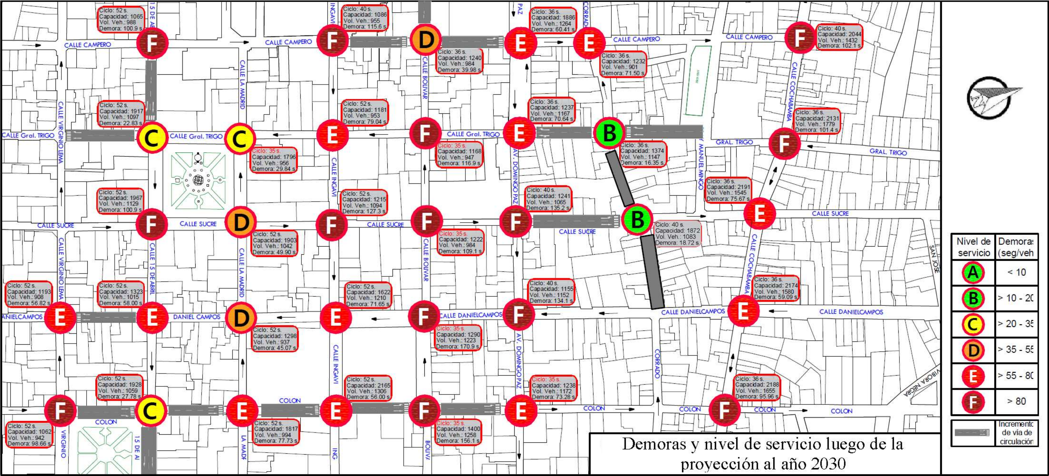
Plano 4: Demoras y nivel de servicio luego de la proyección al año 2030
