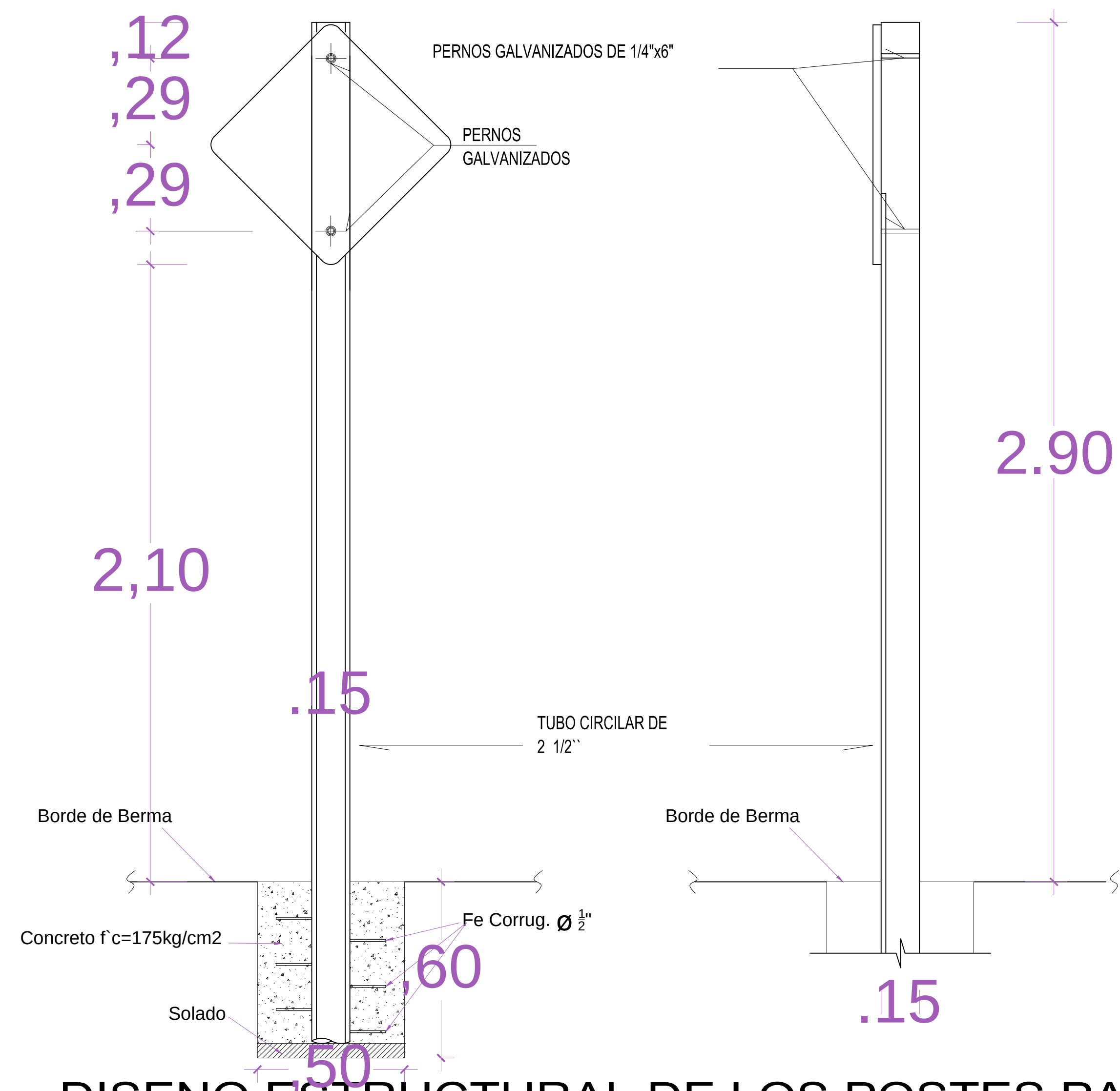
DISEÑO ESTRUCTURAL DE LOS POSTES PARA SEÑALIZACION PREVENTIVA Y REGLAMENTARIA
