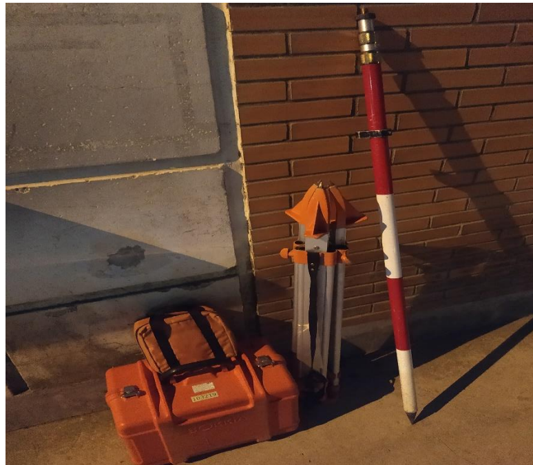
Estacion, trípode y prisma
