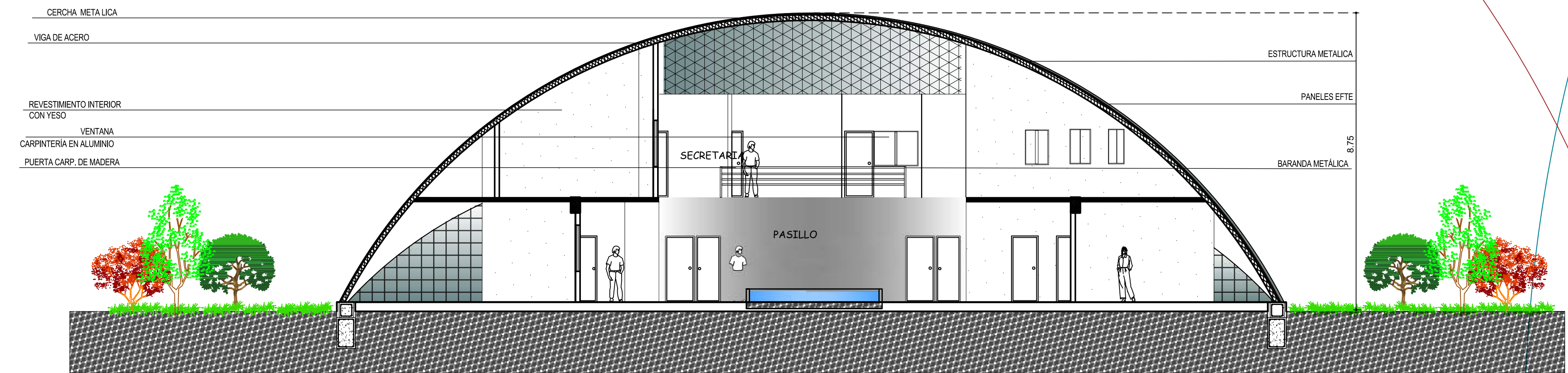
CORTE ADMINISTRACIÓN B-B' ESC: 1:100
