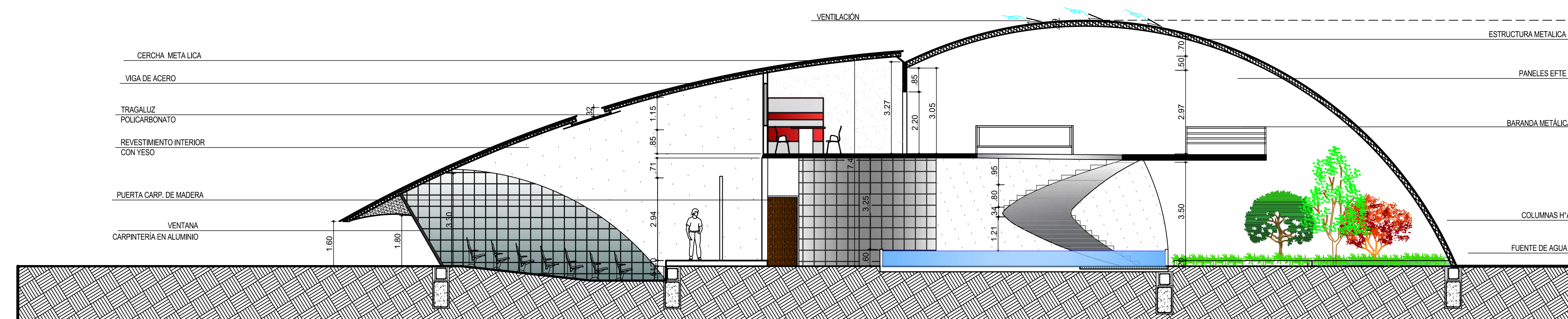
CORTE ADMINISTRACIÓN A-A' ESC: 1:100
