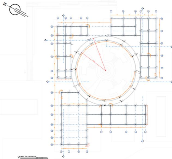
V. PLANO DE CIMENTOS
